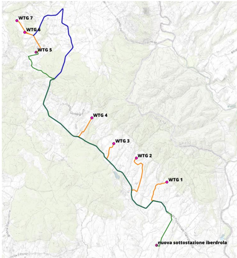
Figure 18 – Inquadramento progetto nella carta Topografica Standard con indicazione della viabilità di trasporto parzialmente esistente (percorso blu), della viabilità per le piazzole degli aerogeneratori (percorso arancione) e del tracciato del cavidotto (percorso verde).
