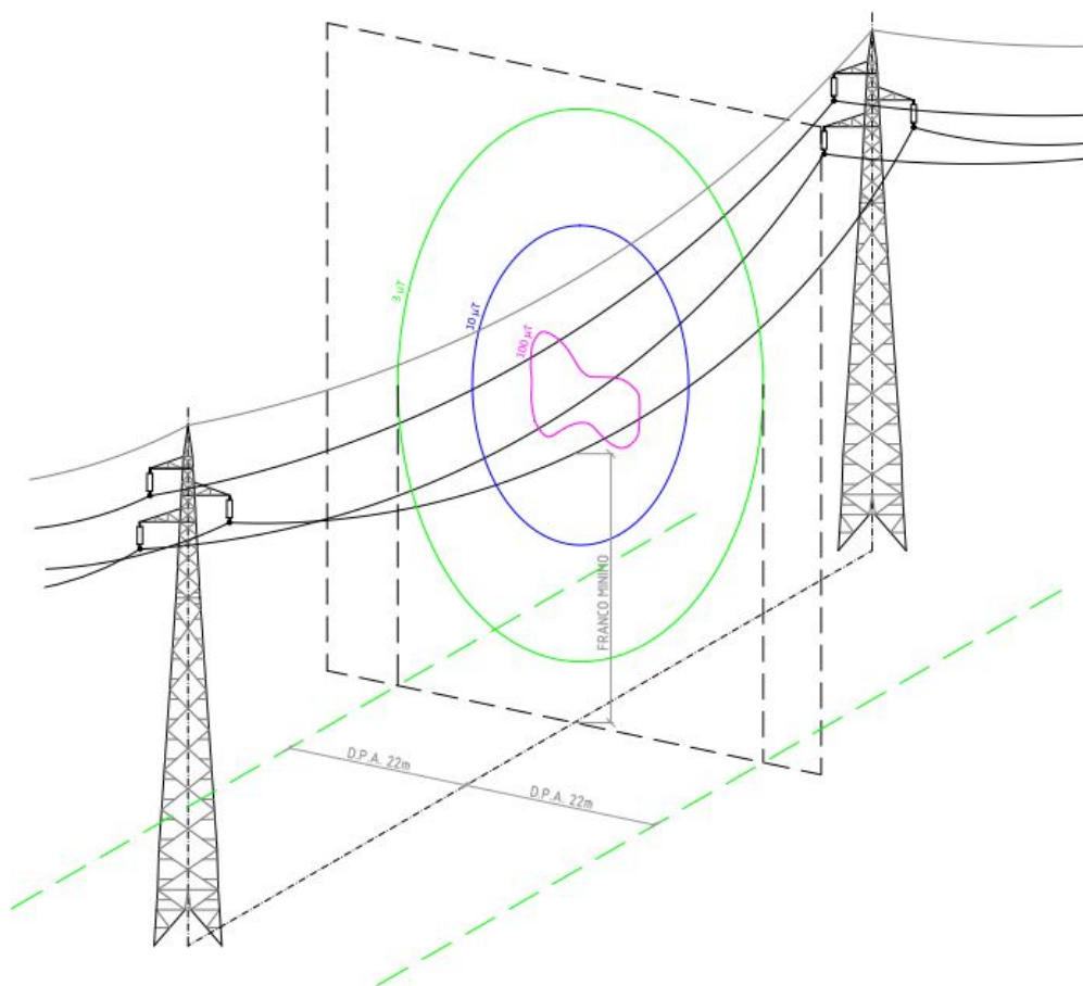
Figura 3 - Schematizzazione isolinee B: 100 \mu T, 10 \mu T e 3 \mu T, in corrispondenza del franco minimo
