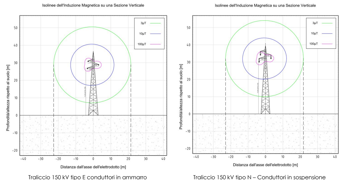
Figura 2 - Isolinee del campo magnetico B, valori: 100µT, 10µT e 3µT alla quota testa tralicci -
