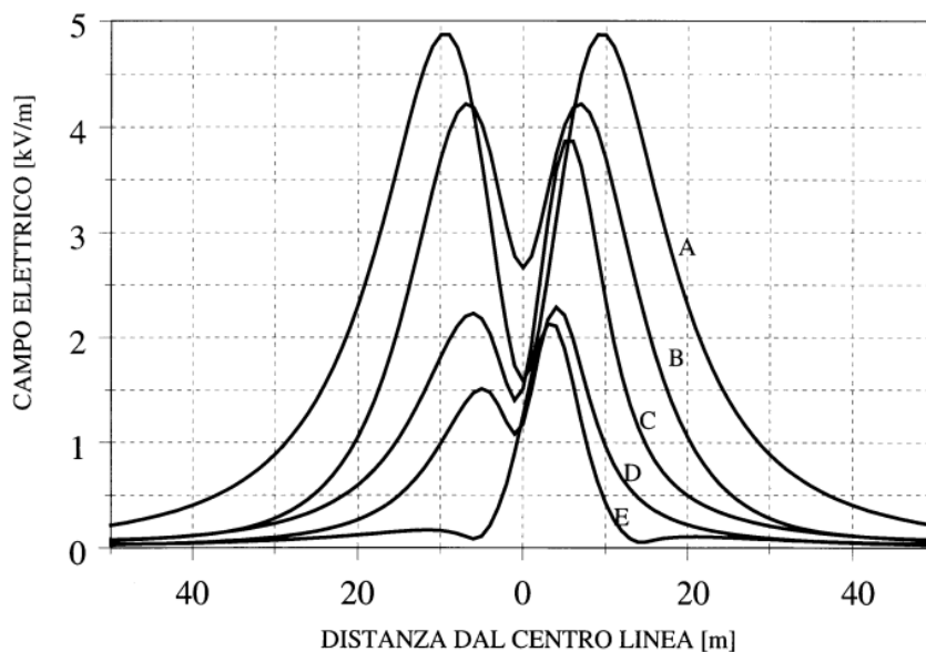
Figura 4 – Profili laterali del campo elettrico per i tralicci AT –
