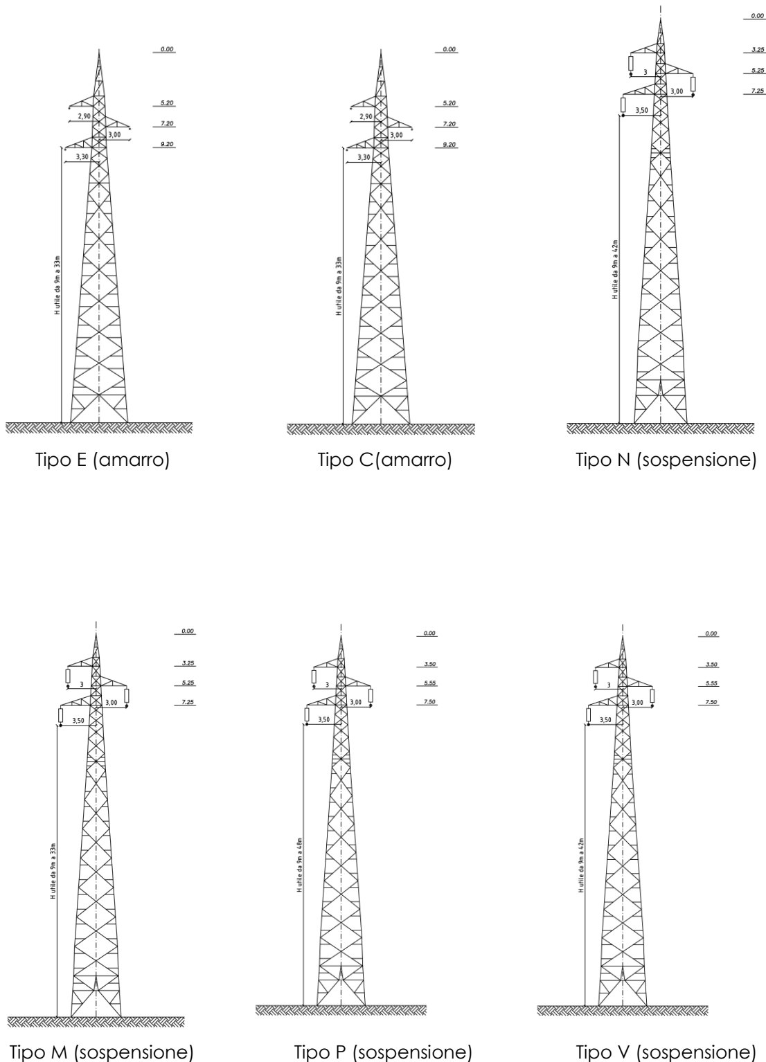
Figura 1 - Pali unificati 150 kV – Semplice terna – in amarro ed a sospensione
