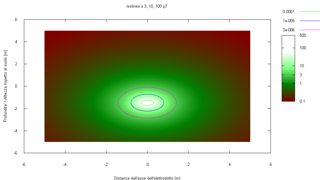
Figura 7 – Isolinee 3, 10 e 100 µT per una doppia terna interrata.
