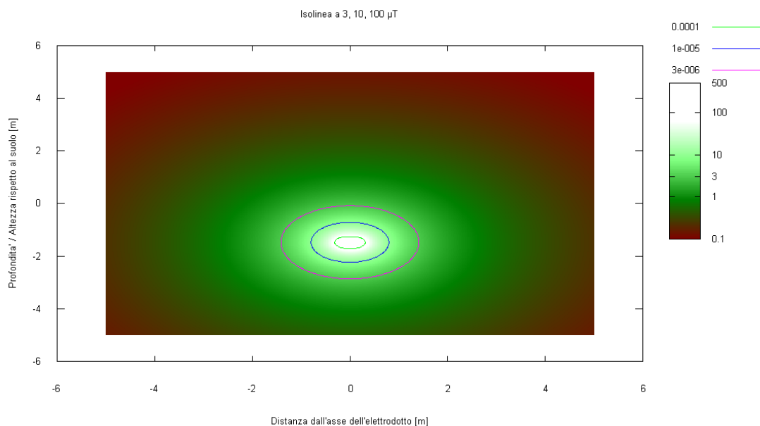
Figura 7 – Isolinee 3, 10 e 100 μT per una doppia terna interrata.
