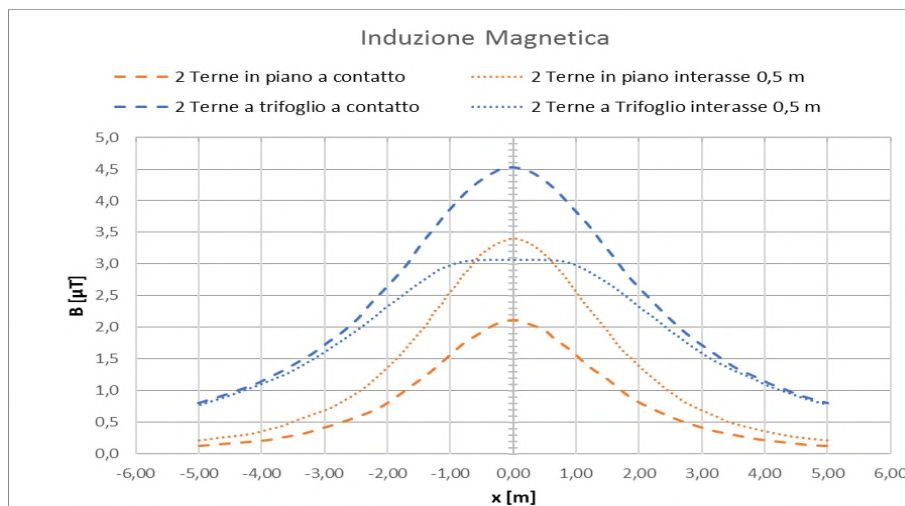
Figura 6 – Confronto induzione magnetica a 1 metro da terra di due terne (RST-TRS) posate: a trifoglio e in piano, I = 1000 A, diametro cavi 100 millimetri (rif. norma CEI 106-11)
