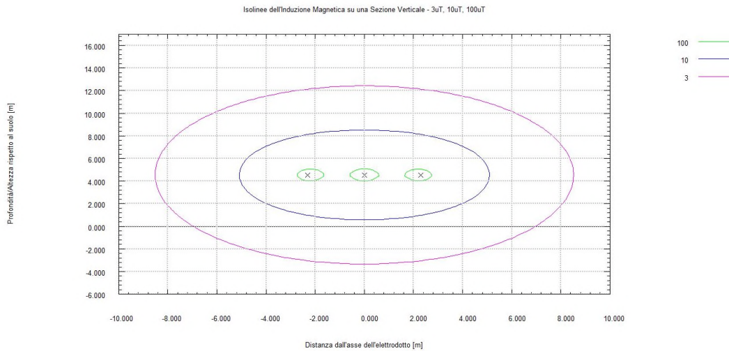
Figura 3 - Sbarre AT in aria - Isolinee induzione magnetica 3, 10 e 100 \mu\text{T}
