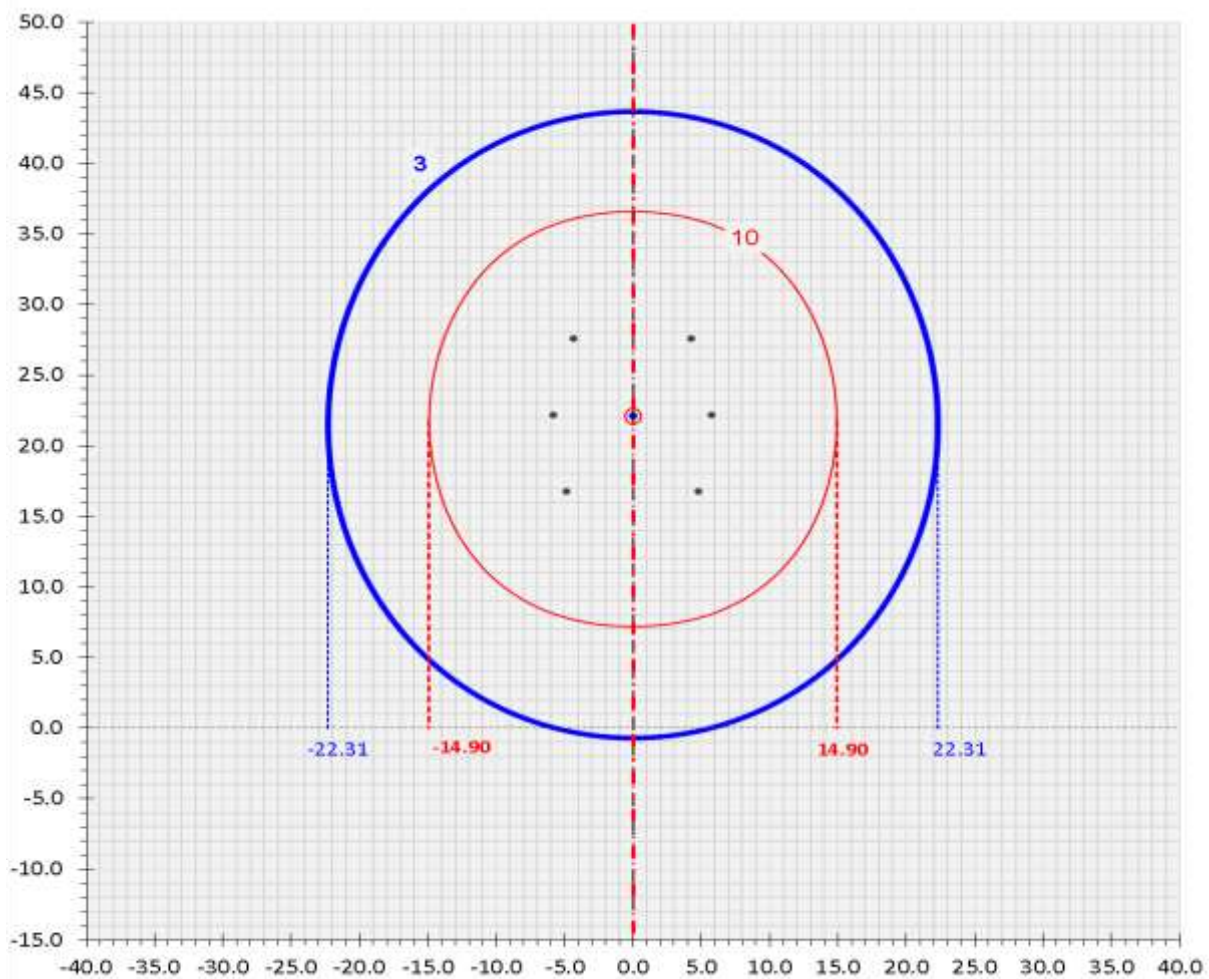
Isolinee dell'induzione magnetica nel caso di sostegno DT
