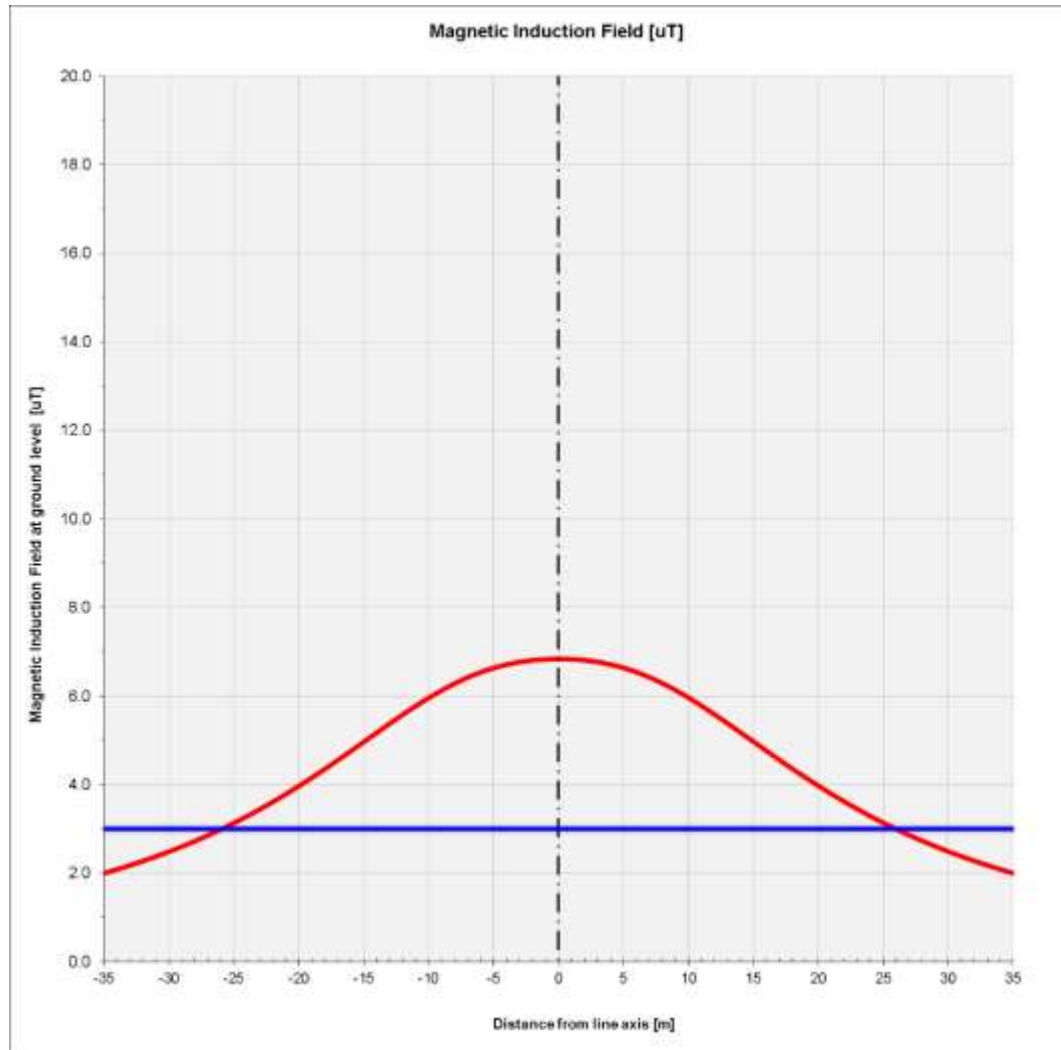
Fig. 1: andamento dell'induzione magnetica in una sezione perpendicolare all'asse linea, calcolata a 1,5 m dal suolo in caso di franco minimo (obiettivo di qualità pari a 3 \mu T)
