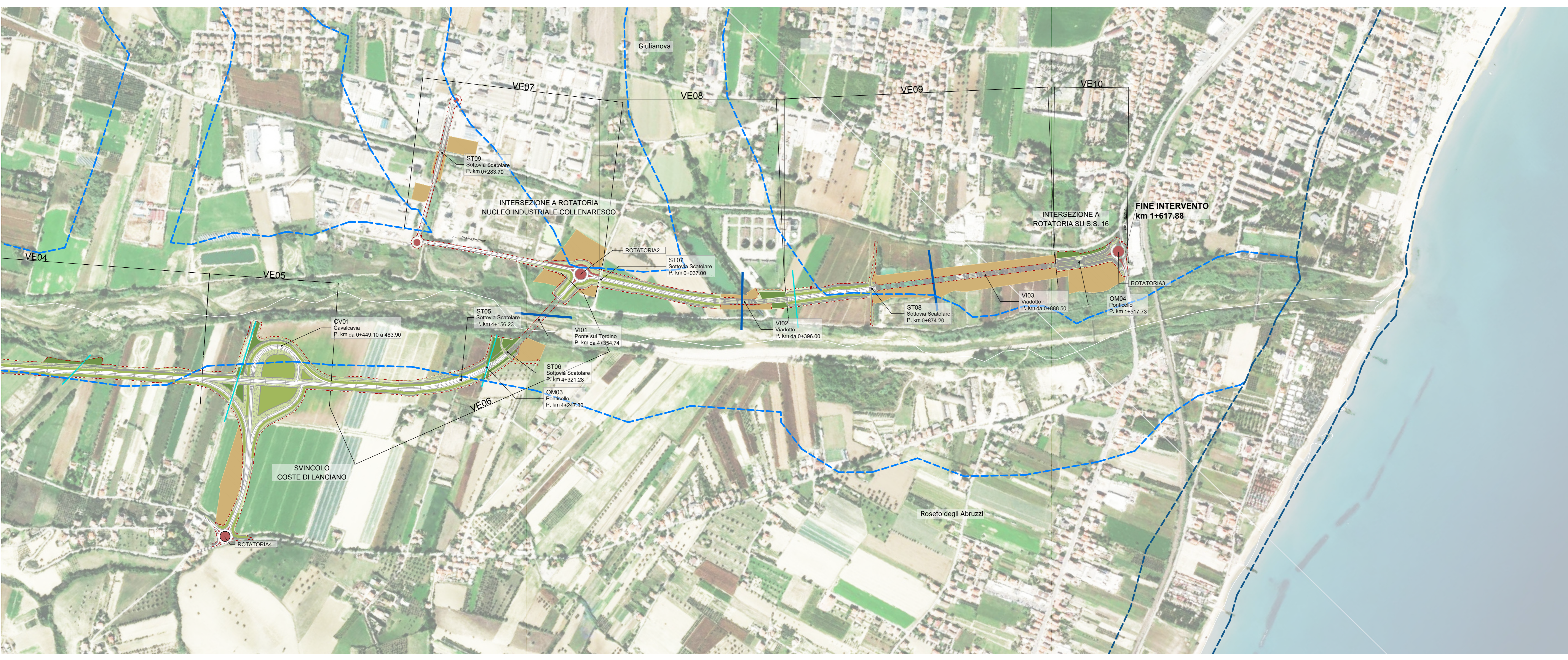
02 PLANIMETRIA GENERALE INTERVENTI DI INSERIMENTO PAESAGGISTICO E AMBIENTALE 1:5000
