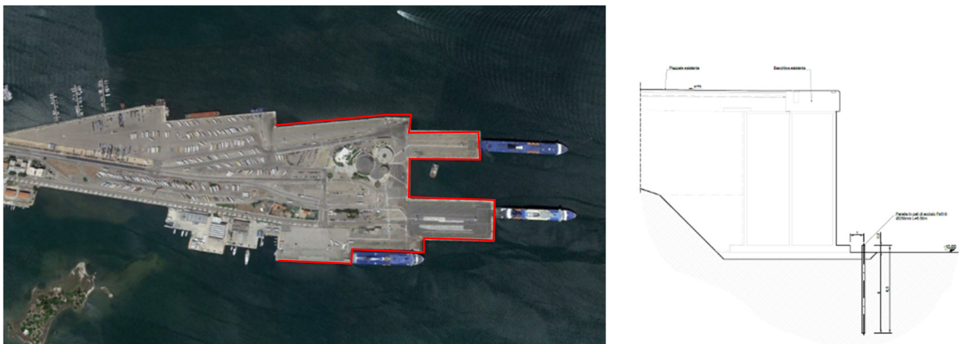
Figura 10. Planimetri e sezione paratia micropali
