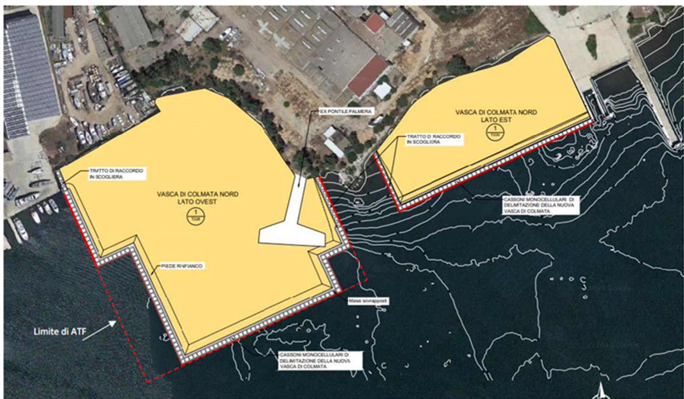
Figura 9. Ubicazione delle vasche di colmata zona colmata ex Palmiera
