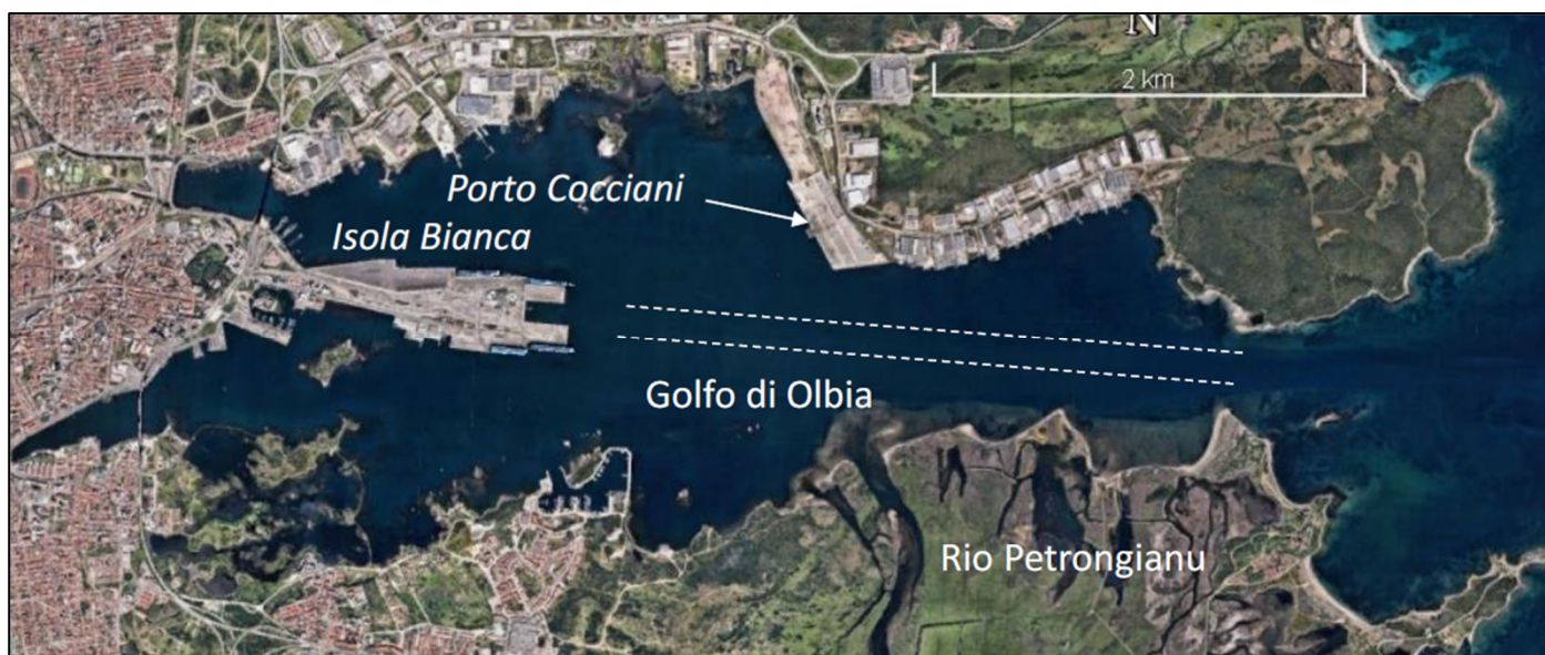
Figura 1. Inquadramento del Porto di Olbia con evidenza del porto commerciale (Isola bianca), del porto industriale (Porto Cocciani) e del canale di accesso, denominato Canaletta (rappresentato con linea tratteggiata)
