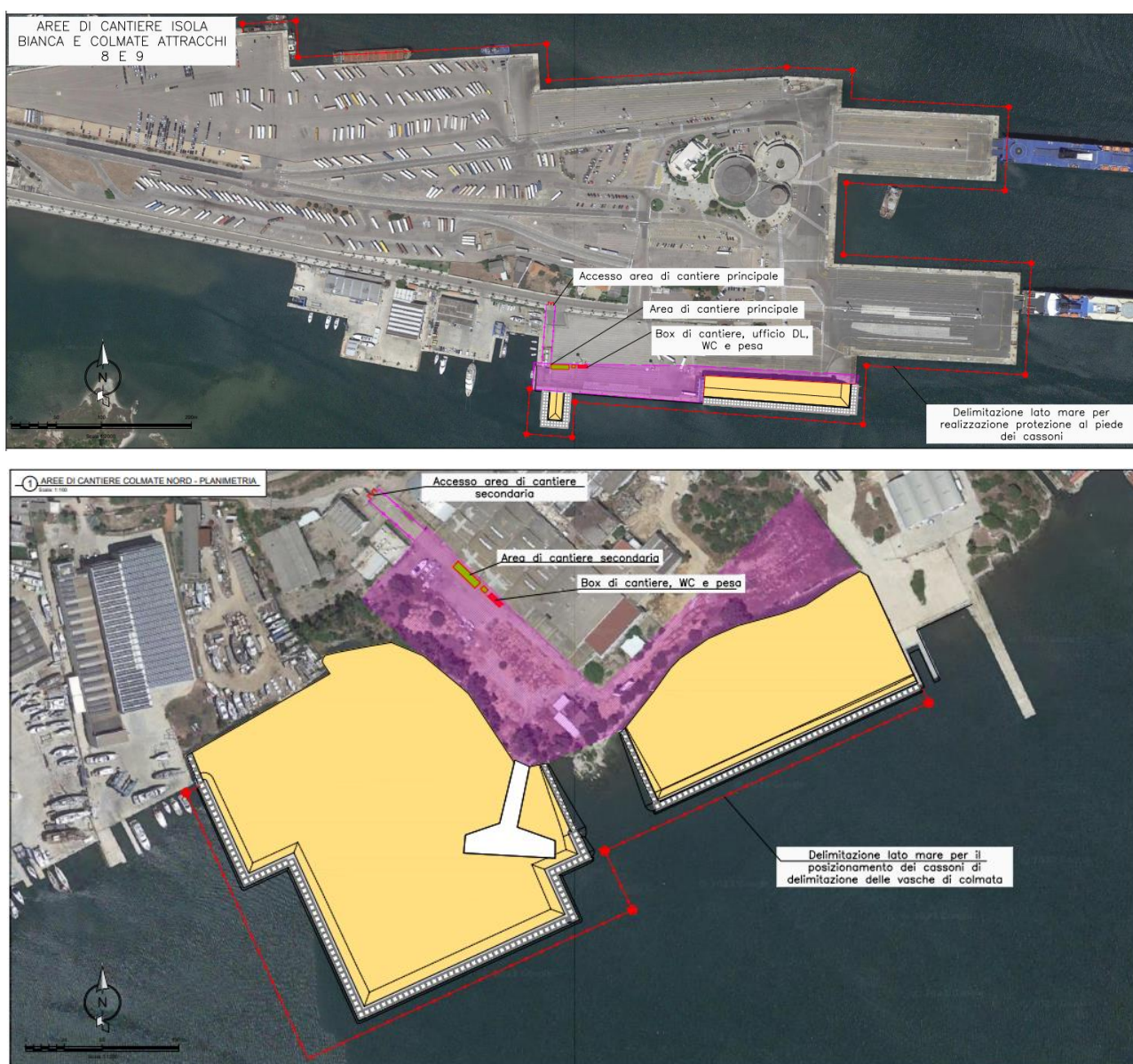
Figura 4-1. Individuazione delle aree di cantiere principale presso Isola Bianca (sopra) e dell'area di cantiere secondaria presso l'ex pontile Palmera (sotto).
