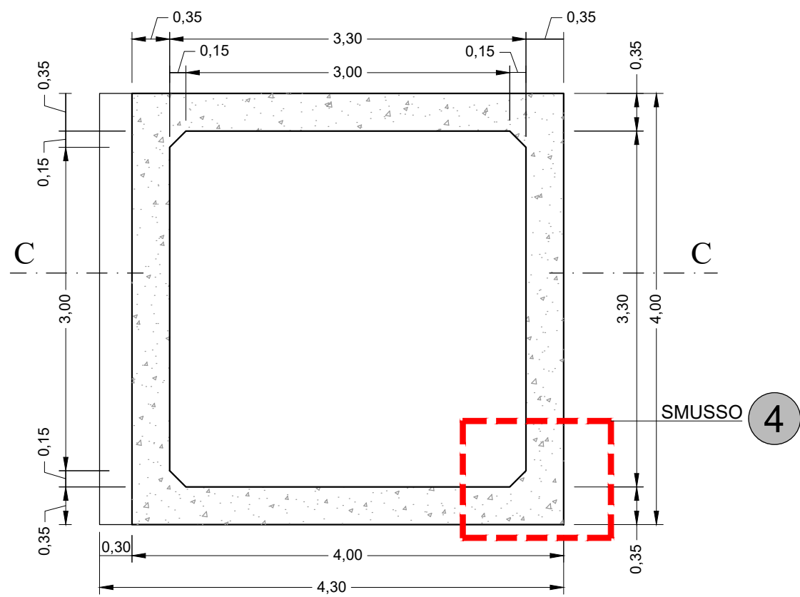
2 CASSONE MONOCELLULARE ANGOLARE TIPO 1b E 2b - PIANTA
