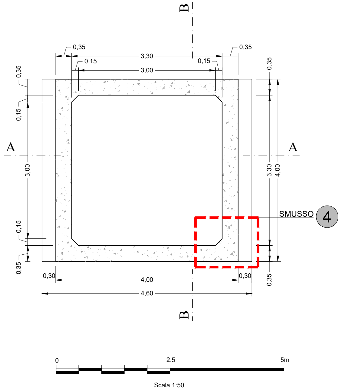
2 CASSONE MONOCELLULARE ANGOLARE TIPO 1b E 2b - PIANTA
