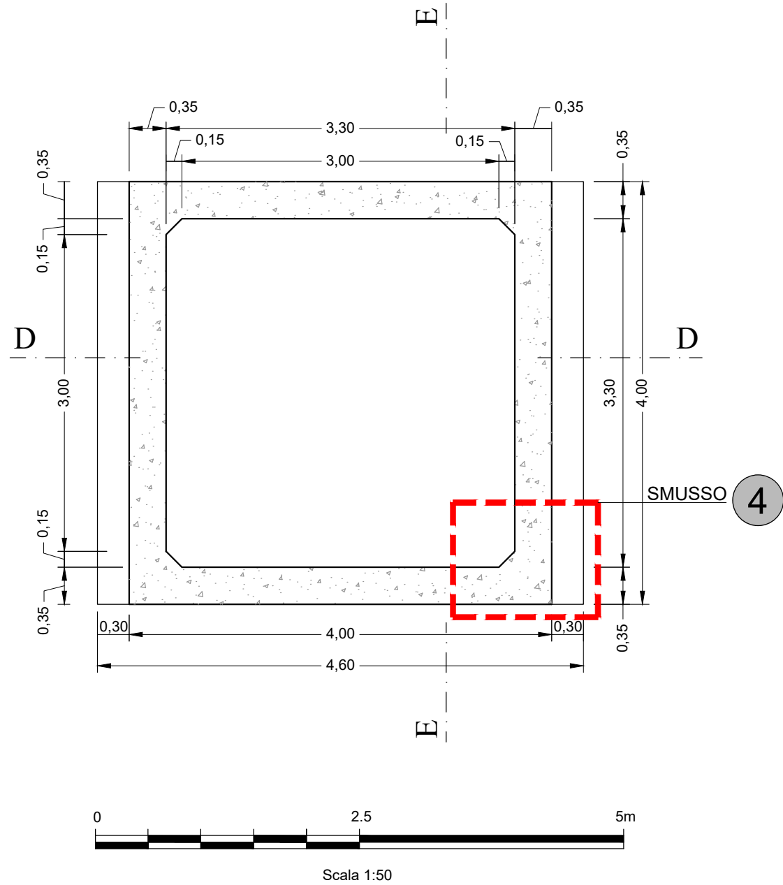
3 CASSONE MONOCELLULARE TIPO 2 - PIANTA
