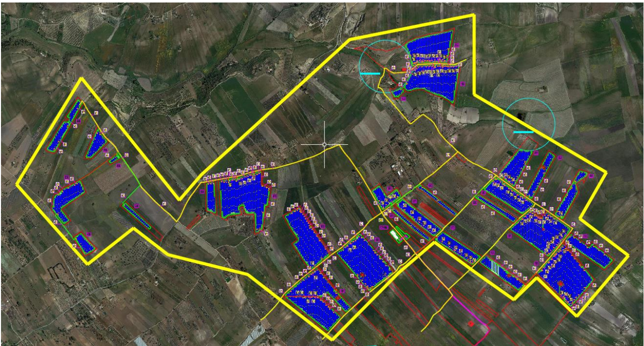
Figura 2 - Planimetria generale impianto
