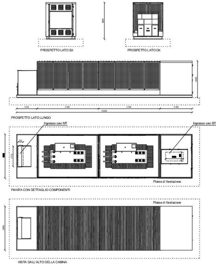
Figura 11 Tipico Cabina MT/bt
