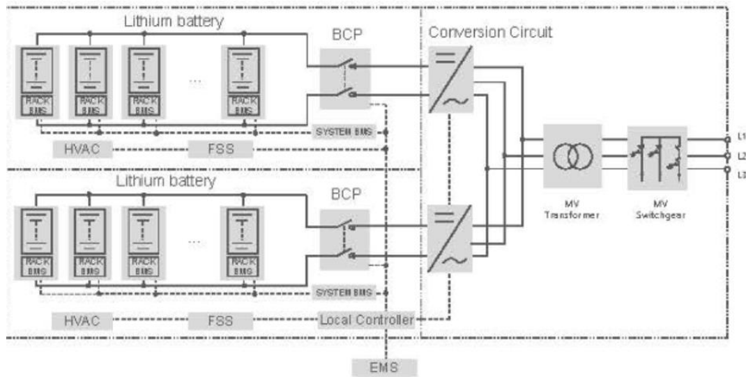
Figura 14 - Schema elettrico sistema di accumulo
