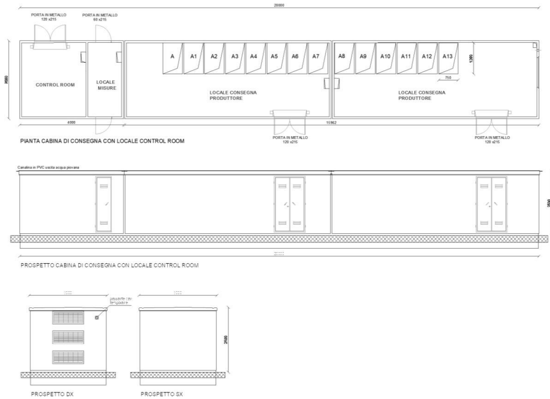
Figura 12 - Cabina di raccolta 20 m x 3 m e control room
