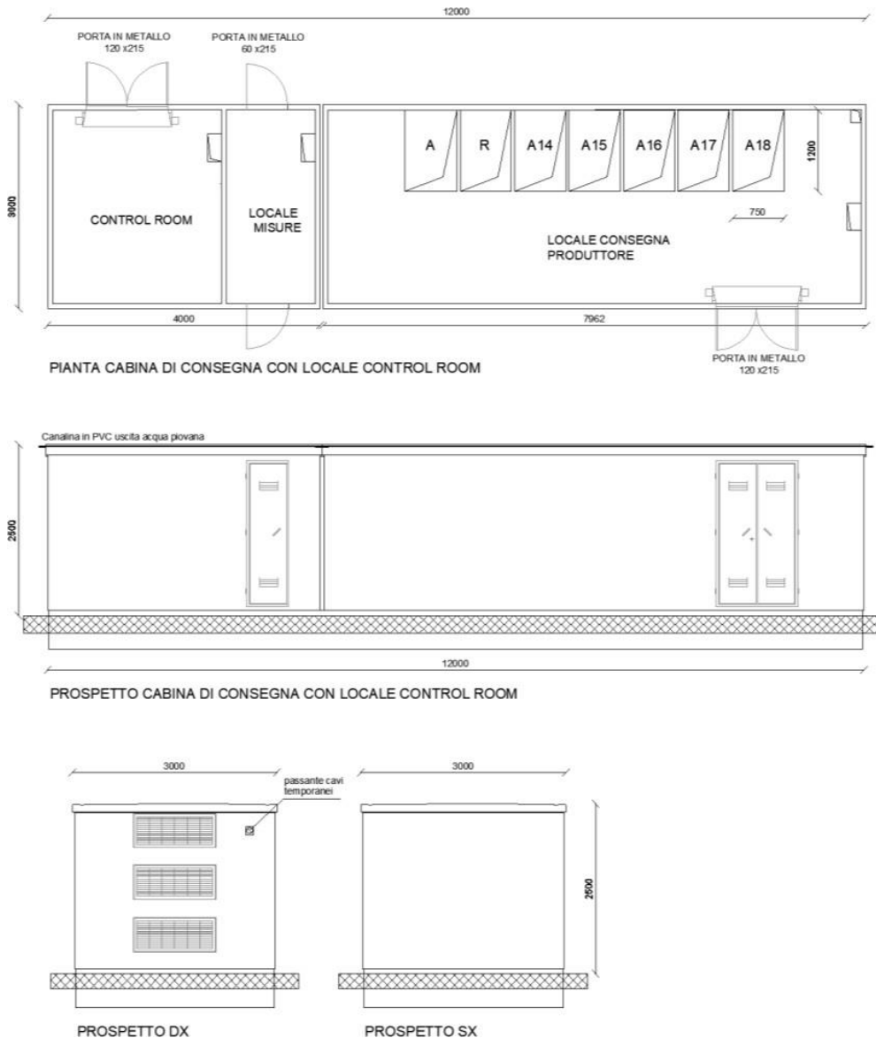
Figura 13 - Cabina di raccolta/generale 12m x 3m e control room
