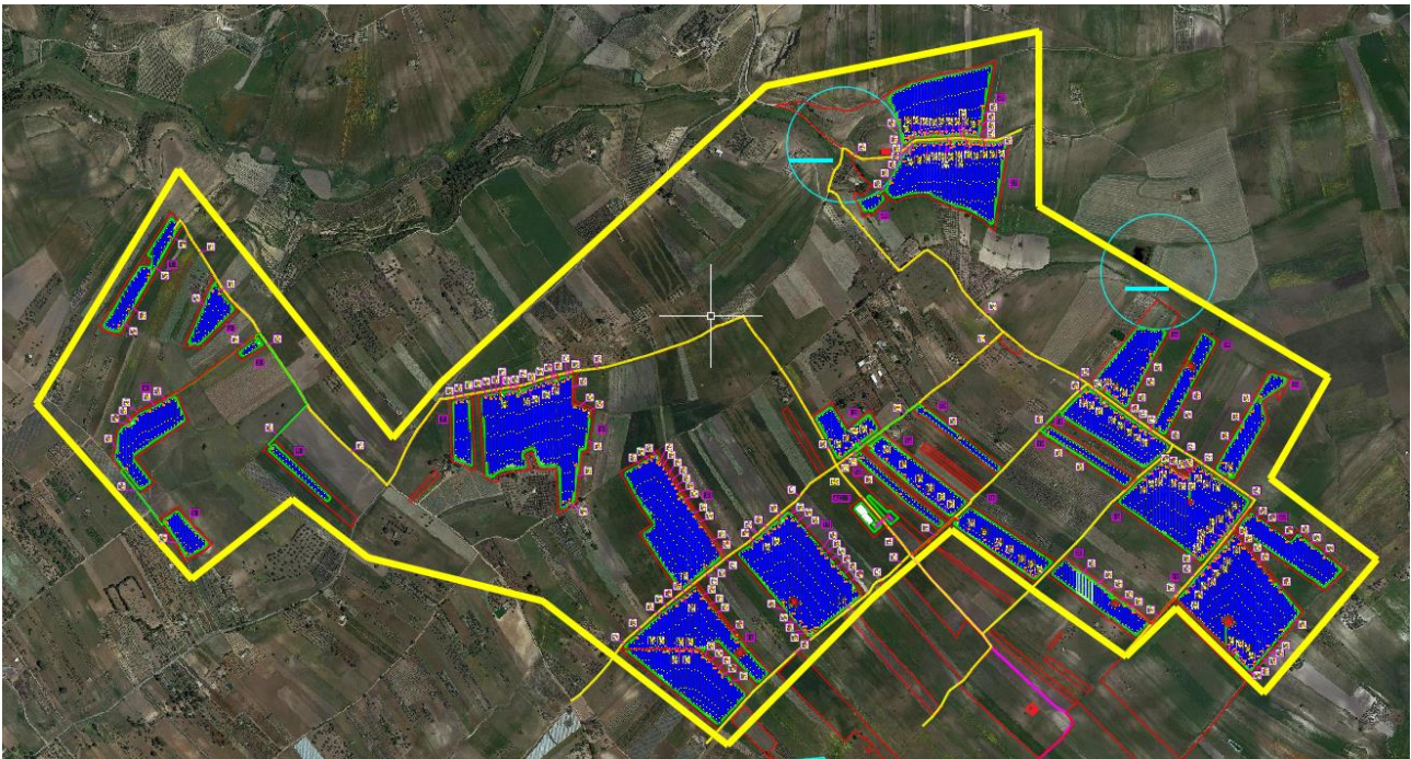
Figura 1 - Planimetria generale impianto
