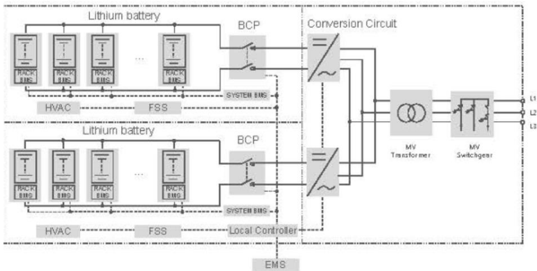
Figura 9 - Schema elettrico sistema di accumulo
