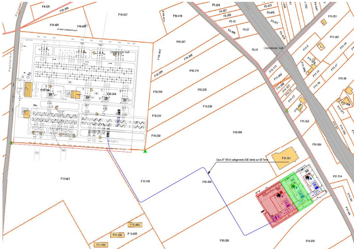
Figura 1 – Planimetria generale SSE Chiaramonte Gulfi (RG) e Stallo condiviso
