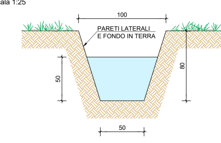
SEZIONE TIPO FOSSO DI GUARDIA TRA I PANNELLI scala 1:25
