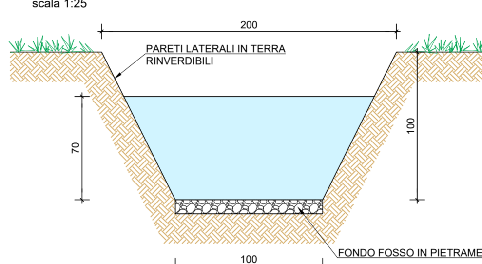
SEZIONE TIPO FOSSO DI GUARDIA PERIMETRALE scala 1:25
