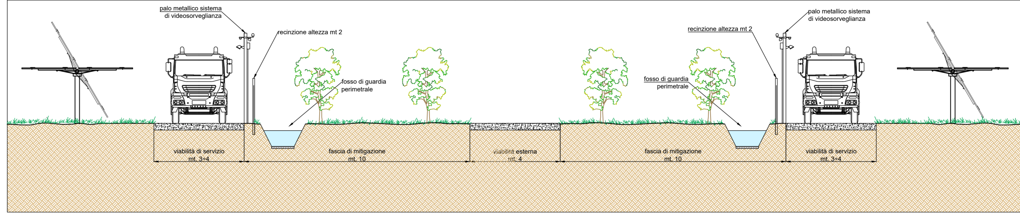
SEZIONE B-B (VIABILITA' TIPO TRA PARTICELLE CONFINANTI) scala 1:100
