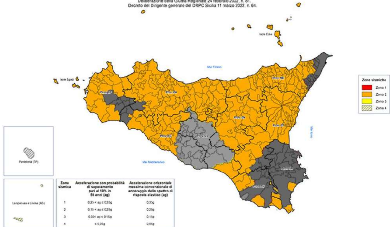
Figura 37. Classificazione sismica regionale
