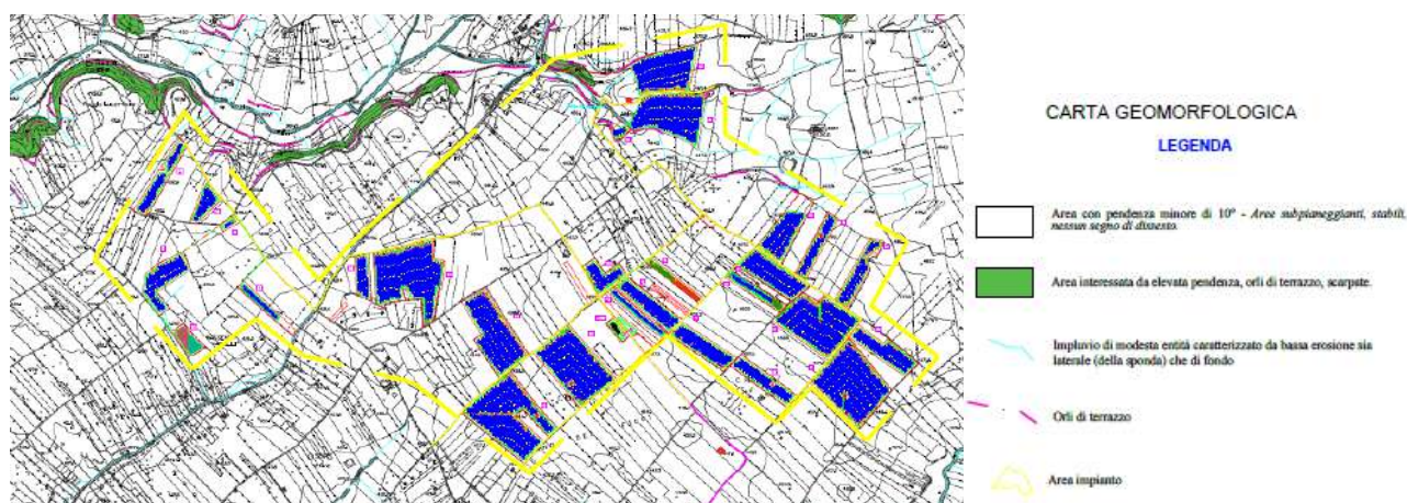
Figura 33. Stralcio carta geomorfologica
