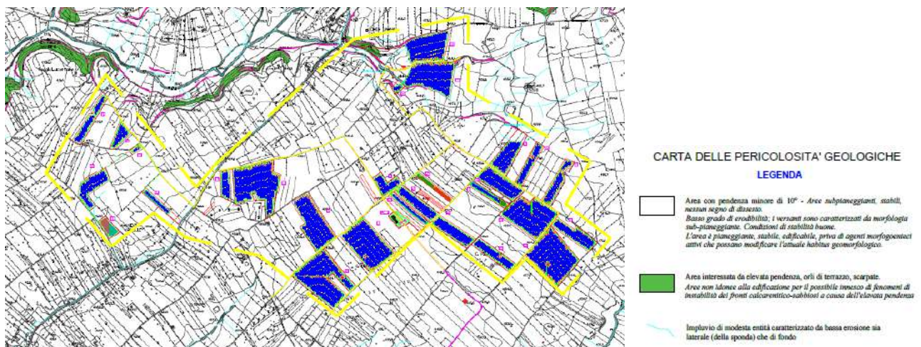
Figura 32. Stralcio carta delle pericolosità geologiche
