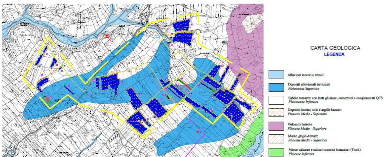
Figura 30. Stralcio carta geologica
