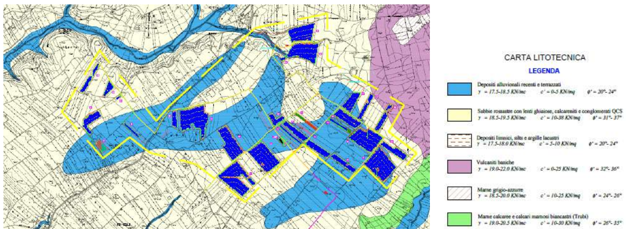
Figura 31. Stralcio carta litotecnica
