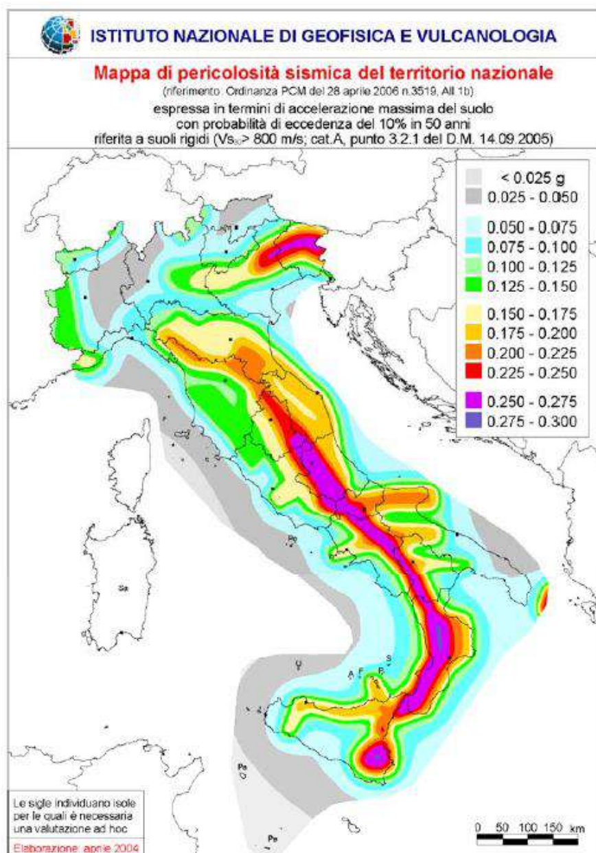
Figura 36. Mapa di pericolosità sismica del territorio nazionale
