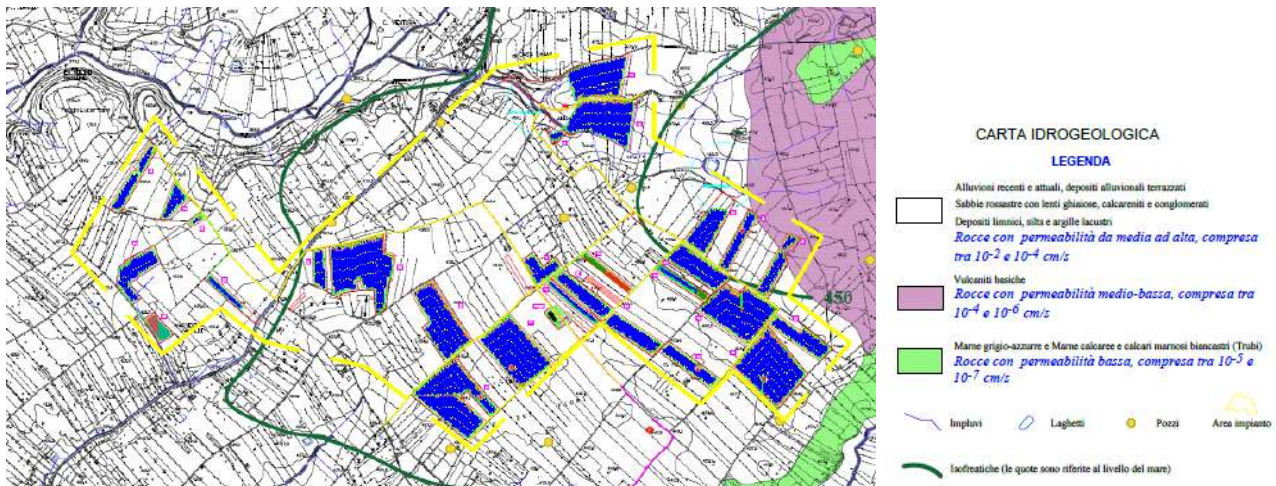
Figura 34. Stralcio carta idrogeologica
