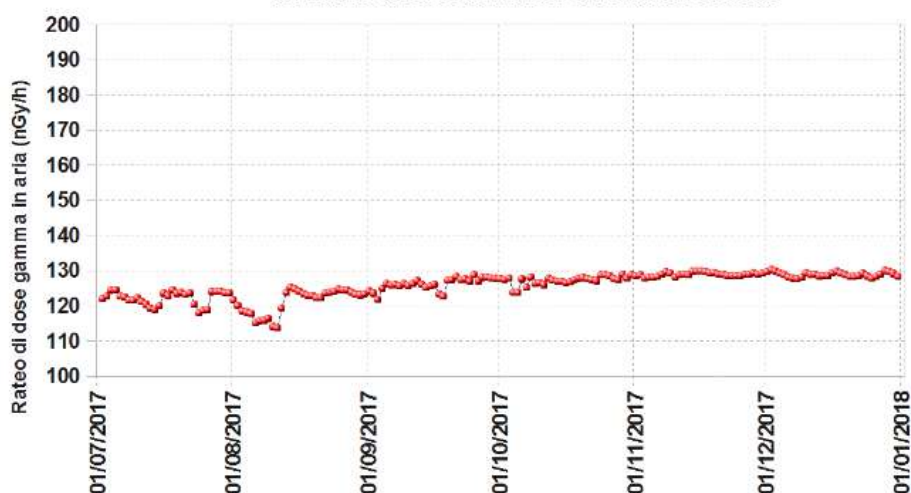
Figura 46: Valori della dose gamma in aria, misurati nella stazione ARPA Sicilia di Palermo (via Nairobi). La misura avviene in continuo durante tutto l'anno mediante camera a ionizzazione secondo le indicazioni delle linee guida ISPRA. [fonte: Agenti fisici, ARPASicilia, 2019]
