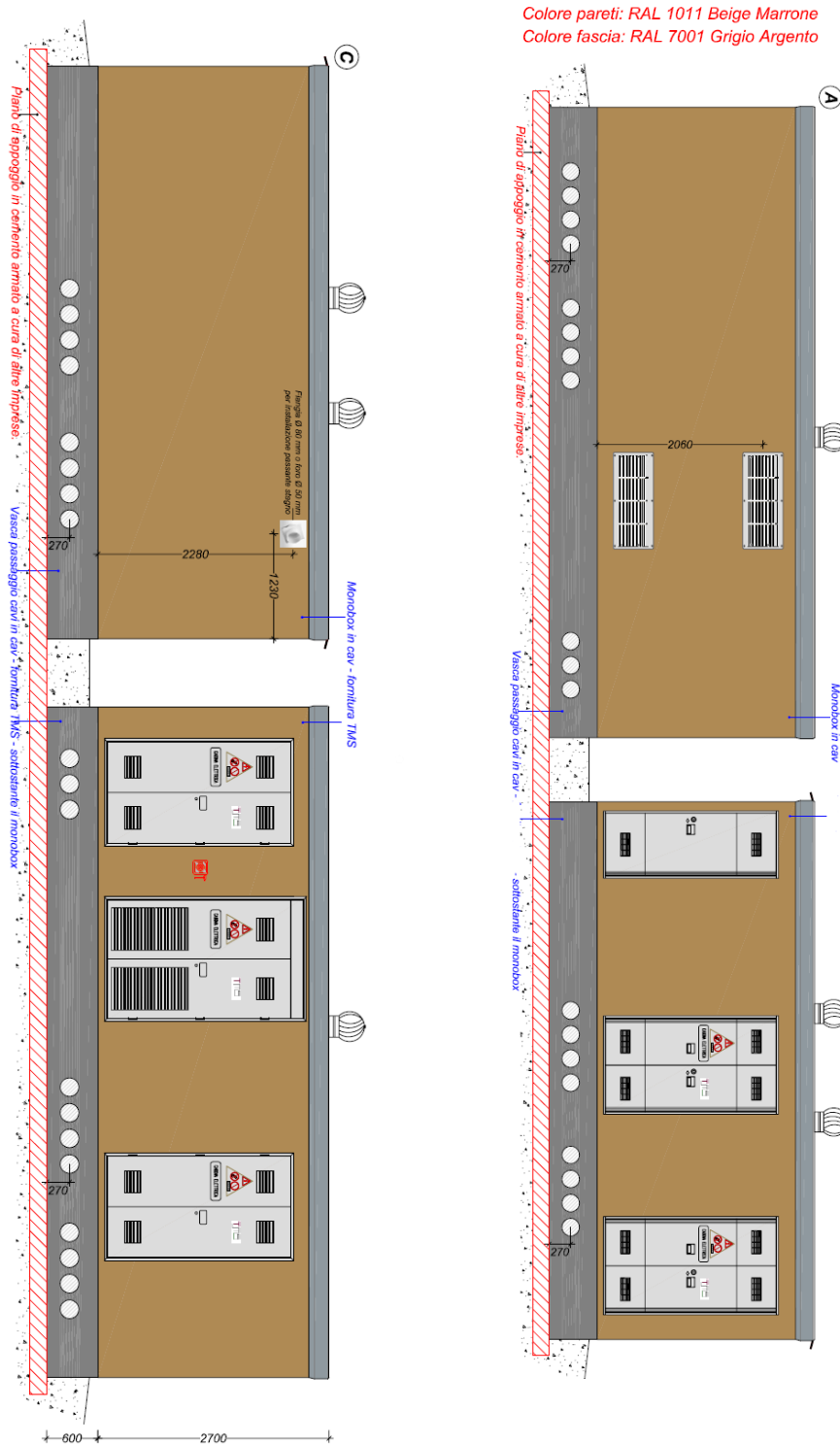
Figura 1: Prospetto tipo Cabina Enel + Cabina Utente
