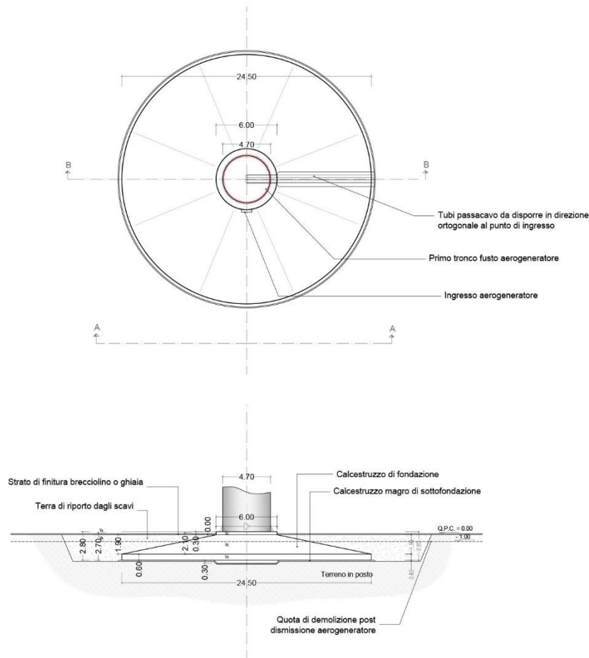
Figura 1 – Pianta e vista della fondazione tipo dell'aerogeneratore
