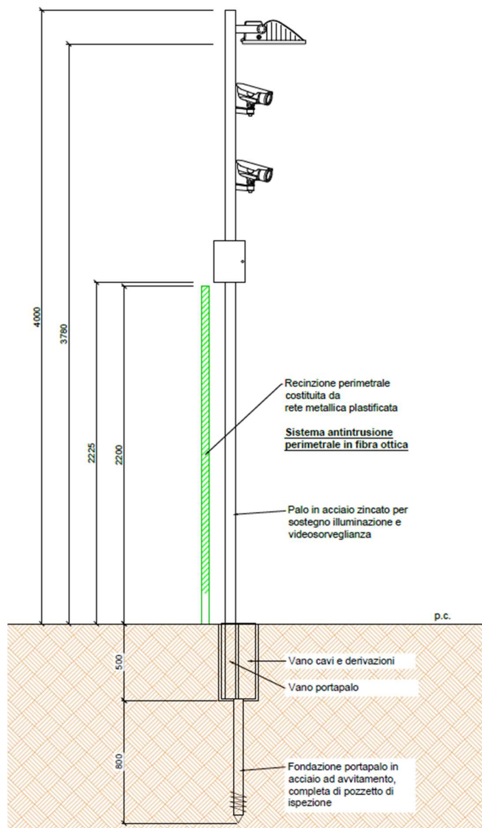
Figura 4. Particolari dell'infissione dei pali per telecamere TVCC
