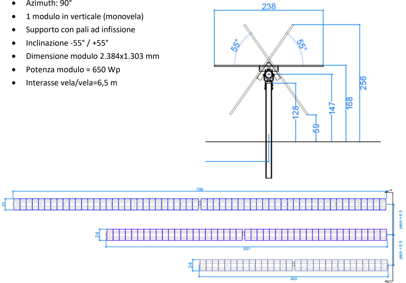
Figura 3. Struttura di supporto moduli
