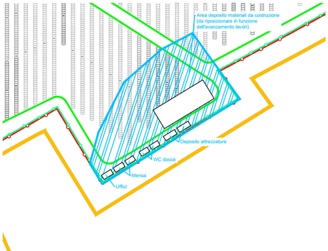
Figura 2. Individuazione delle aree di cantiere (NW– SE)
