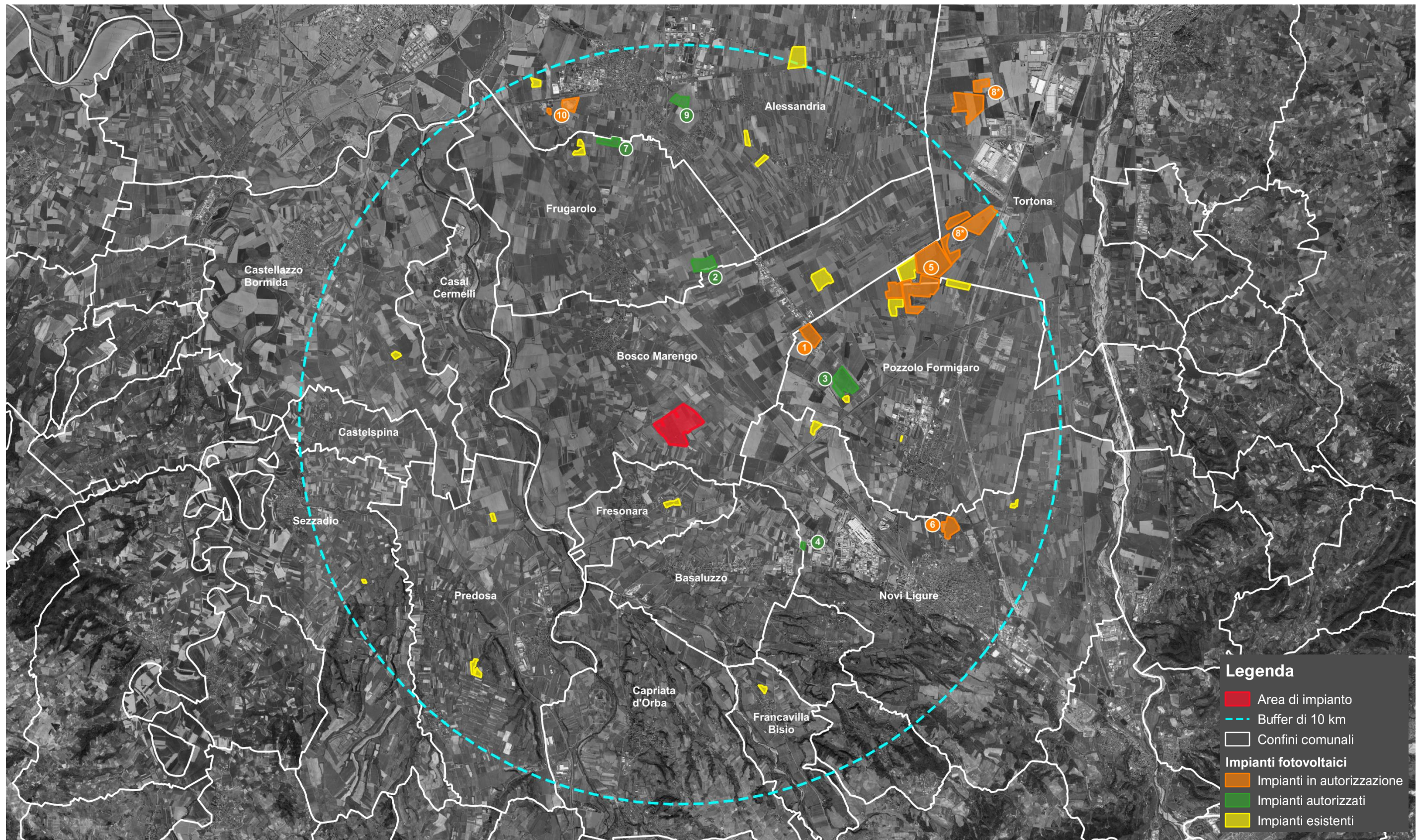
Tavola 2. Localizzazione dell'area di progetto (superficie in rosso) rispetto agli impianti fotovoltaici "REALIZZATI" (superfici in giallo), "IN AUTORIZZAZIONE" (superfici in arancione) e "AUTORIZZATI" (superfici in verde), presenti all'interno di un buffer di 10 km (cerchio azzurro tratteggiato), dall'area di intervento. *L'impianto identificato con il codice numerico 8 risulta suddiviso in più lotti di impianto.
