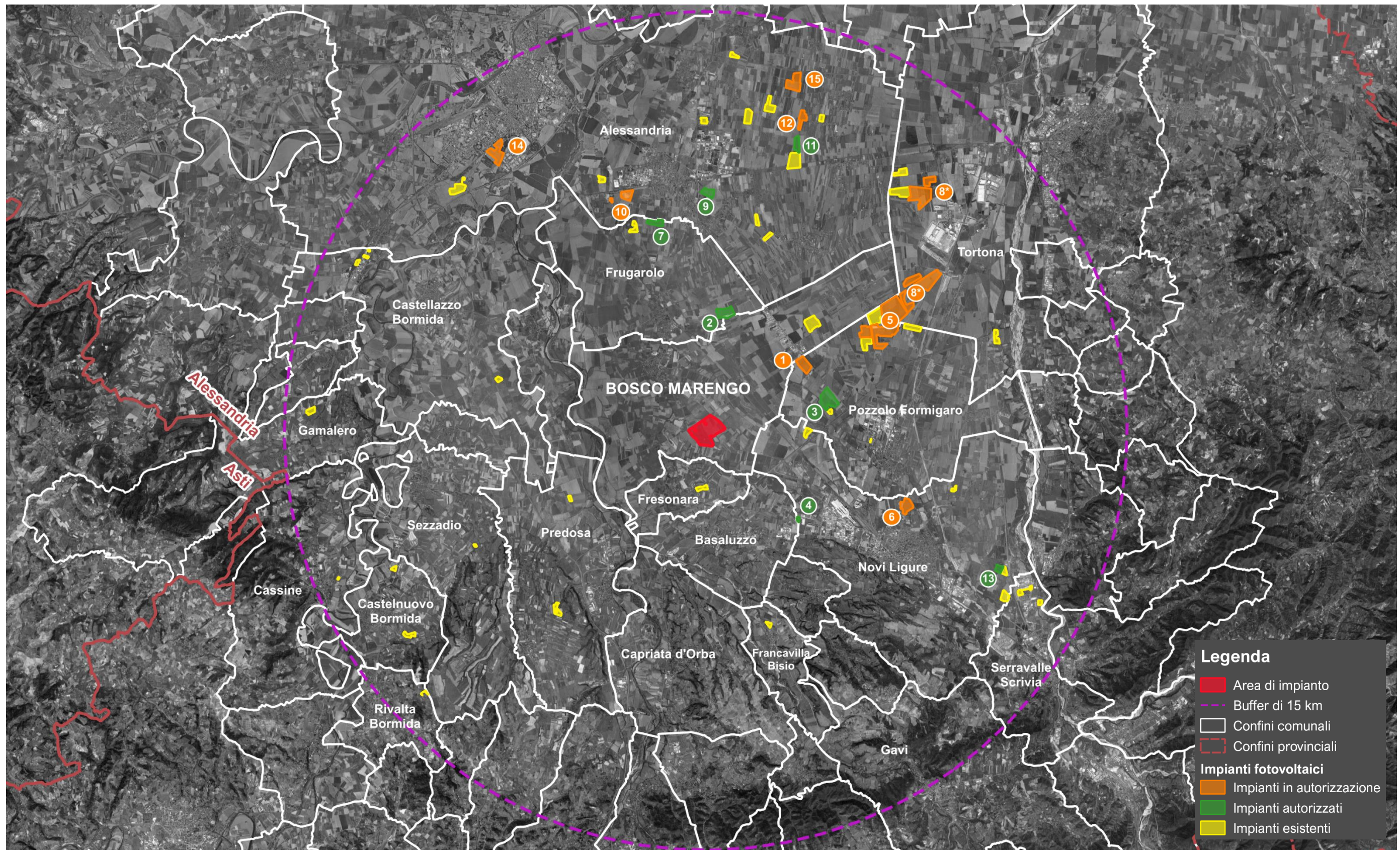
Tavola 3. Localizzazione dell'area di progetto (superficie in rosso), rispetto agli impianti fotovoltaici "REALIZZATI" (superfici in giallo), "IN AUTORIZZAZIONE" (superfici in arancione) e "AUTORIZZATI" (superfici in verde), presenti all'interno di un buffer di 15 km (cerchio in viola tratteggiato) dall'area di intervento. *L'impianto identificato con il codice numerico 8 risulta suddiviso in più lotti.
