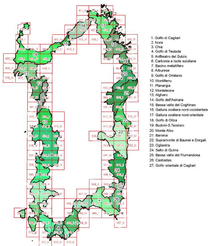
Figura 4 - Ambiti di paesaggio secondo il PPR Sardegna
