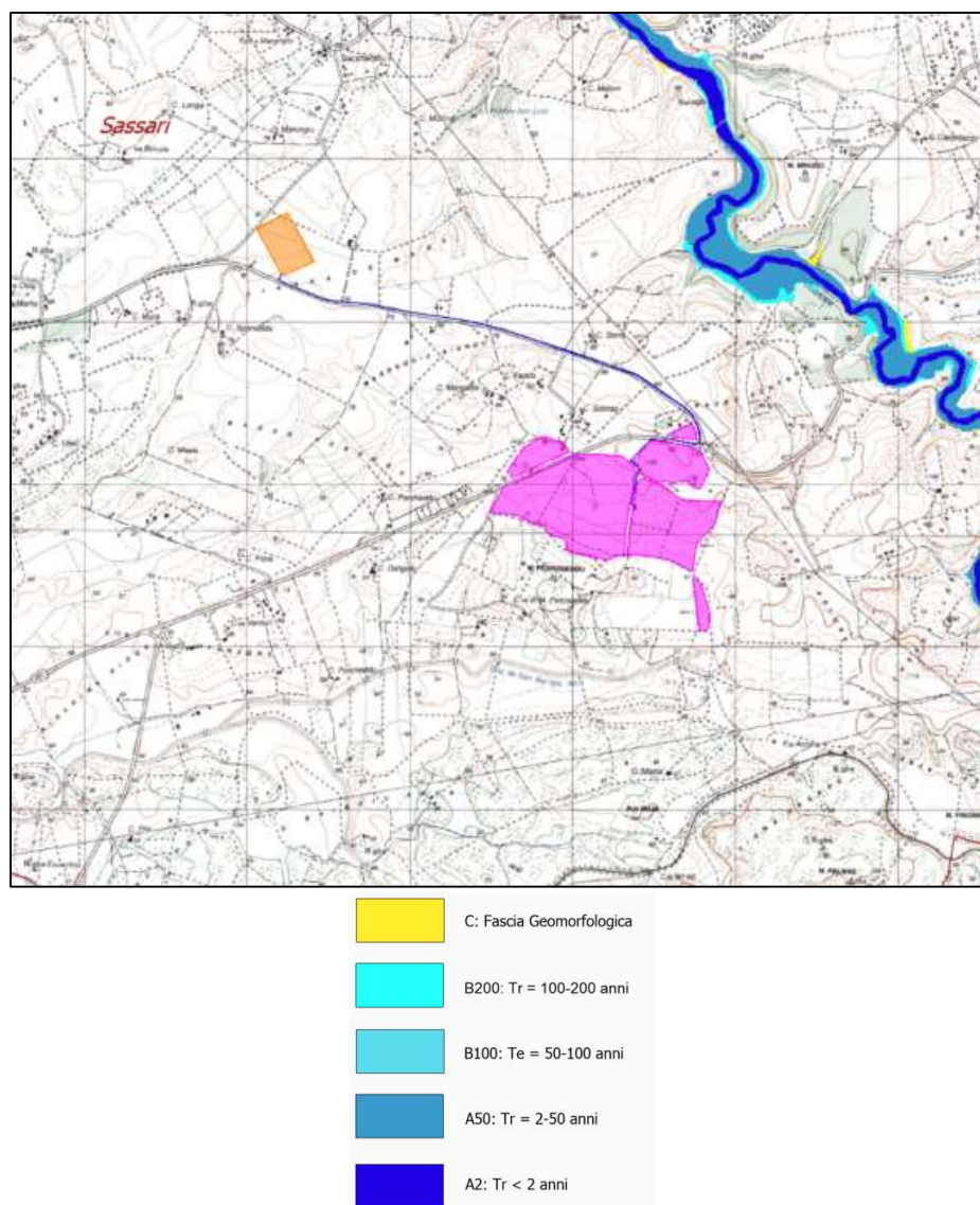
Figura 18 Inquadramento rispetto al PSFF
