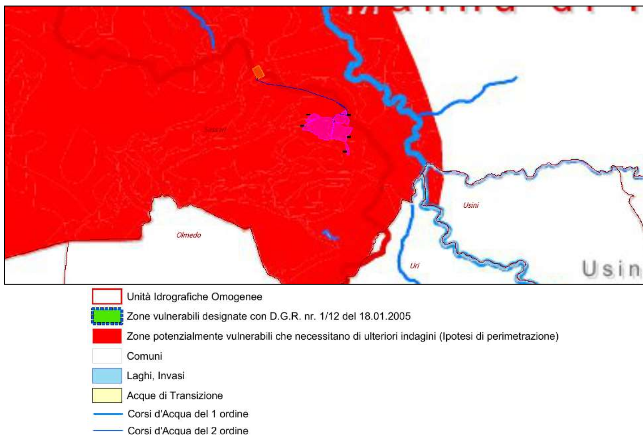
Figura 23 Designazione zone vulnerabili da nitrati (Tav.9)
