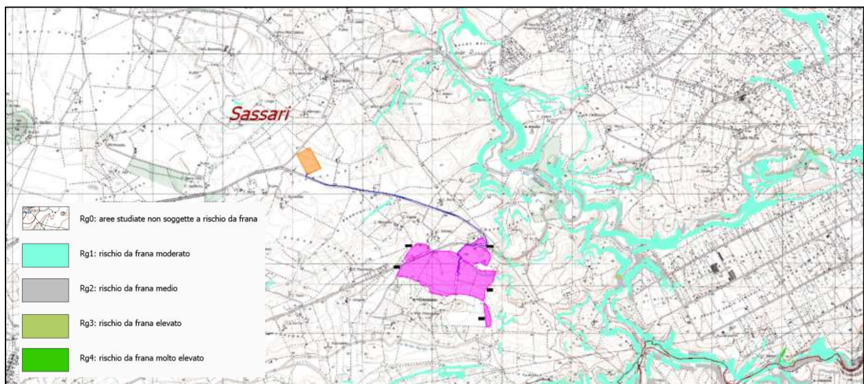
Figura 15 Inquadramento rispetto al rischio geomorfologico PAI Sardegna
