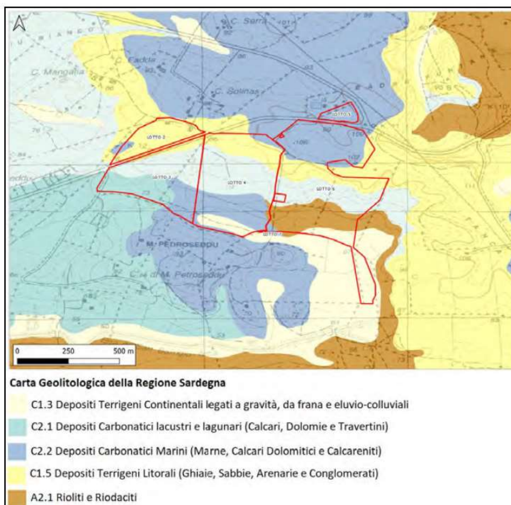
Figura 40 – Carta Litologica di dettaglio redatta dalla Regione Autonoma della Sardegna
