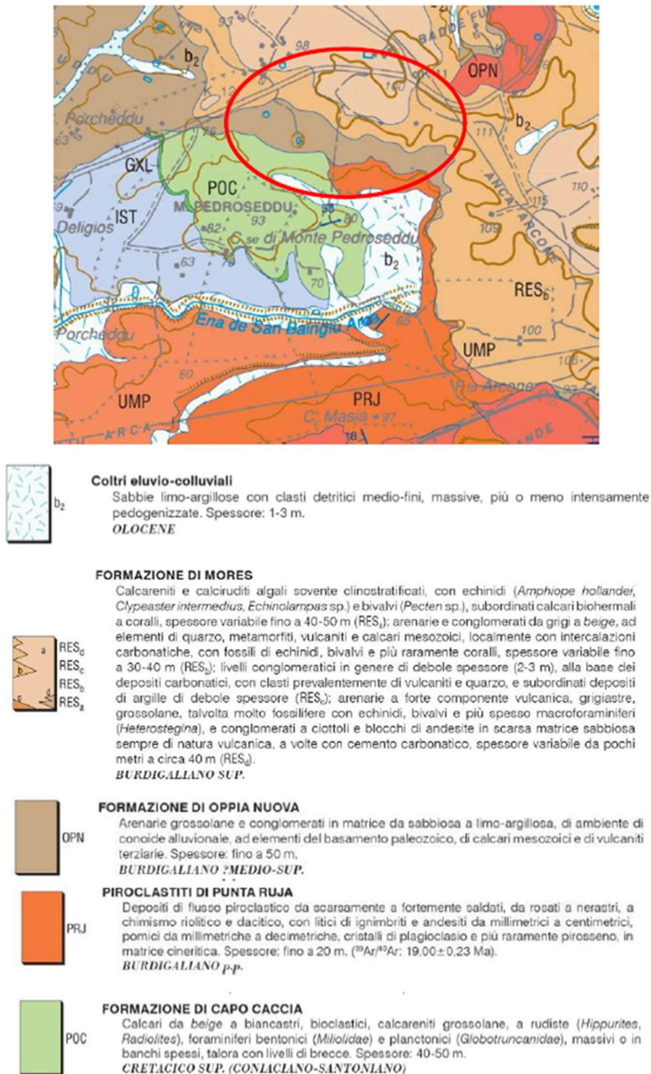
Fig. 7: stralcio del F.459 "Sassari" della Carta Geologica d'Italia in scala 1:50.000.
