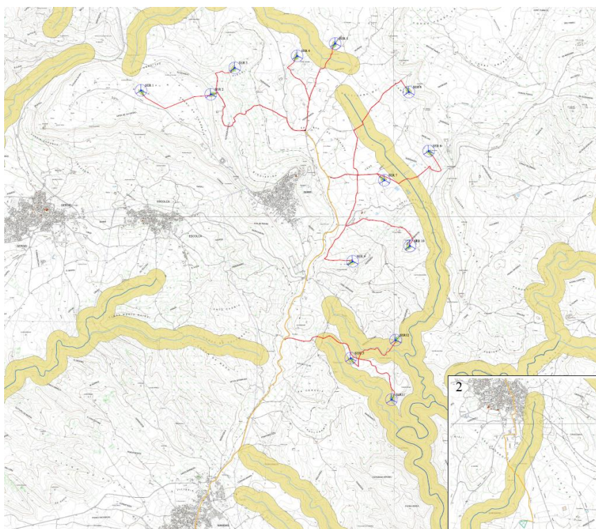
Figura 5. Impianto su cartografia fasce fluviali
