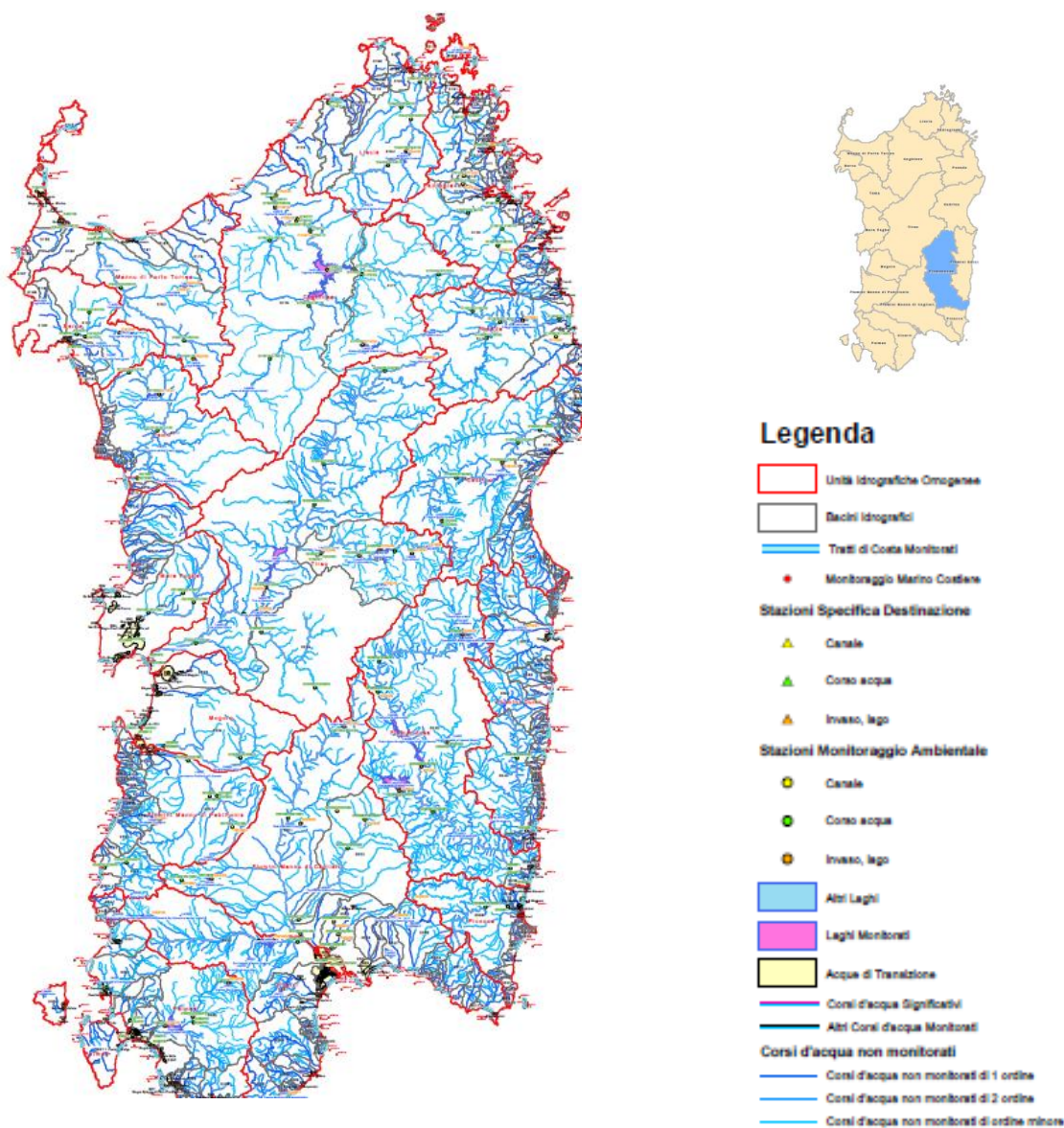
Unità idrogeologiche omogenee della Sardegna
