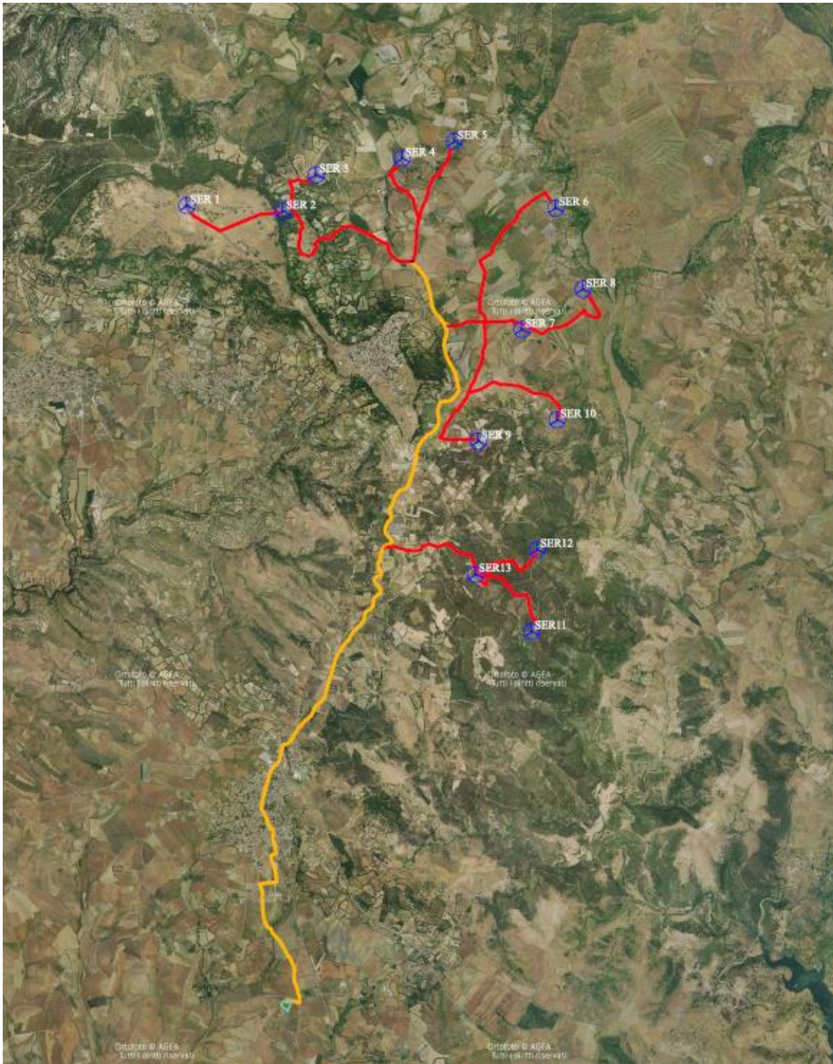
Figura 2. Planimetria di impianto su ortofoto
