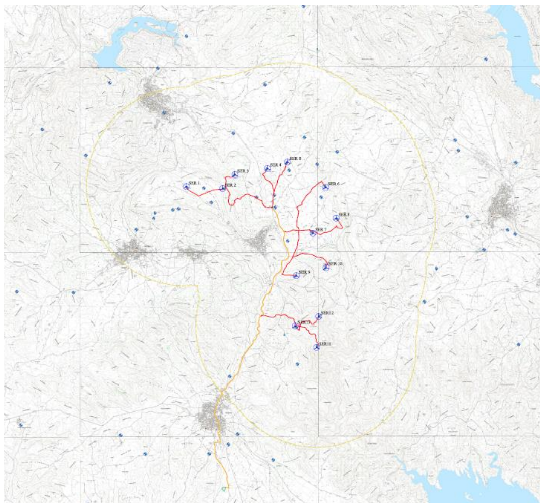
Figura 10. Cartografia con area di inviluppo di 3 km per pozzi e sorgenti
