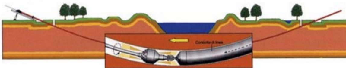
Figura 3. Tecnologia di trivellazione orizzontale controllata (TOC)
