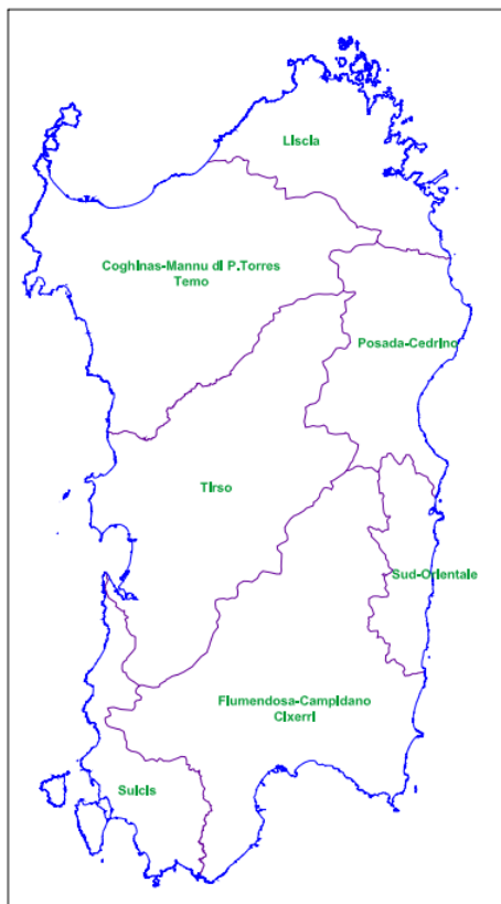
Figura 3. Delimitazione dei 7 sub-bacini regionali sardi.
