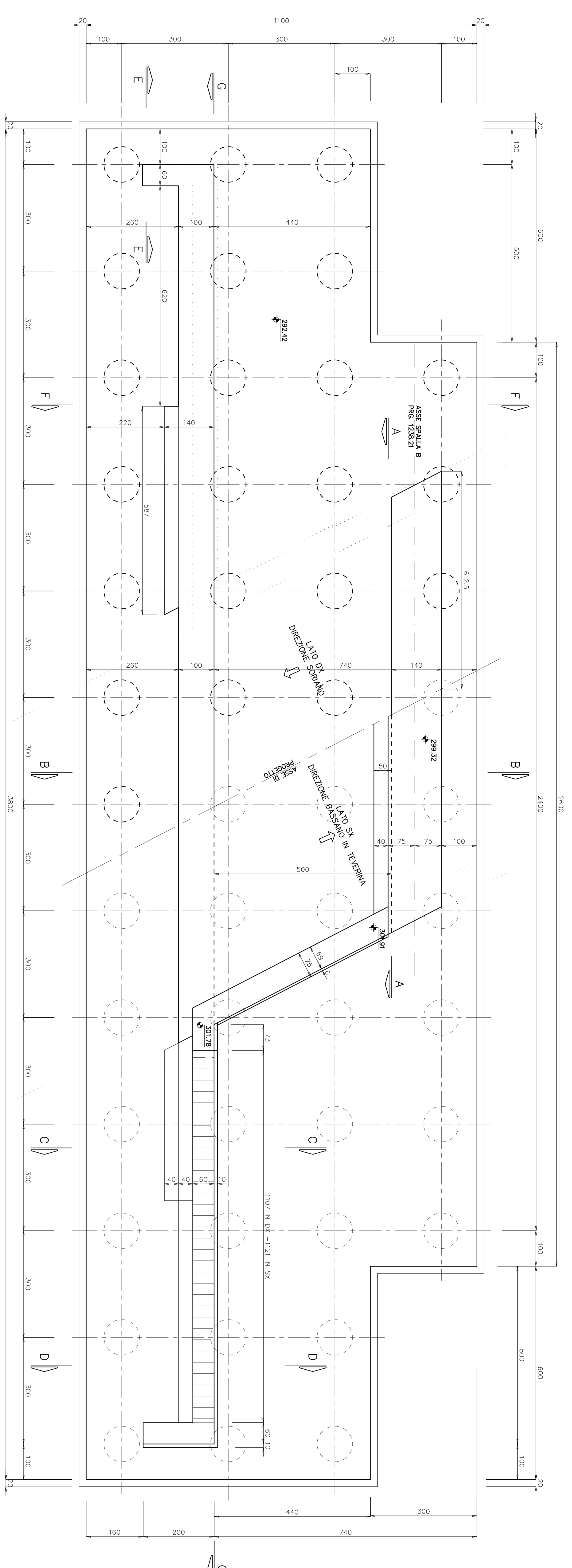
1/2 SEZIONE SPICCATO SPALLA SB scala 1:50 1/2 VISTA DALL' ALTO
