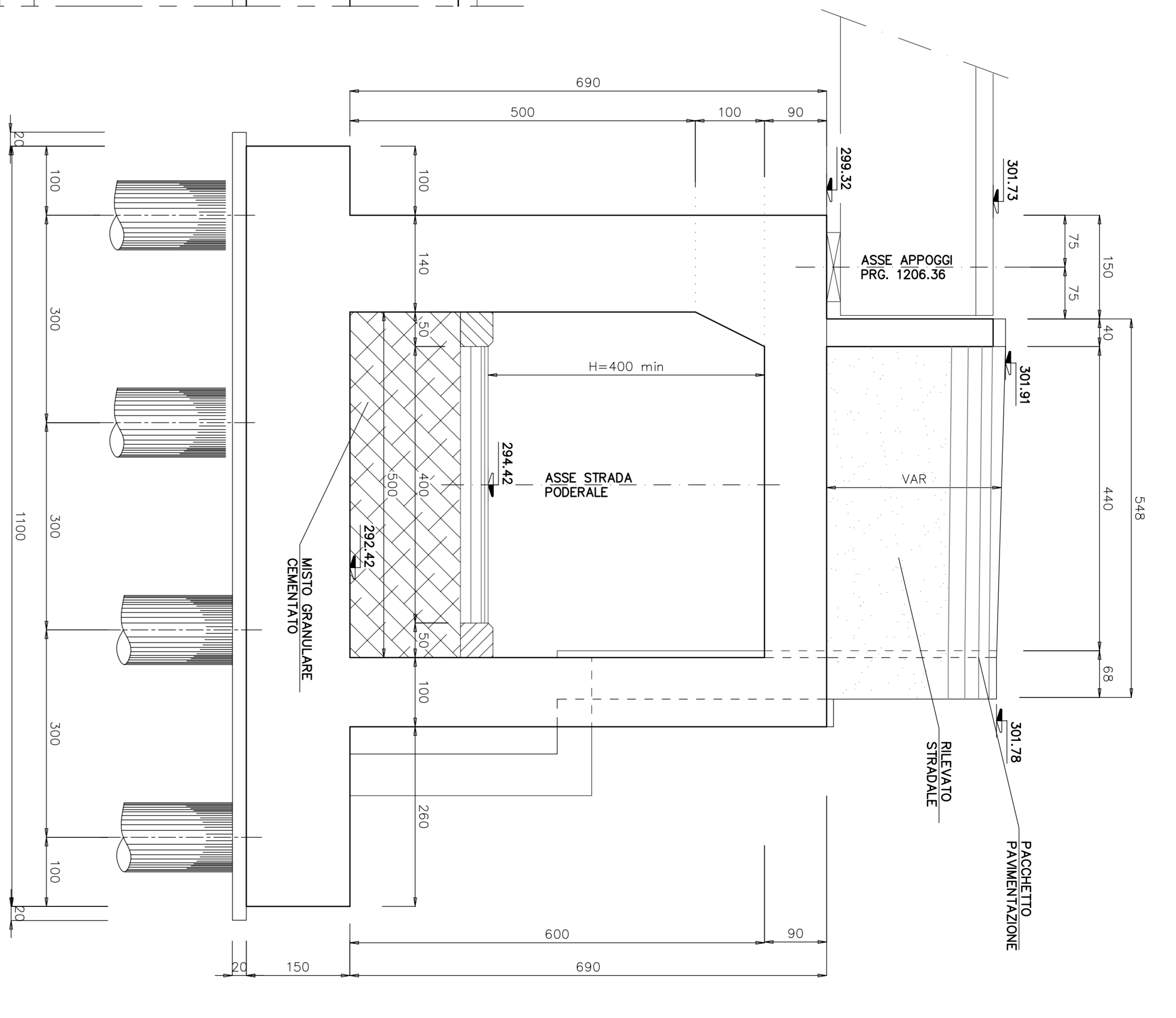
SEZIONE C-C scala 1:50 MURO TIPO 1
