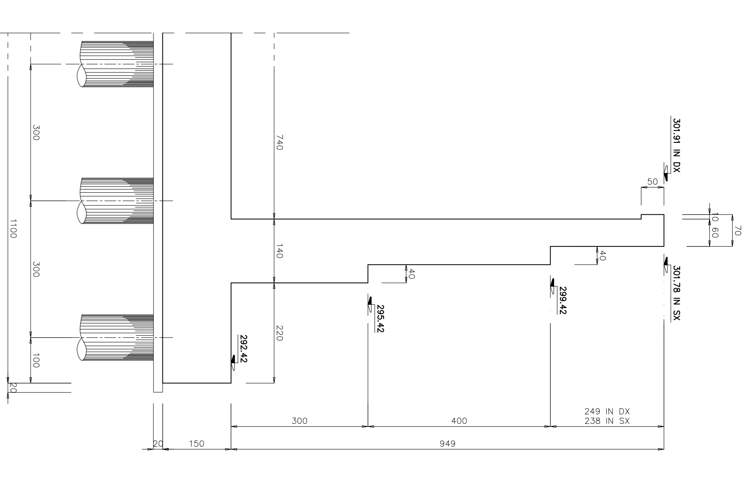
SEZIONE C-C scala 1:50 MURO TIPO 1
