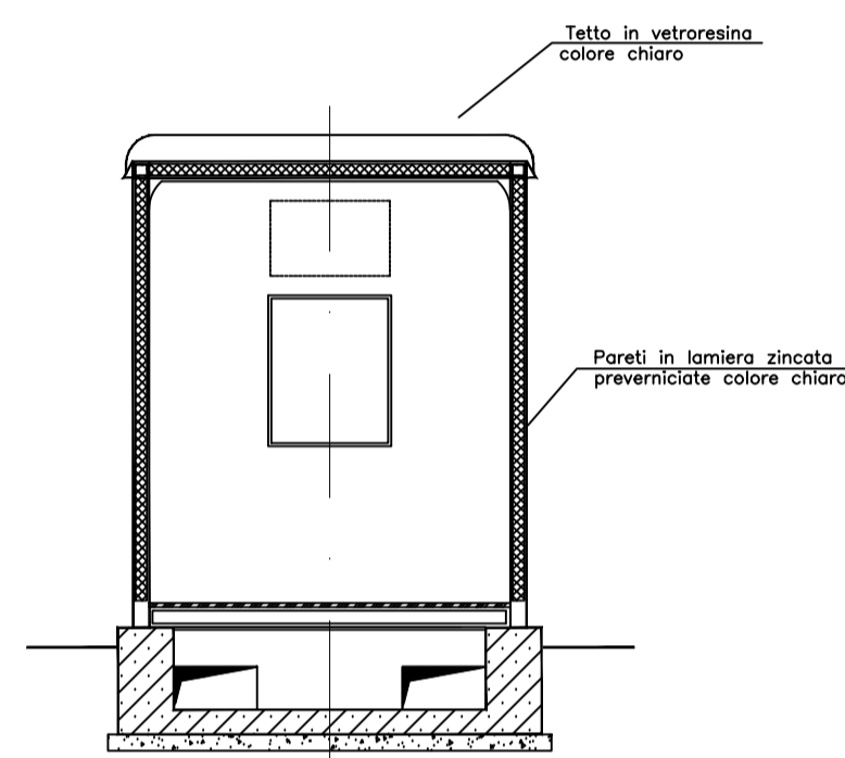
SEZIONE C-C
