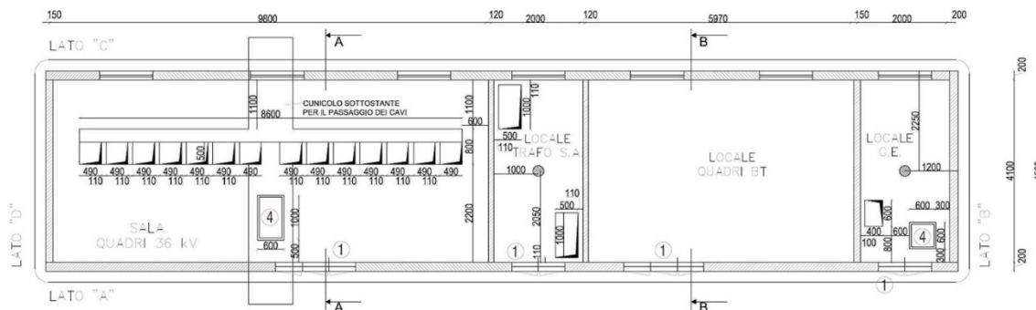
Figura 9: Tipico edificio comandi
