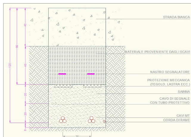
Figura 6: Esempio di tipico di scavo per posa cavidotto a 36 kV su strada bianca.
