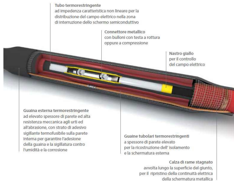
Figura 4: Esempio di giunto per cavo a 36 kV
