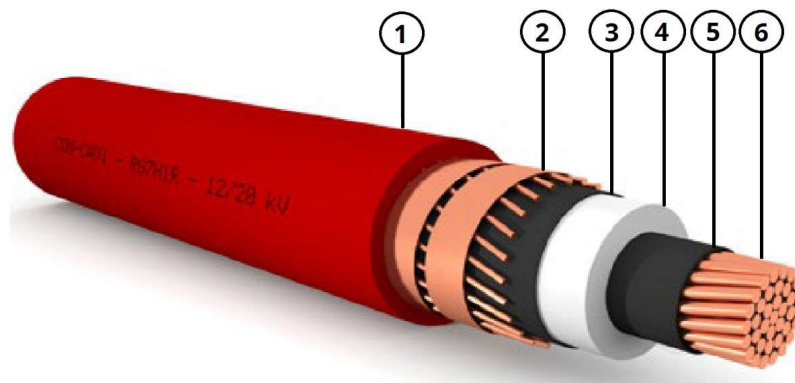
Figura 3: Parti costituenti un cavo unipolare MT: 1) Guaina esterna; 2) Schermo metallico; 3) Semiconduttivo esterno; 4) Isolante; 5) Semiconduttivo interno; 6) Conduttore
