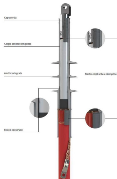
Figura 5: Esempio di terminale per cavo 36 kV
