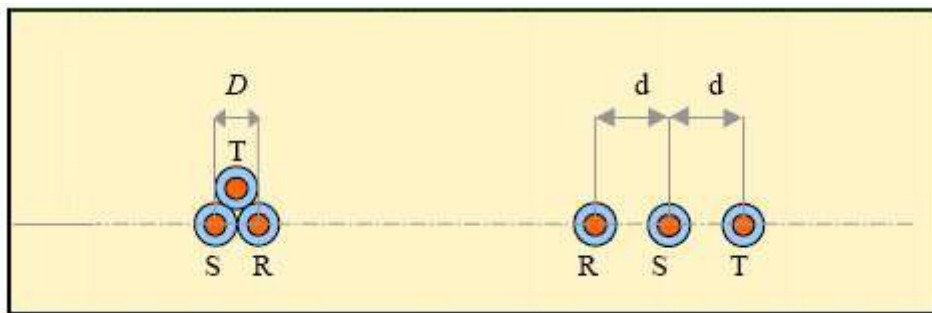
Figura 7: Disposizioni tipiche di posa per cavi unipolari
