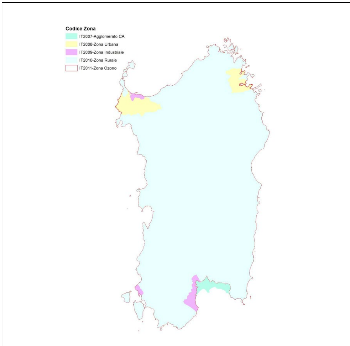
Figura 14. Zonizzazione della Regione Sardegna ai fini della valutazione e gestione della qualità dell'aria
