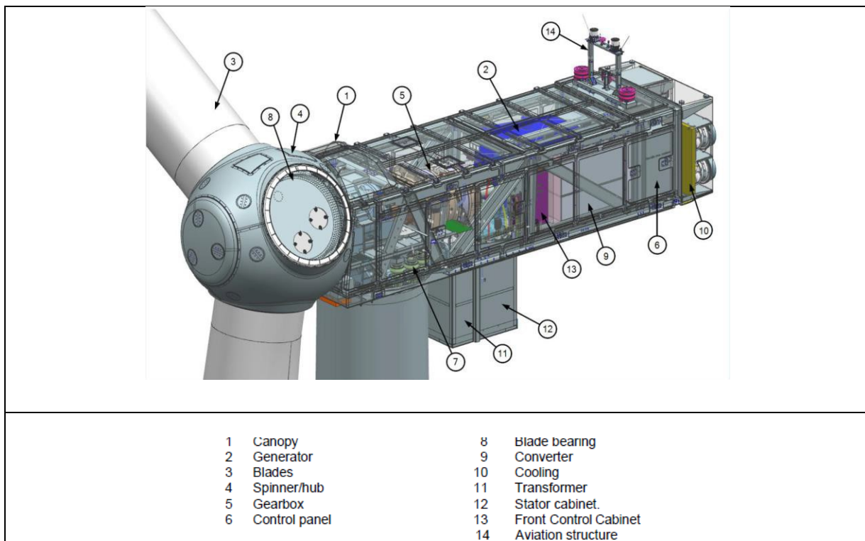
Figura 4. Rappresentazione grafica di una navicella
