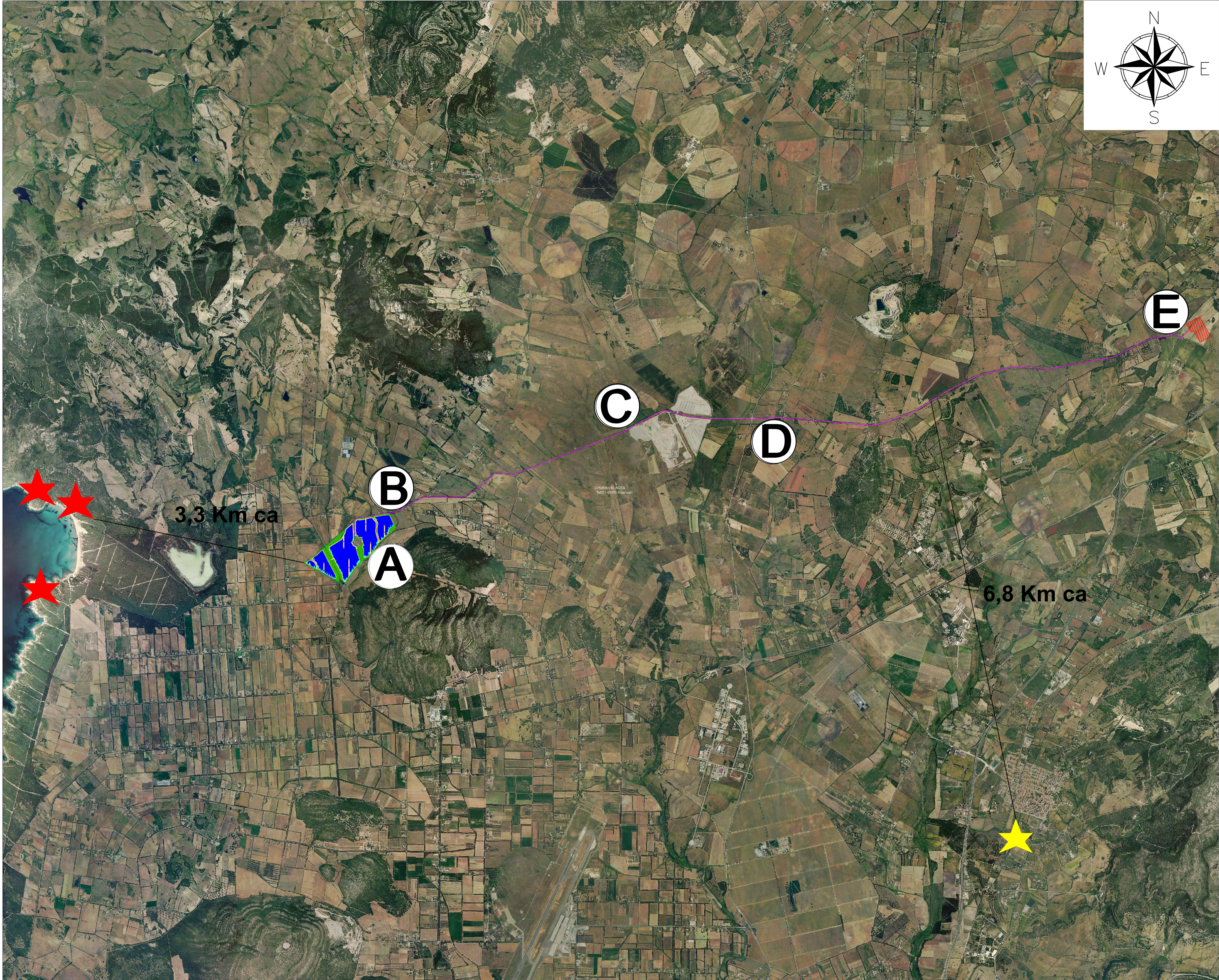
Layout Impianto, Cavidotto e Punto di Connessione su Carta Repertorio Beni 2017
