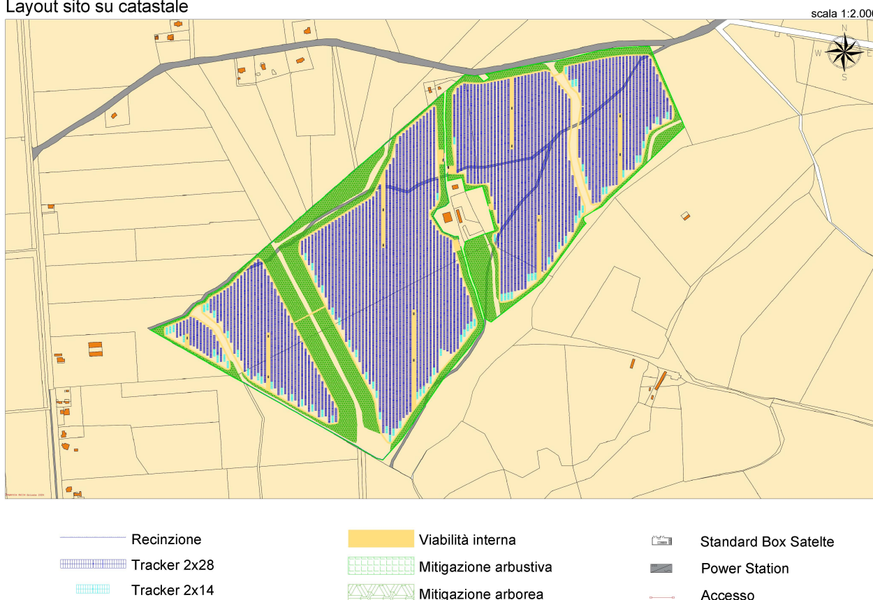
Figura 2 – Layout dell'area d'impianto ricadente nel territorio di Sassari (SS) località “Su Bacchileddu”, su base catastale
