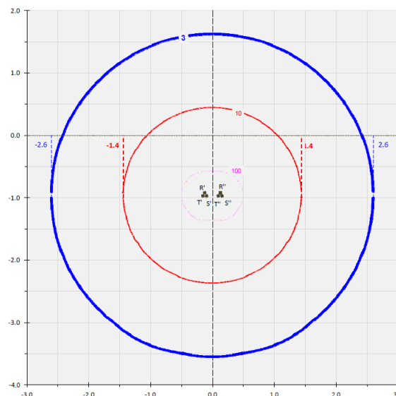
Figura 7 - Curve di equivello per il campo di induzione magnetica generato da una linea M.T. posata a trifoglio ( I_{max}=720\text{A} ; formazione (3x1x630))
