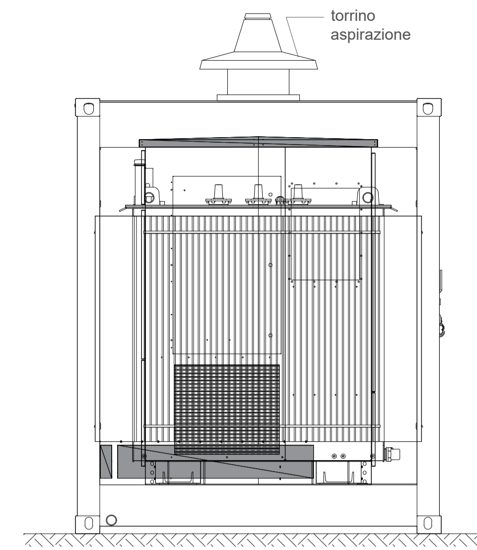
PROSPETTO OVEST
