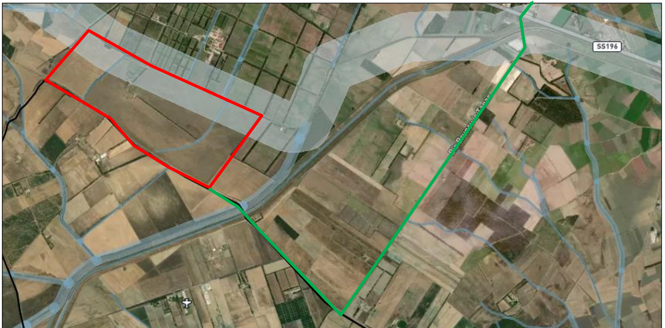
Fig. 7.1.2/A: perimetrazione aree a pericolosità idraulica
