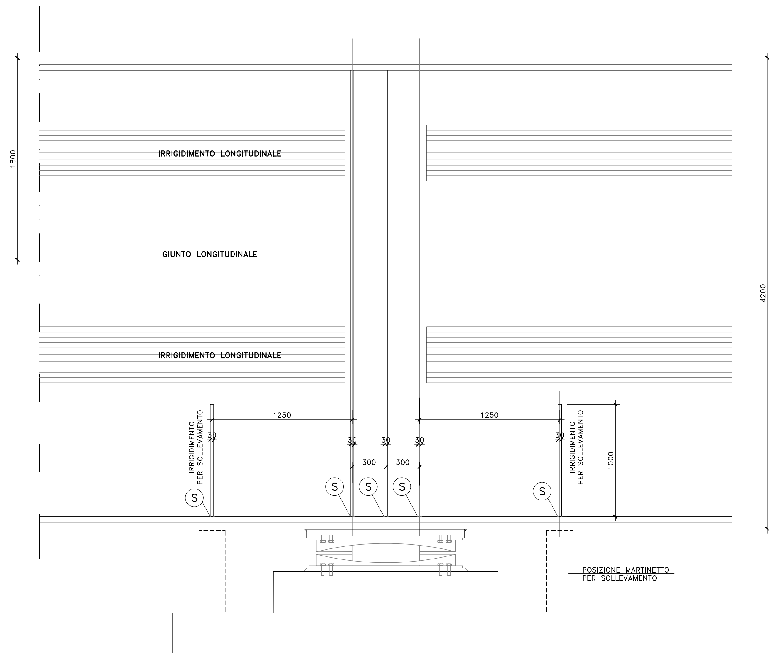
IRRIGIDIMENTI PER SOLLEVAMENTO SCALA 1:20
