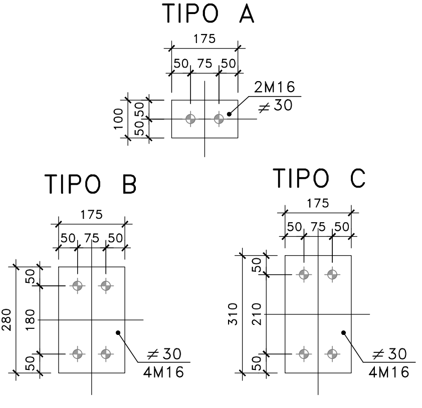
DETTAGLIO CALASTRELLI SCALA 1:10
