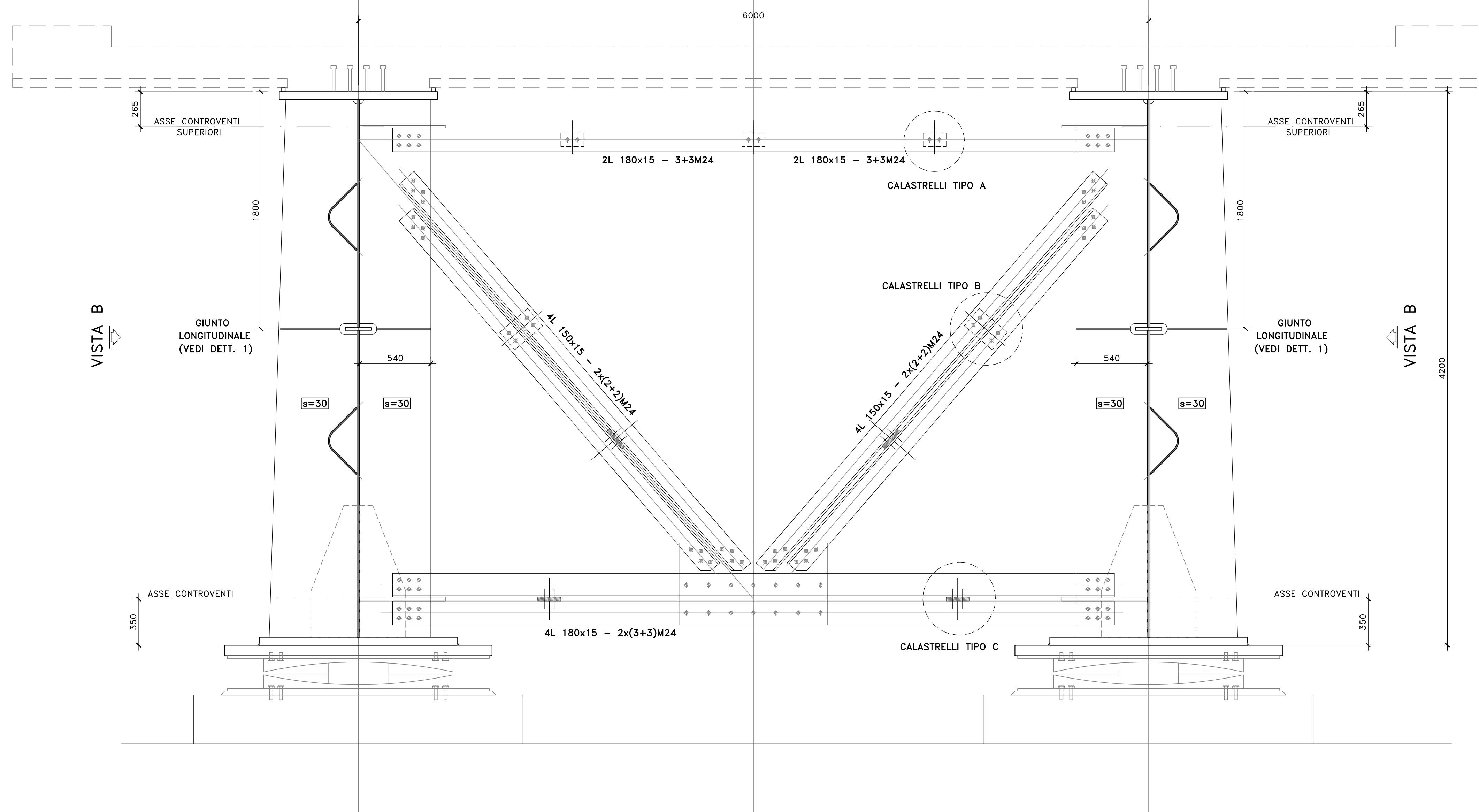
VISTA DIAFRAMMA (DP1) SCALA 1:20
