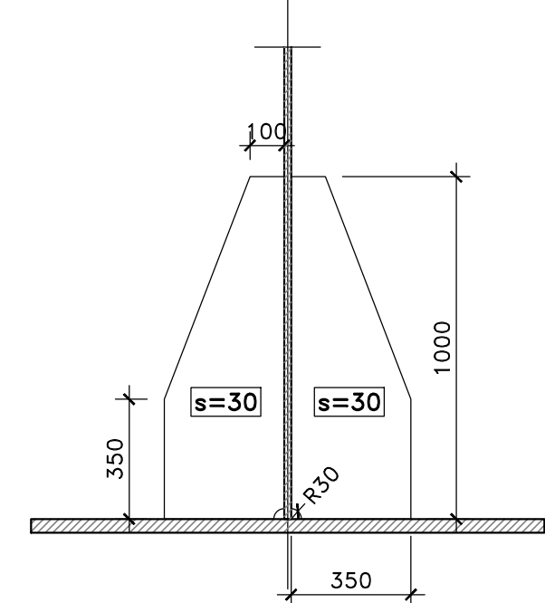
IRRIGIDIMENTI PER SOLLEVAMENTO SCALA 1:20
