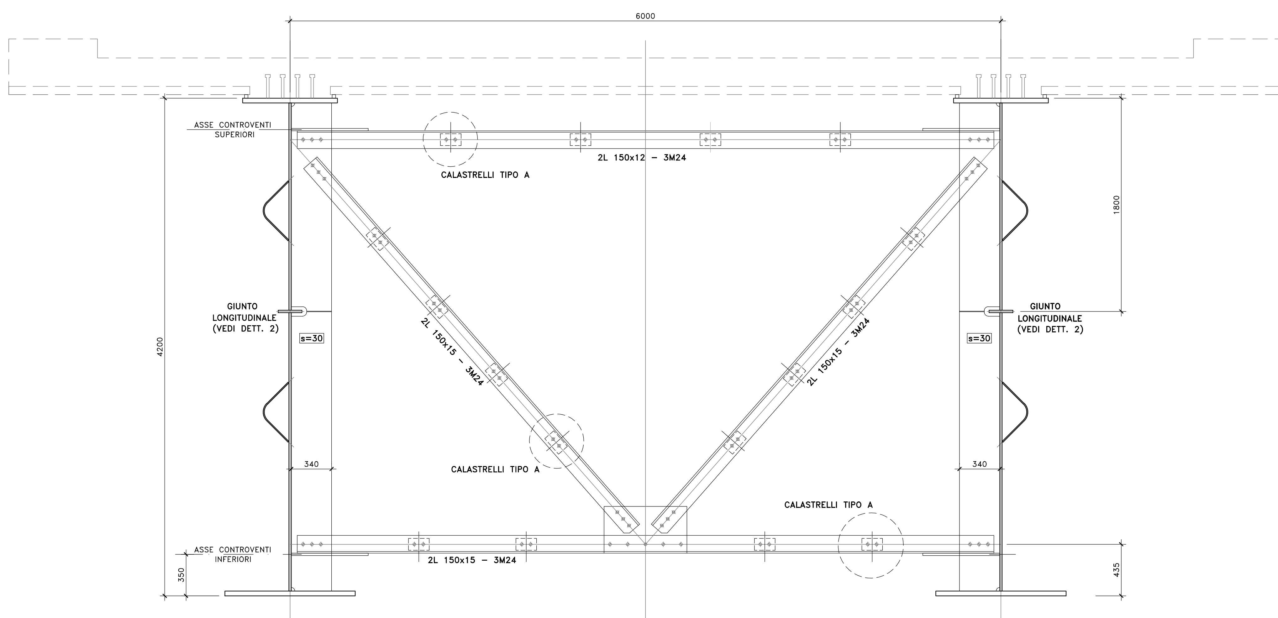
VISTA DIAFRAMMA (D11) SCALA 1:20
