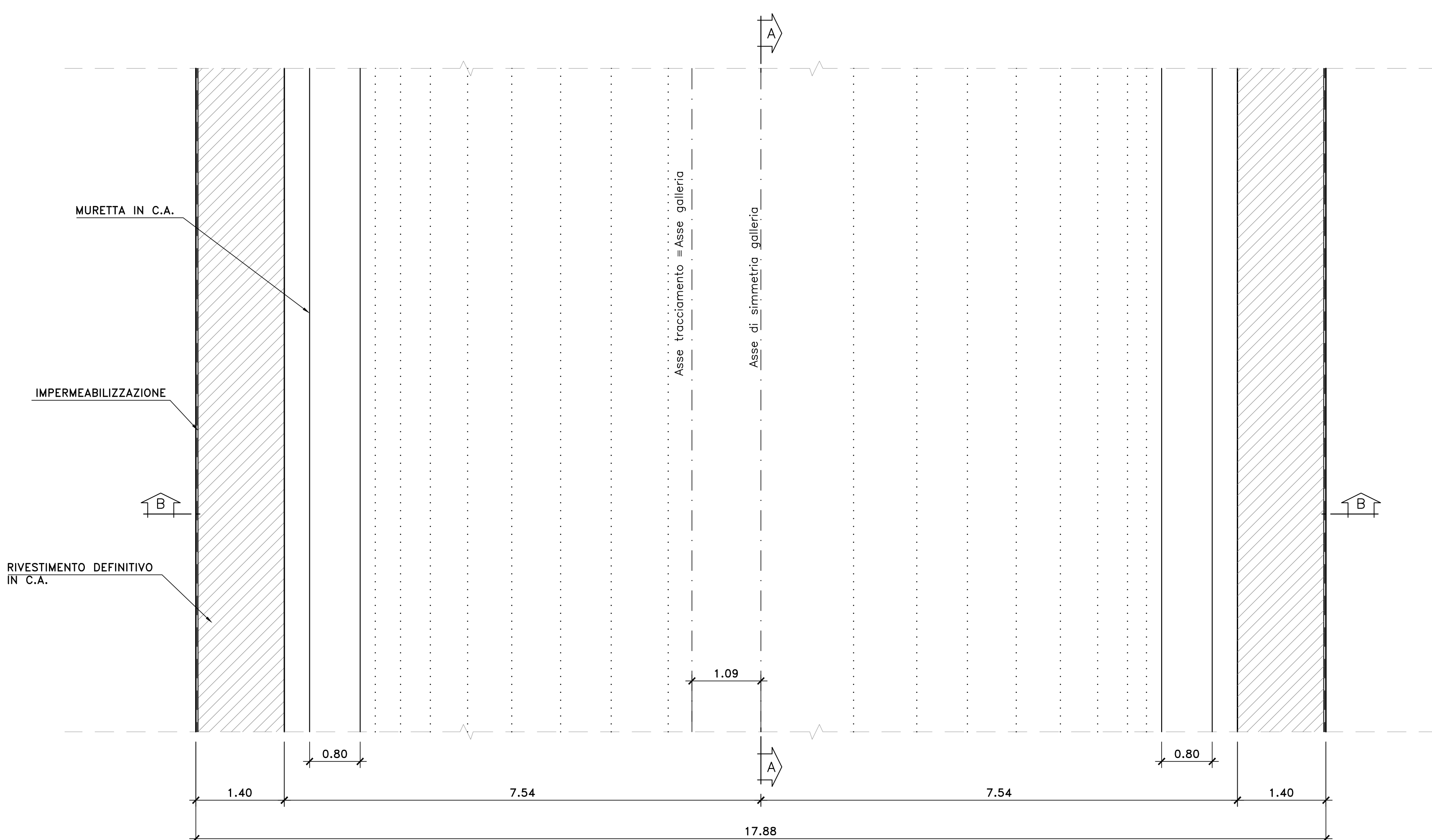
SEZIONE "C-C" PIANTA
