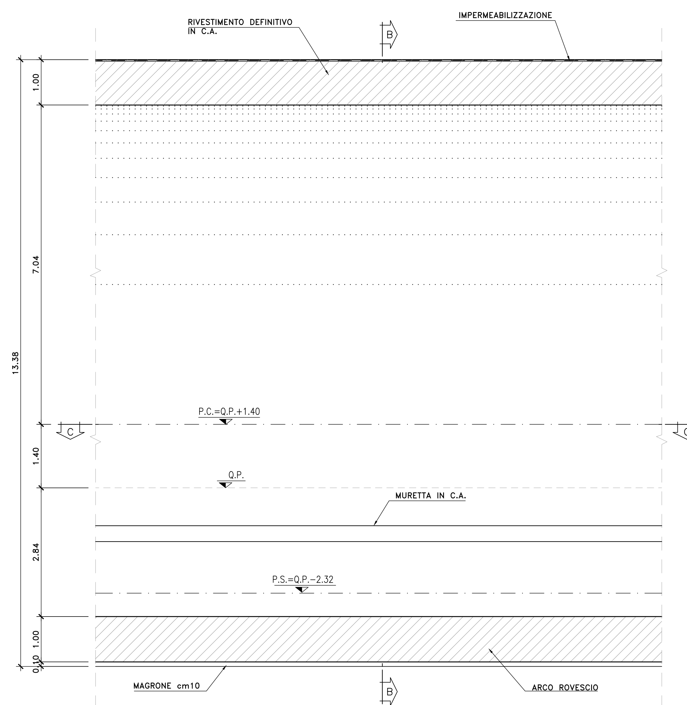
SEZIONE "A-A" PROFILO LONGITUDINALE
