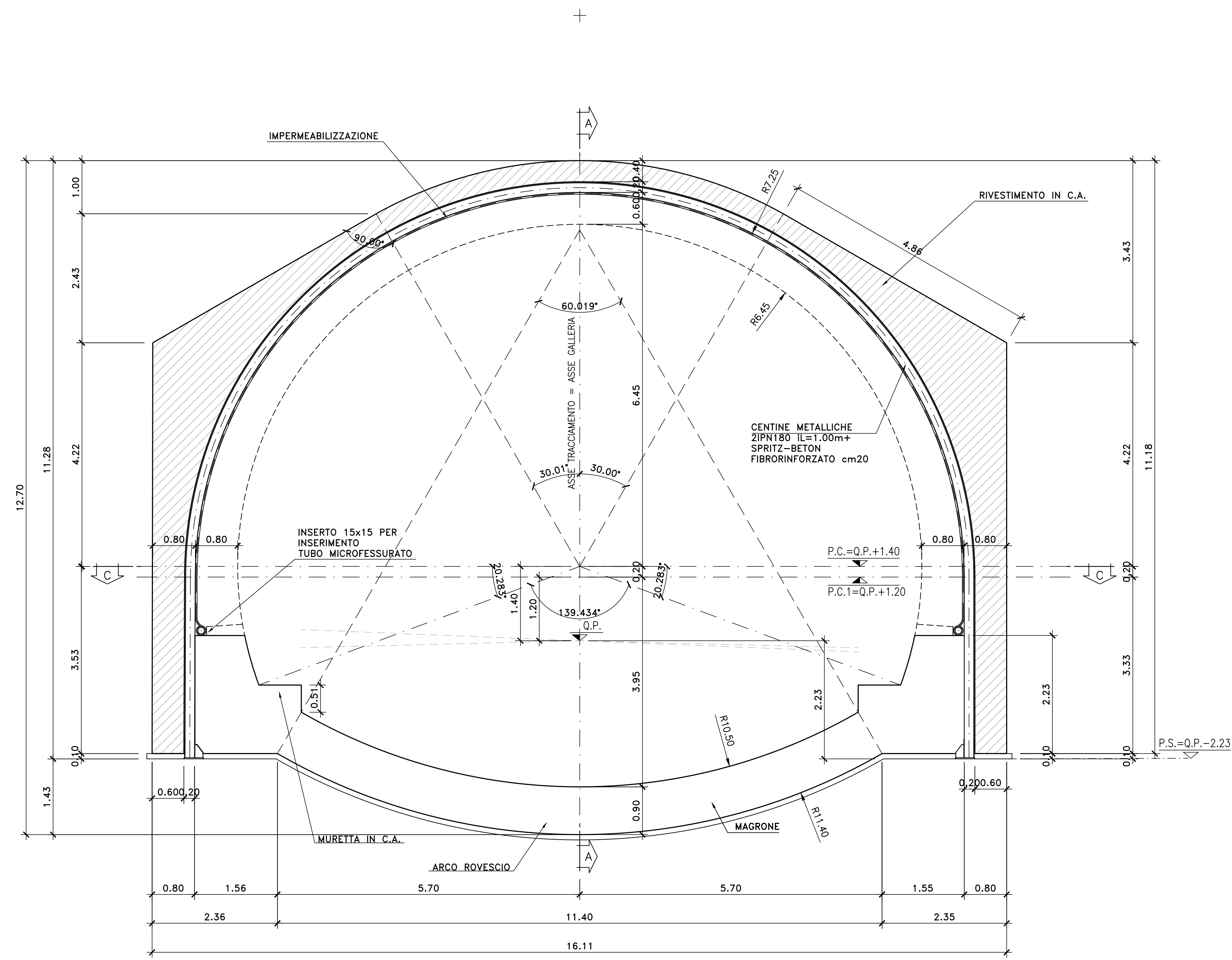
SEZIONE "B-B" SEZIONE TRASVERSALE Scala 1:50
