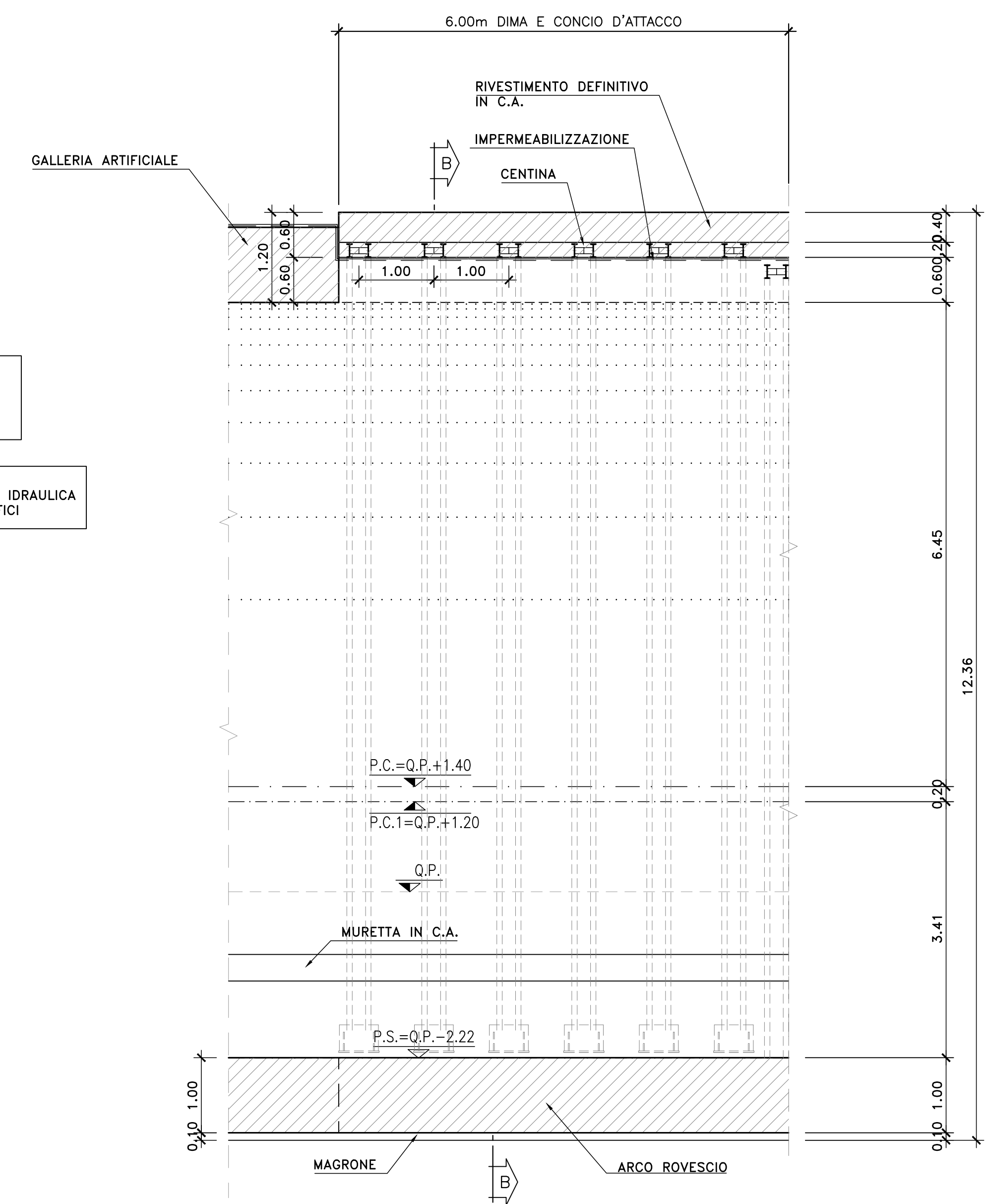
SEZIONE "A-A" PROFILO LONGITUDINALE Scala 1:50
