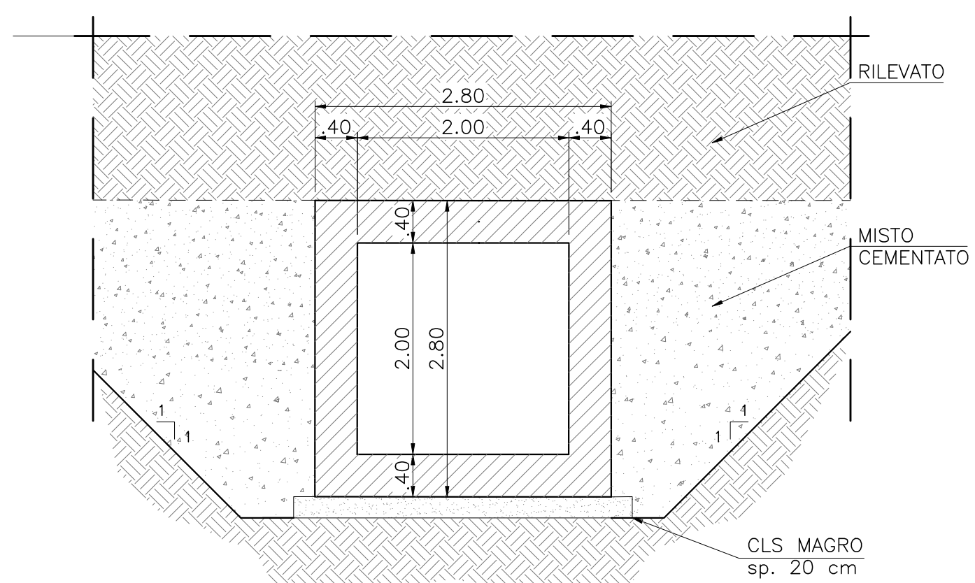
SEZIONE A-A TOMBINO IN C.A. 2.00x2.00 Scala 1:50
