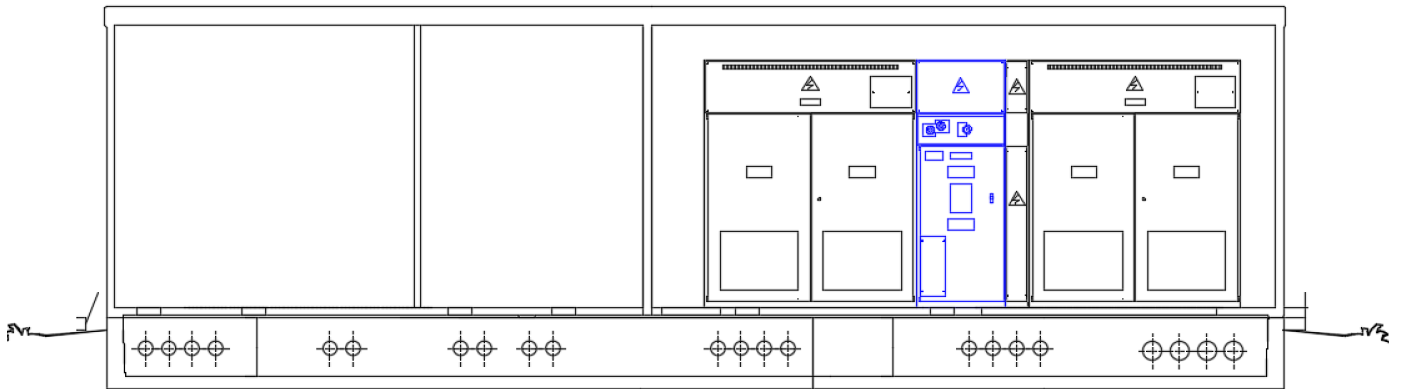
SEZIONE
