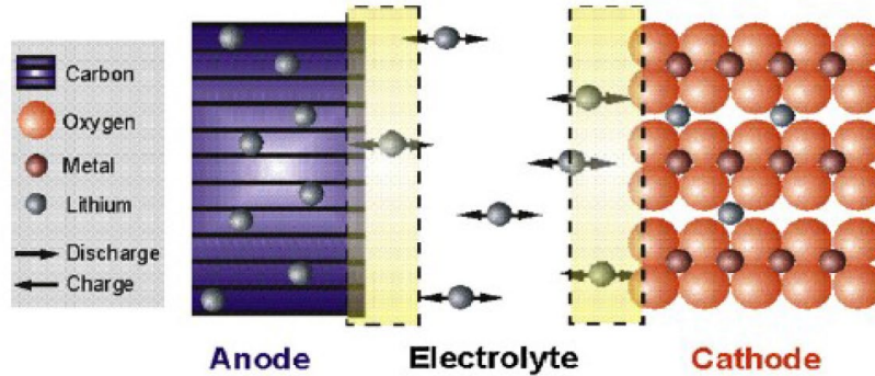
Figura 2. Reazioni chimiche per batteria Litio/Ioni
