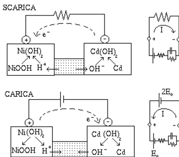
Figura 5: Struttura della batteria Nichel / Cadmio
