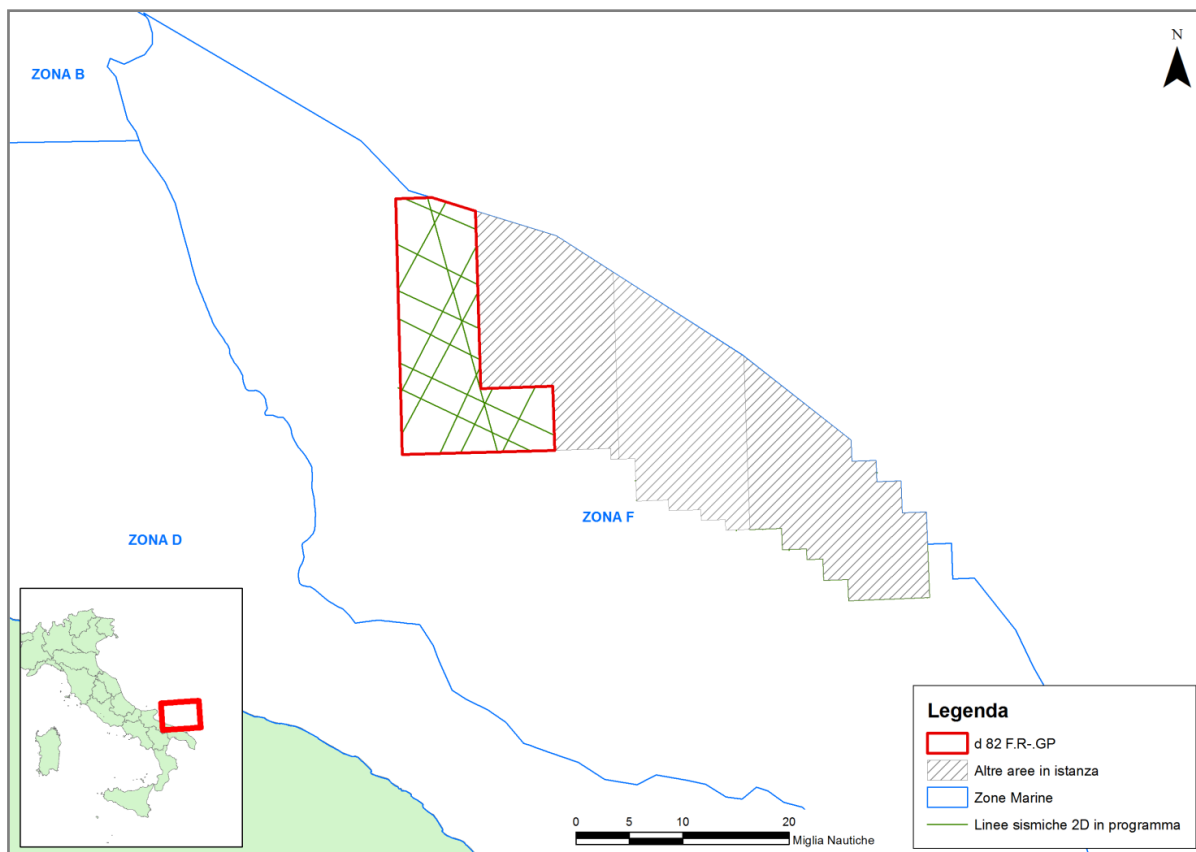
Figura 2.4 – Ubicazione delle linee sismiche 2D in progetto di acquisizione, all'interno del perimetro dell'istanza di permesso di ricerca idrocarburi "d 82 F.R.-GP".
