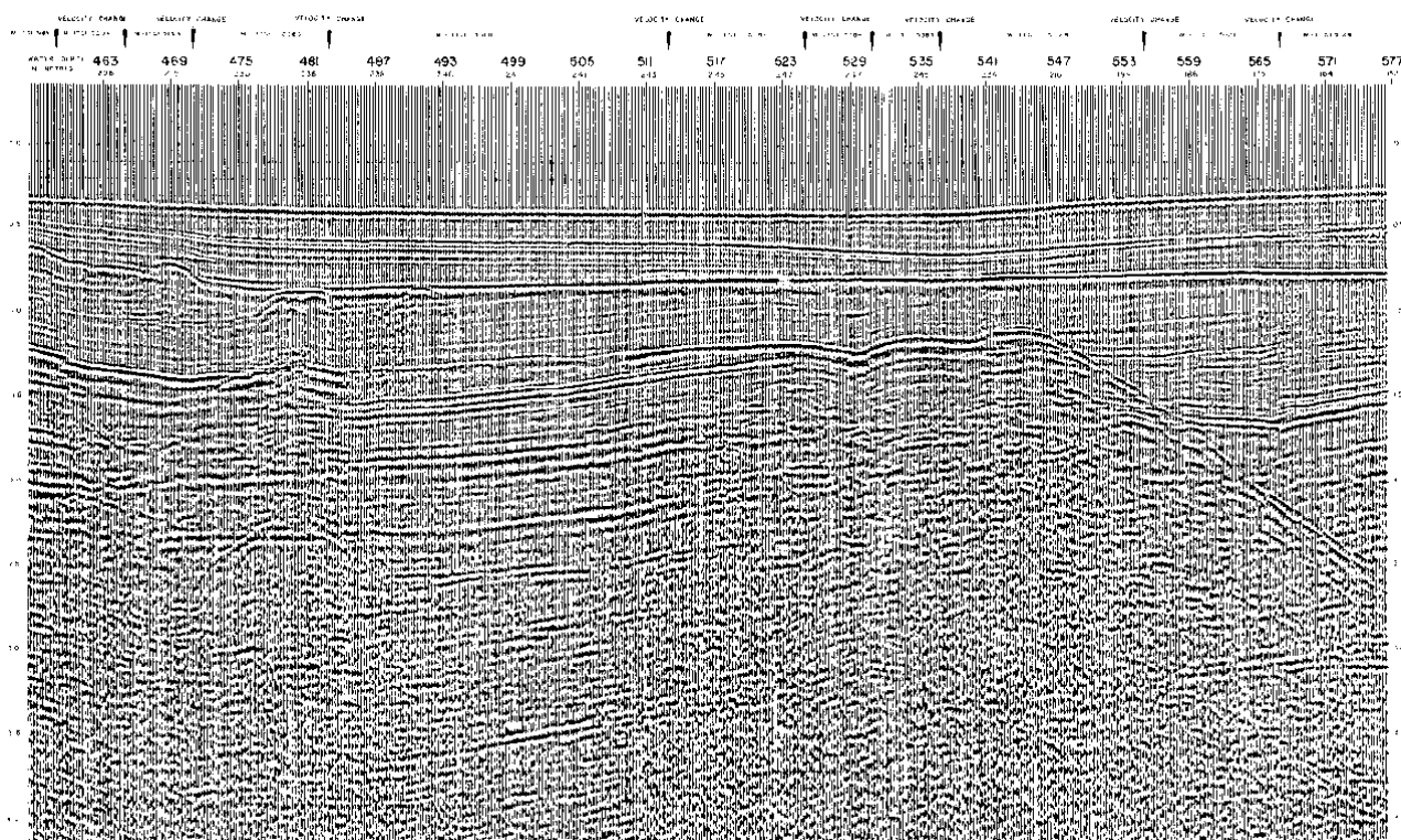
Figura 3.24 – Esempio di sezione sismica non interpretata (fonte: www.unmig.sviluppoeconomico.gov.it/videpi , modificata).
