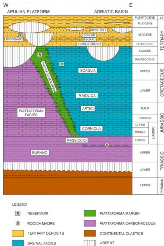
Figura 4.10 – Stratigrafia generale della piattaforma Apula e del bacino Ionico-Albanese (fonte: unmig.sviluppoeconomico.gov.it/vidempi ).
