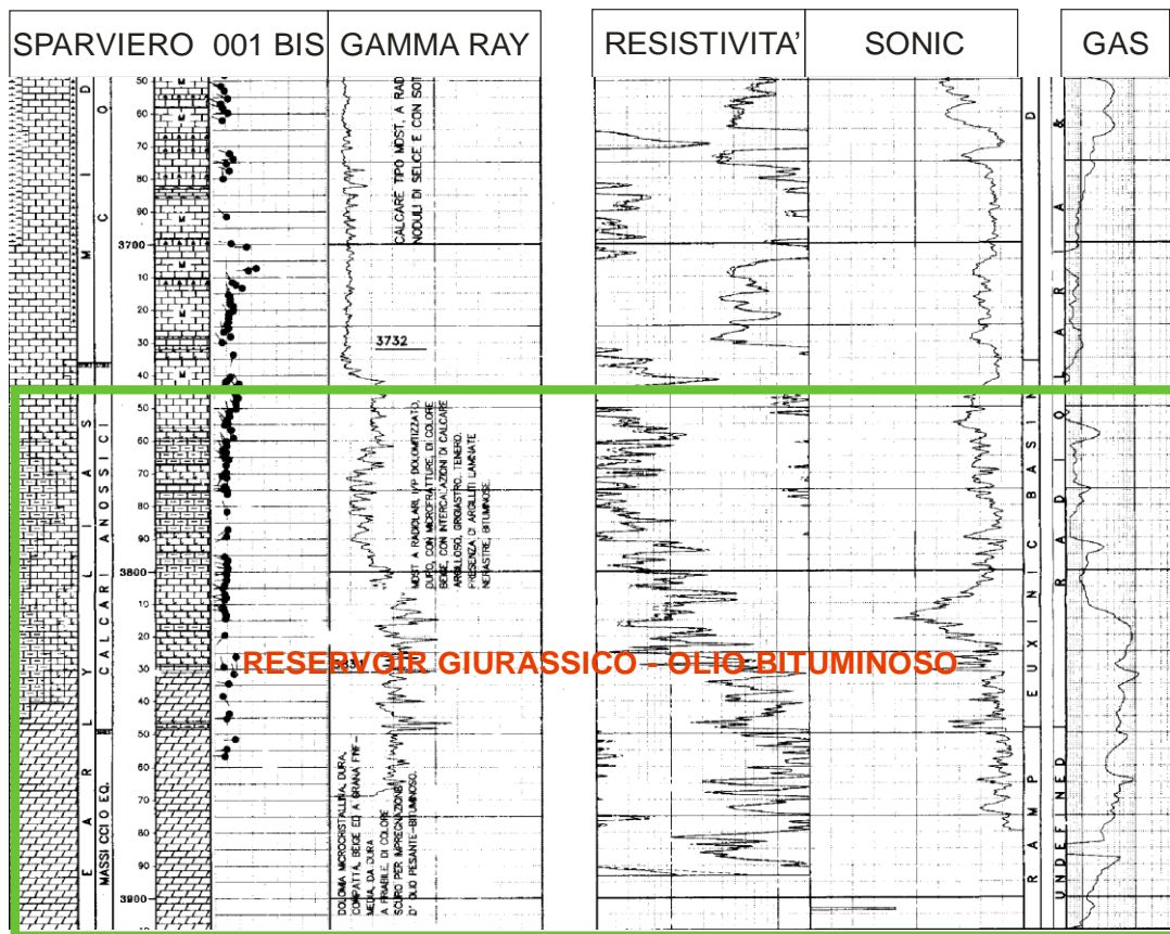
Figura 3.7 – Estratto del composite log del pozzo Sparviero 001 bis con evidenziato il target giurassico raggiunto a fondo pozzo dalla perforazione (fonte: www.unmig.sviluppoeconomico.gov.it/videpi , modificata).
