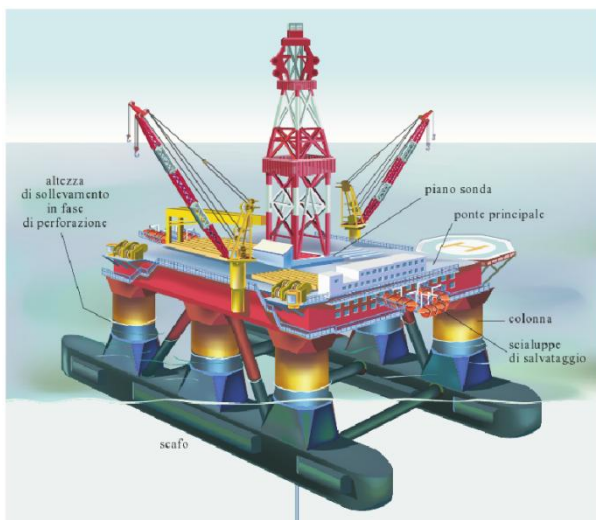
Figura 3.27 – Schema di un impianto di perforazione semisommersibile, a sinistra (fonte: Treccani, 2009) e immagine di una piattaforma semisub in navigazione, a destra (fonte: www.worldmaritimeneews.com ).
