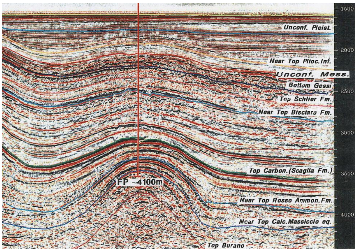
Figura 3.8 - Struttura intercettata dal pozzo Sparviero 1 bis (fonte: unmig.sviluppoeconomico.gov.it/videpi/ ).
