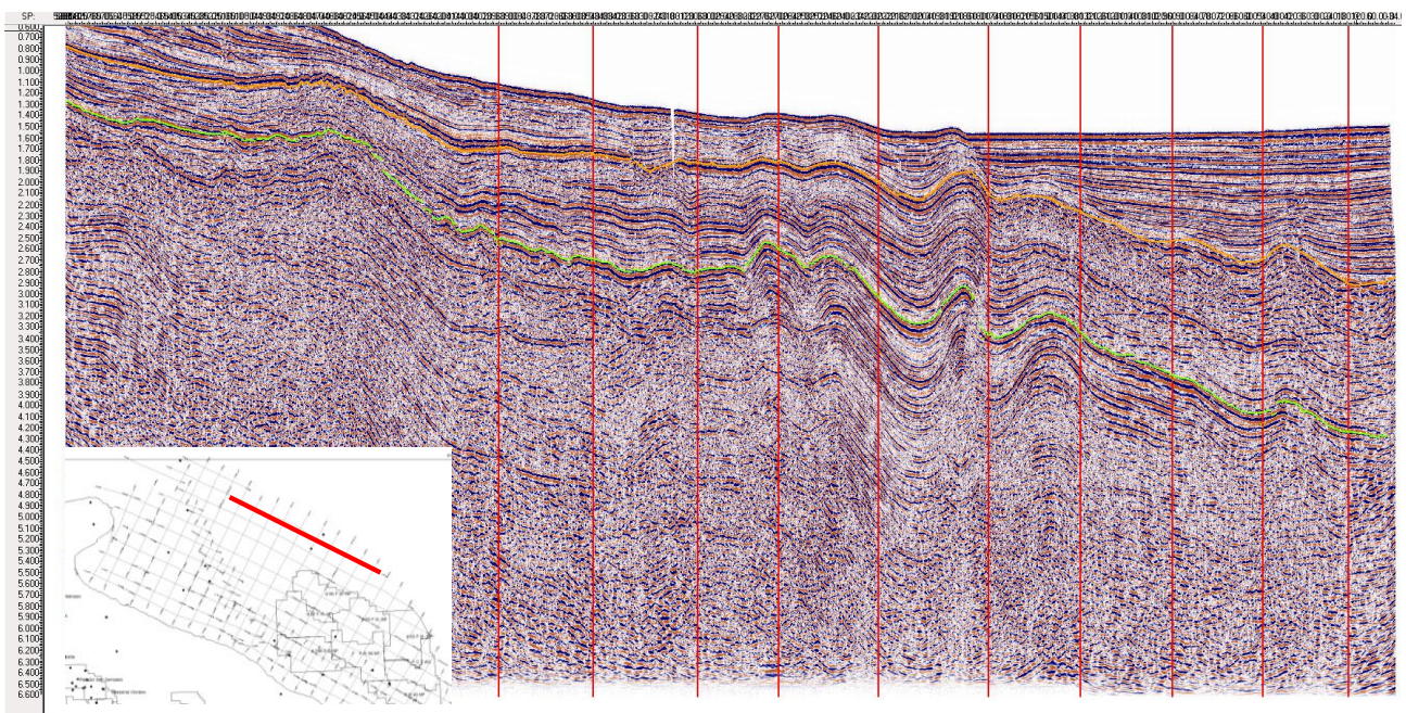
Figura 4.12 – Sezione sismica lungo la linea evidenziata in rosso nel quadrante in basso a sinistra (fonte dei dati: unmig.sviluppoeconomico.gov.it/videpi ).
