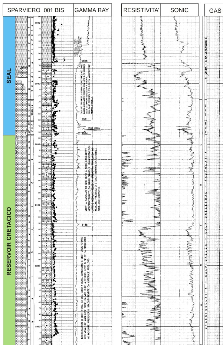
Figura 3.11 – Composite log del pozzo Sparviero 001bis dove si osserva la duplice presenza della roccia di copertura rappresentata dalle Marne a Fucoidi e/o Scaglia Cinrea (fonte: www.unmig.sviluppoeconomico.gov.it/videpi , modificata).
