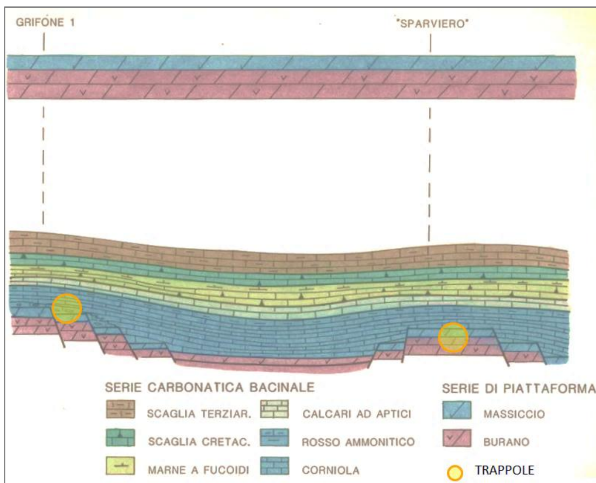
Figura 3.17 – Esempio di possibili trappole presenti nella zona di interesse (fonte: unmig.sviluppoeconomico.gov.it/videpi , modificata).
