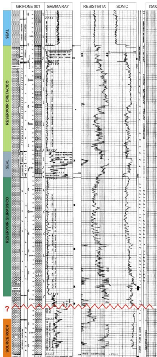
Figura 3.5 – Pozzo Grifone 001 ubicato all'interno dell'area di interesse. Lungo il composite log sono stati evidenziati i possibili sistemi (fonte: www.unmig.sviluppoeconomico.gov.it/vidempi , modificata).
