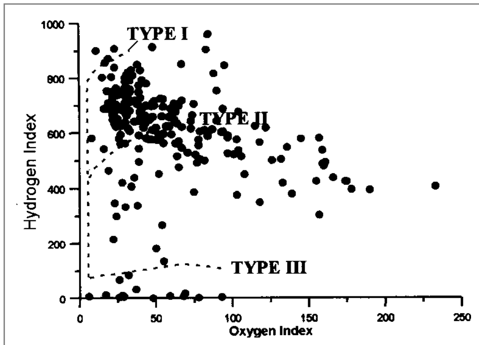
Figura 3.12 – I valori di TOC variano da 0.1 a 0.6%, con picchi di 1.5%, con un contenuto di idrogeno superior ai 600 mg HC /g TOC (Paulucci et al. 1988). La material organica sembra essere di origine marina con kerogene di tipo II (fonte: Paulucci et al. 1988).
