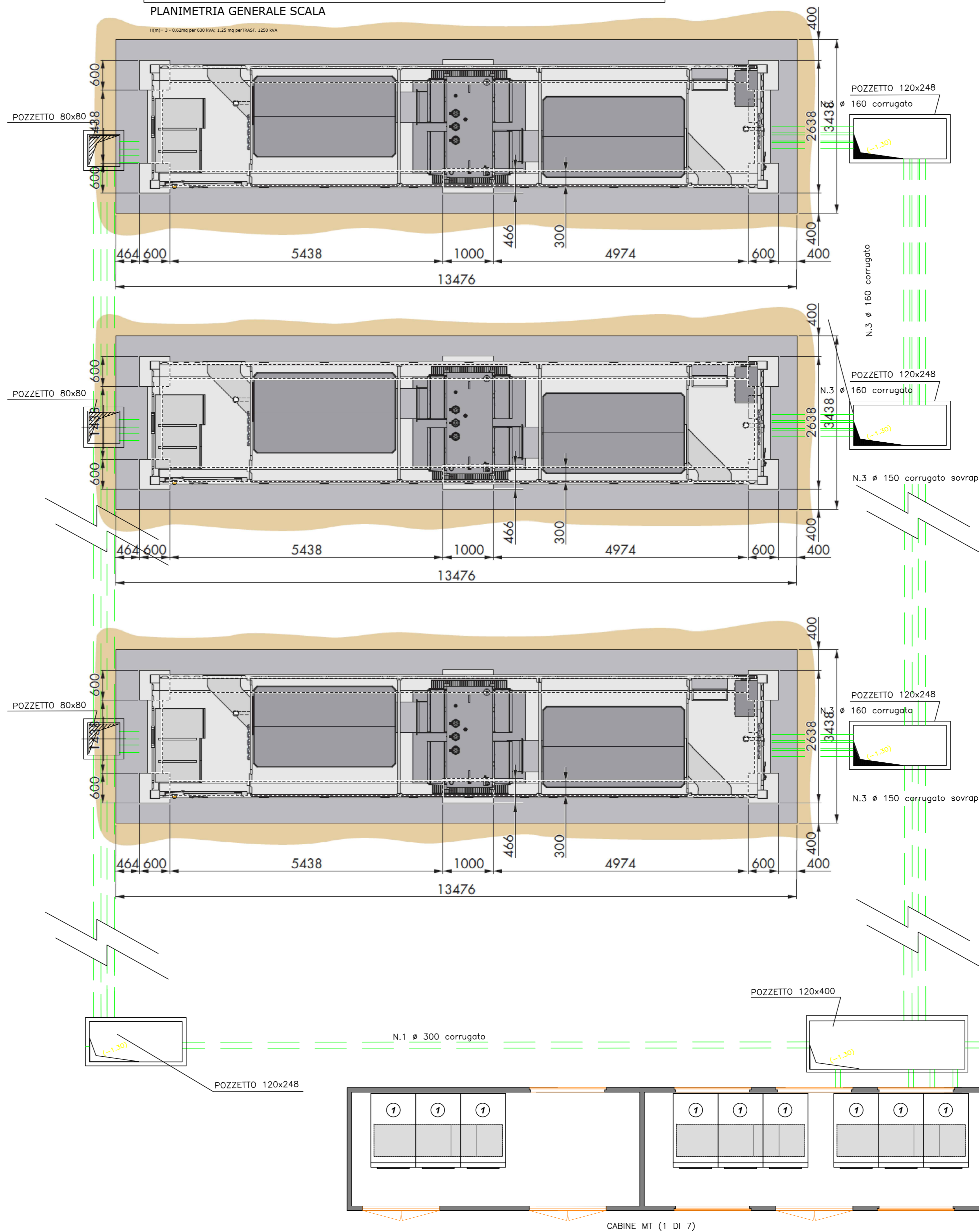
CABINA INVERTER Scala 1:50
