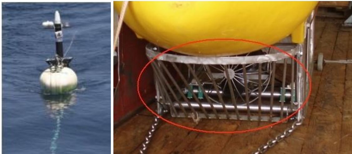
Figura 6.1 – A sinistra: esempio di boa di coda, fissata all’estremità del cavo sismico. A destra: dispositivo che esclude la possibilità di intrappolamento delle tartarughe marine (fonte: www.ketosecology.co.uk )
