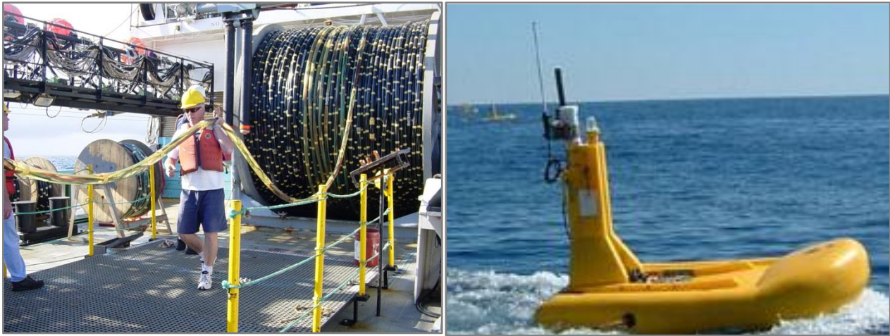
Figura 3.24 – Streamer o cavo sismico per l’acquisizione a sinistra (fonte: www.ig.utexas.edu ) e Boa di coda a destra (fonte: www.seamap.com ).
