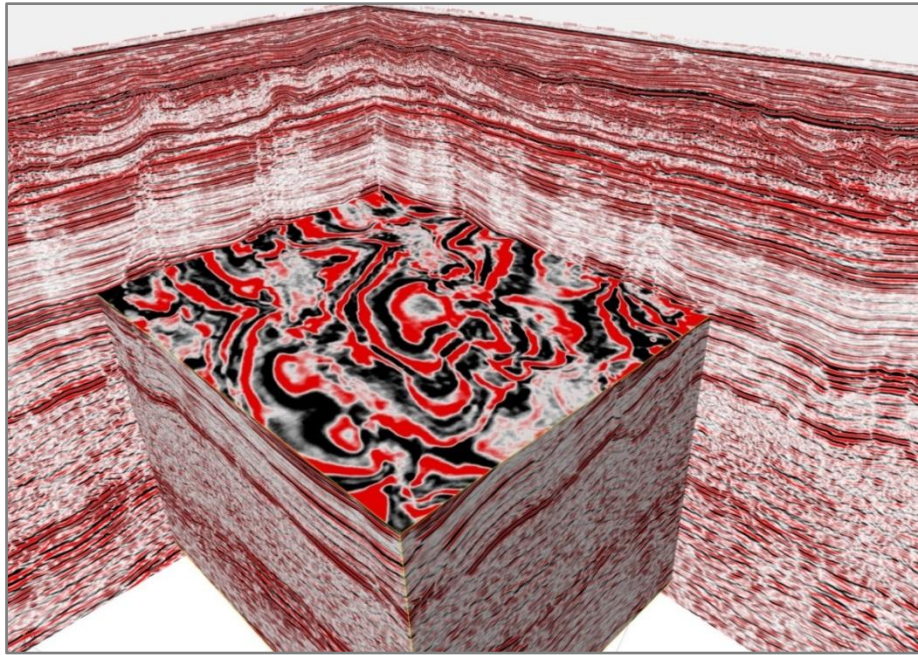
Figura 3.27 – Esempio di modello 3D ottenuto dall’elaborazione di un’acquisizione 3D (fonte: www.spectrumasa.com )
