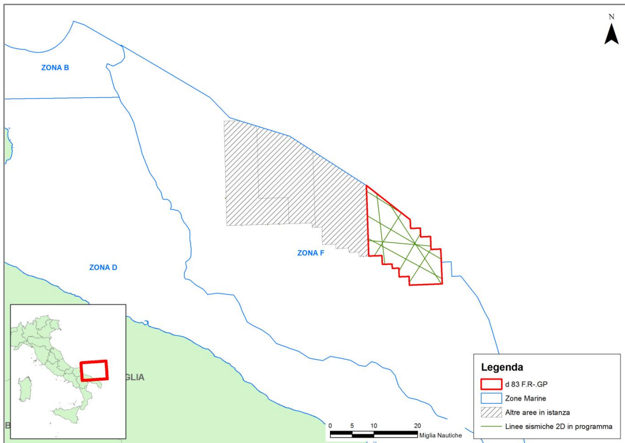
Figura 3.20 – Ubicazione delle linee sismiche 2D in progetto di acquisizione, all'interno del perimetro dell'istanza di permesso di ricerca idrocarburi "d 83 F.R.-GP"
