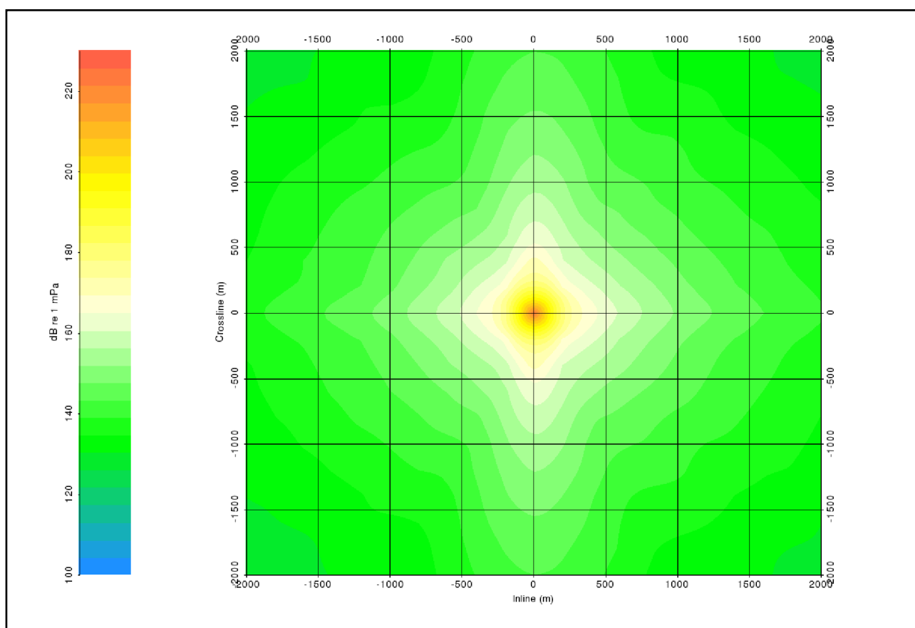
Figura 5.2 - Livelli attesi del segnale acustico generato dall'array di air-gun nella "configurazione array 2" (paragrafo 3.5.2), ad una profondità di 10 metri e per un raggio di 2 chilometri dalla sorgente
