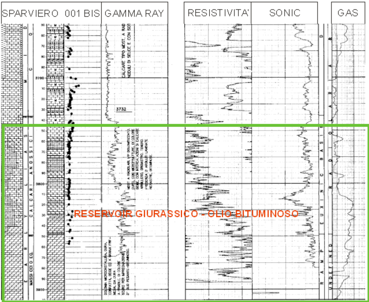
Figura 3.9 – Estratto del composite log del pozzo Sparviero 001 bis con evidenziato il target giurassico raggiunto a fondo pozzo dalla perforazione (fonte: unmig.sviluppoeconomico.gov.it/vidapi )
