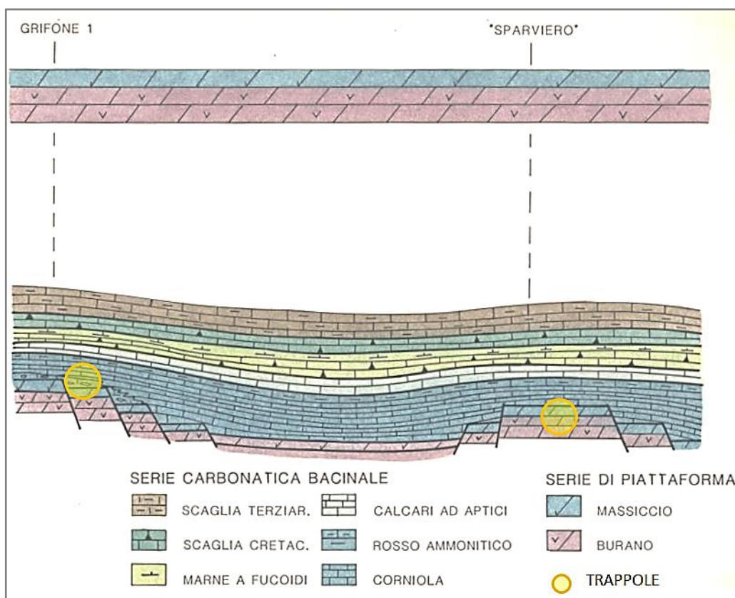
Figura 3.19 – Esempio di possibili trappole presenti nella zona di interesse (fonte: unmig.sviluppoeconomico.gov.it/vidempi, modificata)
