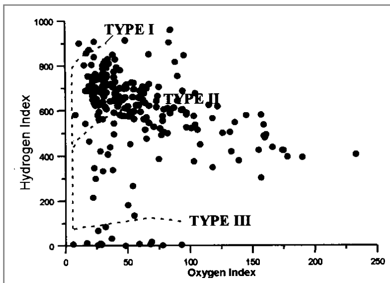
Figura 3.14 – I valori di TOC variano da 0.1 a 0.6%, con picchi di 1.5%, con un contenuto di idrogeno superiore ai 600 mg HC/g TOC (Paulucci et al. 1988). La materia organica sembra essere di origine marina con kerogene di tipo II (fonte: Paulucci et al. 1988).
