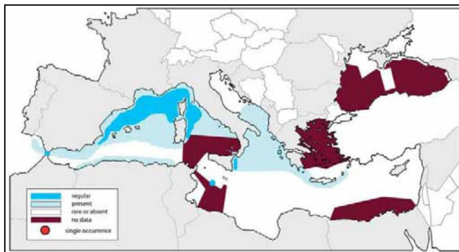
Figura 4.37 - Distribuzione della Balenottera Comune nel Mediterraneo (fonte: Notarbartolo di Sciara & Birkun, 2010)
