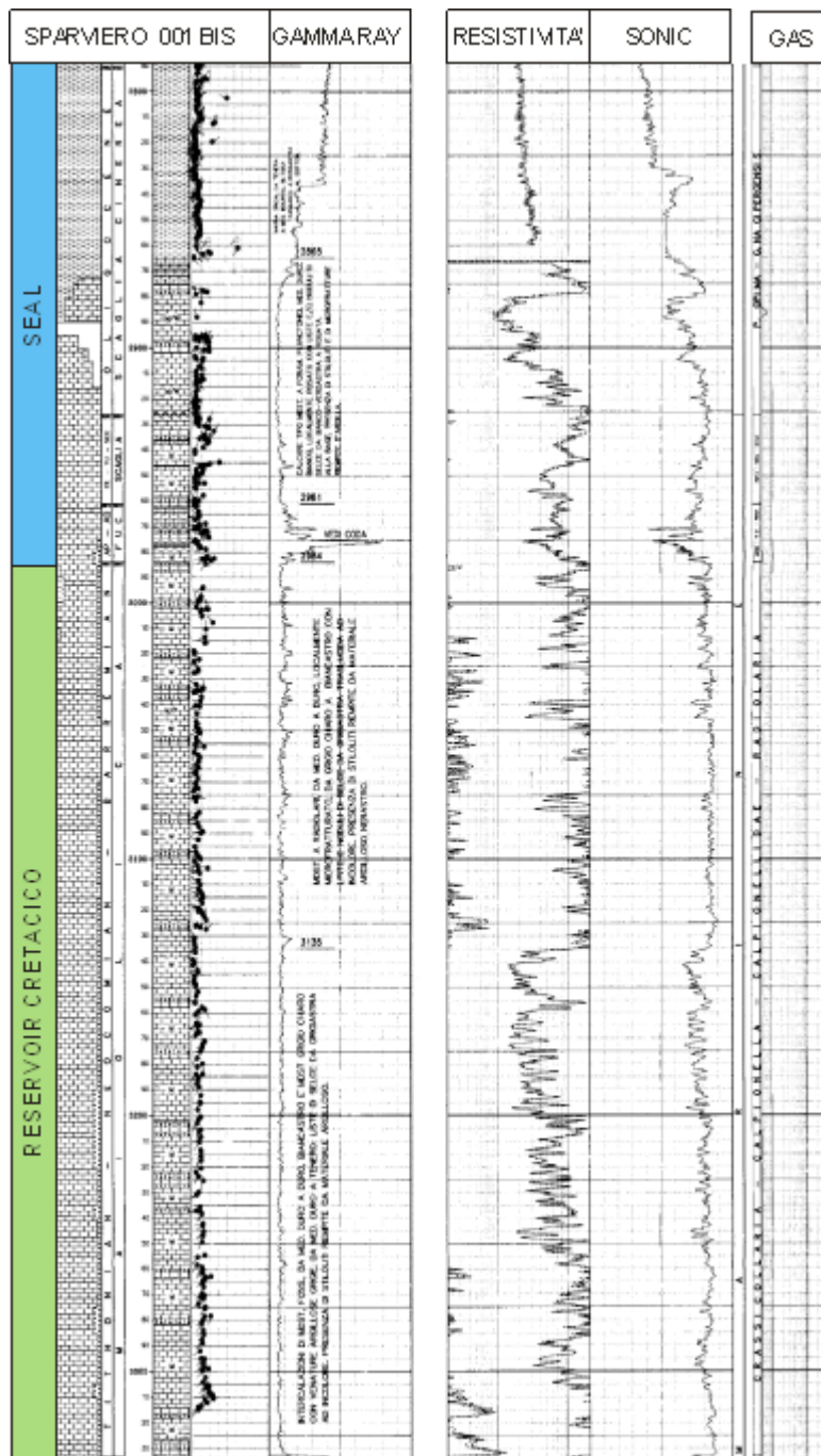
Figura 3.13 – Composite log del pozzo Sparviero 001bis dove si osserva la duplice presenza della roccia di copertura rappresentata dalle Marne a Fucoidi e/o Scaglia Cinerea (fonte: www.unmig.sviluppoeconomico.gov.it/videpi , modificata).
