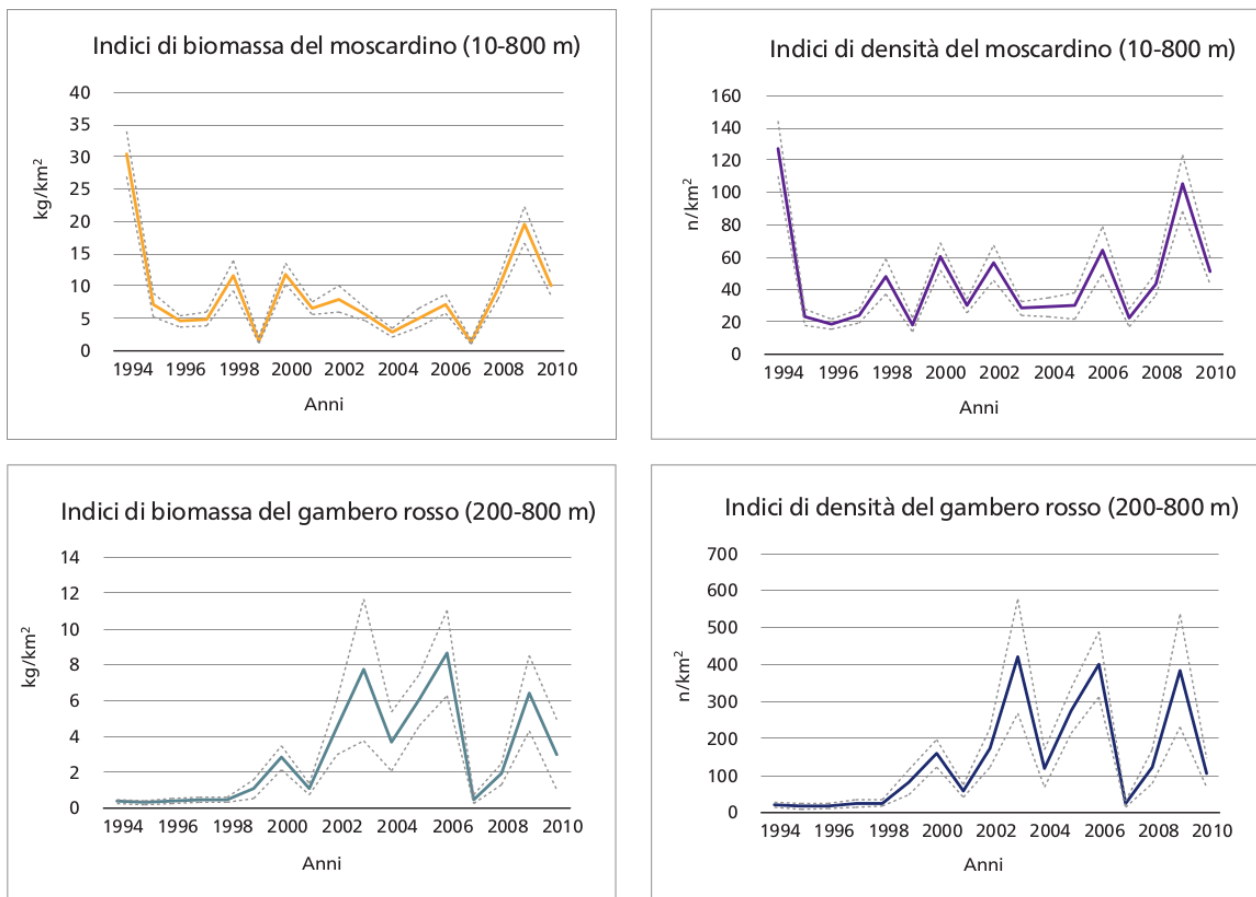
Figura 4.69 - Indici di biomassa ( \text{kg}/\text{km}^2 ) e di densità ( \text{n}/\text{km}^2 ) e relativi limiti di confidenza (linee tratteggiate) delle principali specie bersaglio stimati sul loro areale di distribuzione, (fonte: Dati MEDITS 1994-2010, tratti da "Lo stato della pesca e dell'acquacoltura nei mari Italiani" – Capitolo 2).
