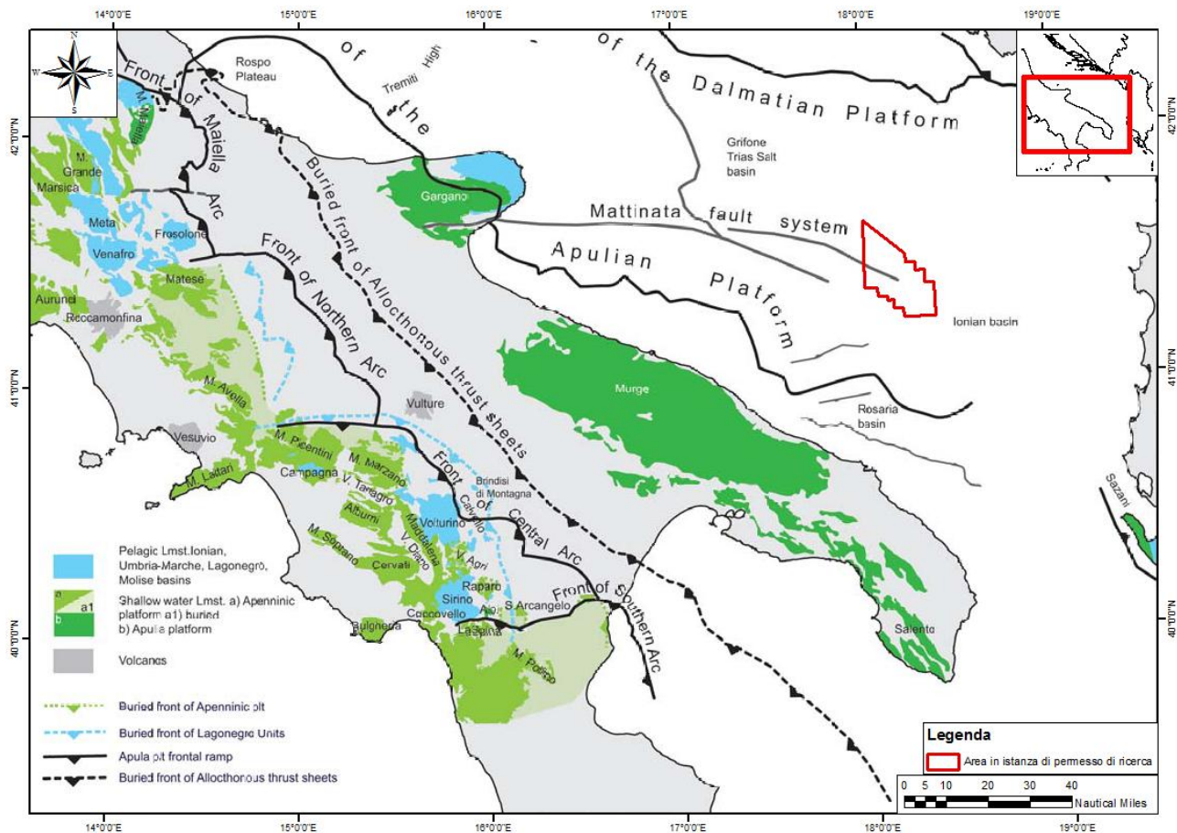
Figura 4.11 – Principali affioramenti di carbonati mesozoici (sopra) e principali lineamenti strutturali al top carbonati. All'interno della catena sono localizzati quattro settori principali che da nord verso sud sono la Majella, l'arco settentrionale, l'arco centrale e l'arco meridionale. Nell'avampaese viene indicata la forma del margine della piattaforma composta da tratti NW-SE collegati da zone ad andamento W-E. Sono visibili anche l'Alto Centro-Adriatico, il sistema della Faglia di Mattinata (MFS), l'area a pieghe di Grifone e il bacino di Rosaria Mare (fonte: Nicolai e Gambini, 2007, modificata).
