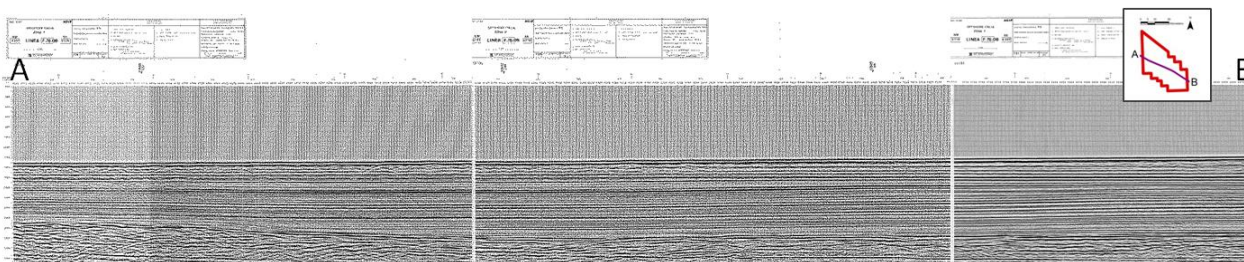
Figura 4.3 – Profilo sismico della linea F76-06 (parti 9-10-11) in corrispondenza dell'area in istanza, orientata lungo la direzione NO-SE. Il margine superiore del riquadro grigio è il livello del mare, mentre le linee scure indicano gli strati geologici nel sottosuolo, di cui la parte sommitale rappresenta il fondale marino
