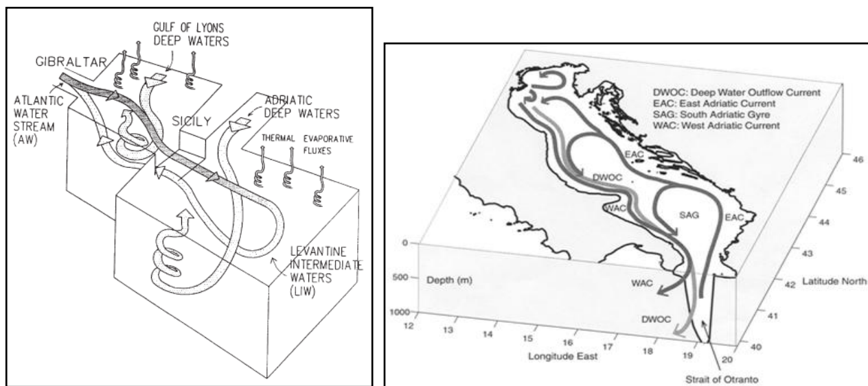
Figura 4.30 – A sinistra: rappresentazione schematica della circolazione termalina nel Mediterraneo (fonte: Lascaratos, 1999). A destra: circolazione schematica nell'Adriatico (fonte: www.devotes-project.eu/adriatic-sea )
