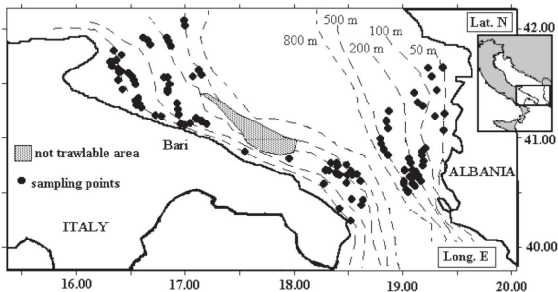
Figura 4.71 – Stazioni di campionamento come riportate dallo studio di Ungaro (fonte: Ungaro et al., 2005)
