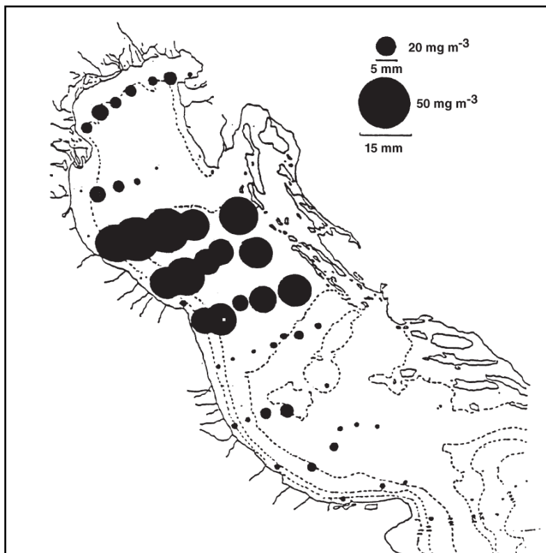
Figura 4.34 – Distribuzione geografica della biomassa netta di zooplancton nel mar Adriatico. (figura tratta da Fonda Umani 1996, come riportata da Fonda Umani 1994).
