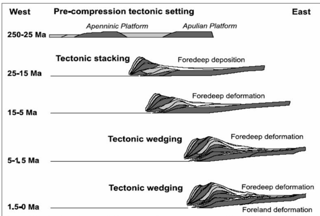
Figura 4.9 - Cinematica semplificata dell'Appennino Meridionale con la migrazione da ovest verso est delle unità appartenenti alla Catena, Avanfossa (o Foredeep) e Avampaese (o Foreland) (fonte: Turrini et al. 2004)
