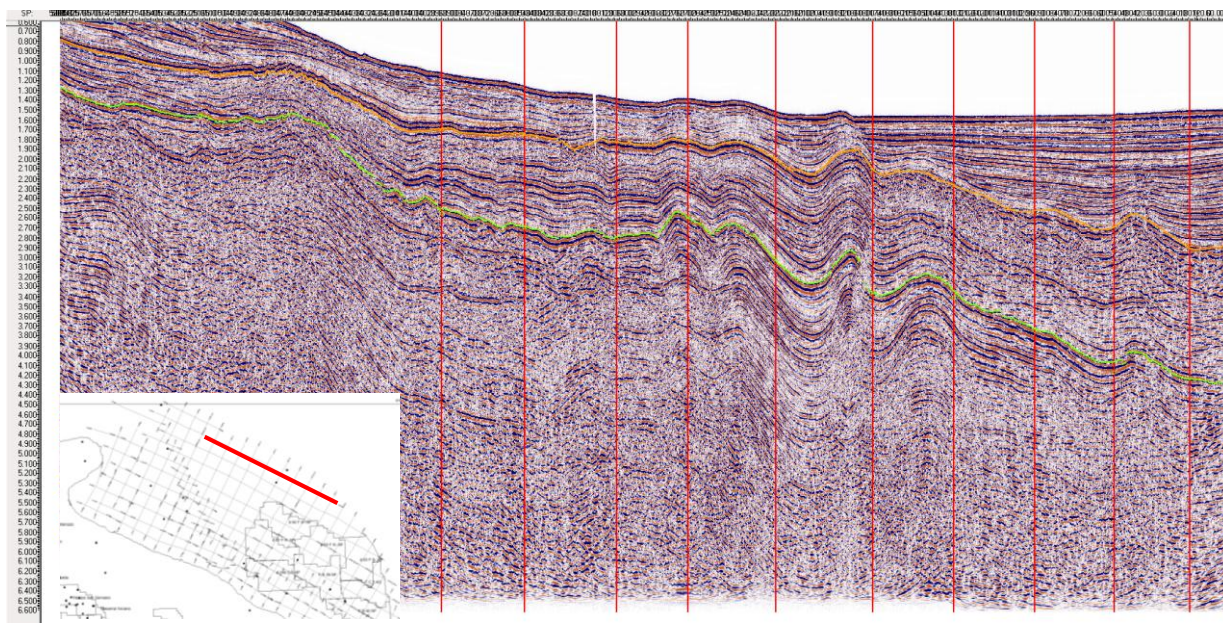
Figura 4.12 – Sezione sismica lungo la linea evidenziata in rosso nel quadrante in basso a sinistra (fonte dei dati: unmig.sviluppoeconomico.gov.it/videpi )
