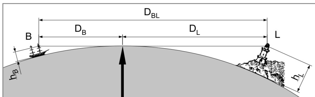
Figura 5.5 – Distanza geometrica dell'orizzonte
