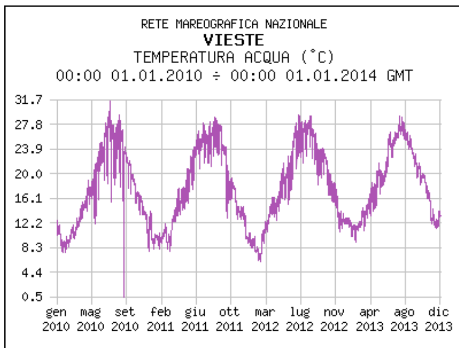
Figura 4.14 – Temperatura dell'acqua nella stazione di Vieste periodo 2010 – 2014 (fonte: www.mareografico.it ).
