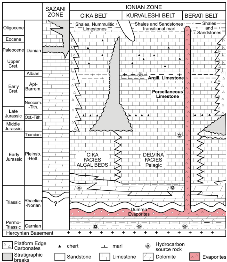
Figura 3.16 – Successione del Bacino Ionico in Albania rispetto alle unità tettoniche limitrofe. Le aree di Cika e Berati possono essere confrontate con la parte centrale del Bacino Adriatico (fonte: Velaj et al., 1999).
