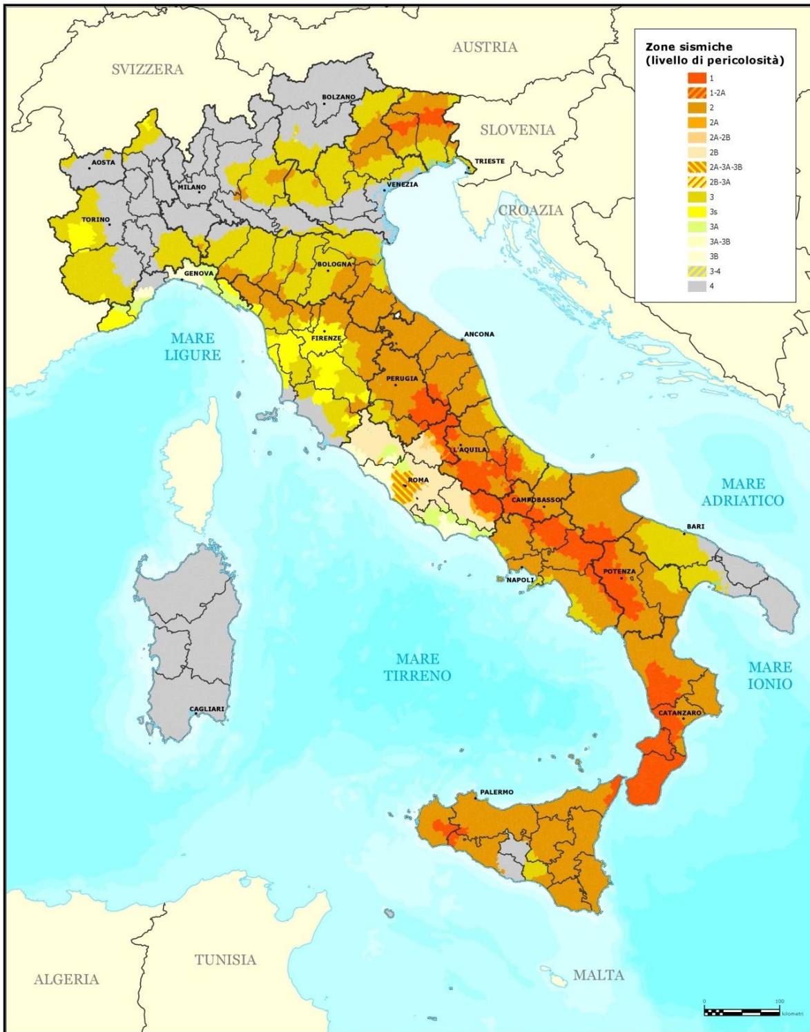
Figura 2.17 - Classificazione sismica del territorio italiano aggiornata al 2012 (fonte: www.protezionecivile.gov.it/resources/cms/documents/A3_class2012_03prov_.pdf )
