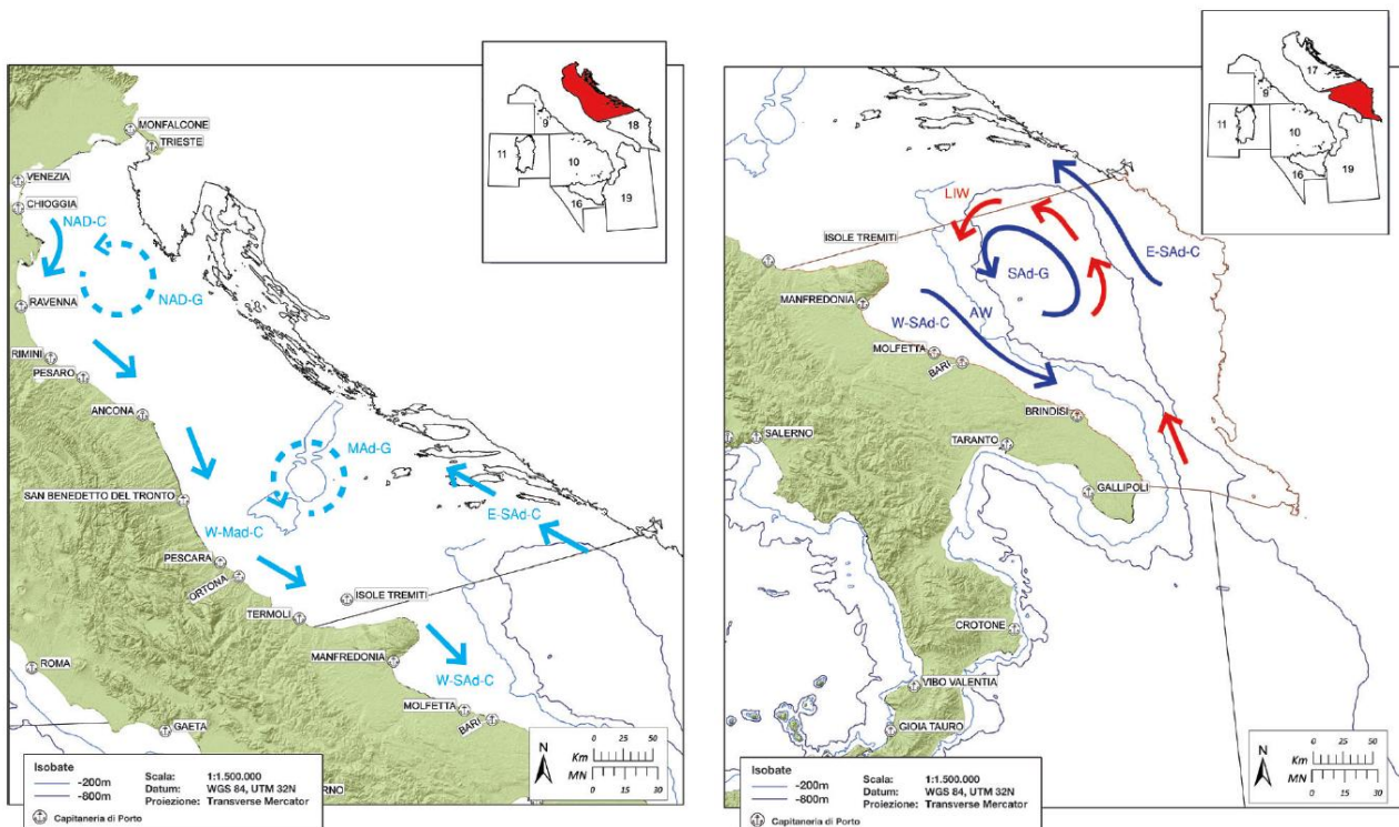
Figura 4.32 – Circolazione dell'Adriatico Settentrionale (GSA17, a sinistra) e dell'Adriatico Meridionale (GSA18, a destra). NAd-C: corrente adriatica settentrionale; NAd-G: vortice nord adriatico (autunno); W-MAd-C: corrente adriatica centro-occidentale (primavera, estate e autunno); MAd-G: vortice Medio Adriatico (primavera, estate, autunno); W-SAd-C: corrente adriatica sud-occidentale (primavera, estate, autunno); E-SAd-C: corrente adriatica sudorientale (autunno, primavera, inverno). AW: acque di derivazione atlantica superficiali modificate; LIW: acque intermedie levantine; SAd-G: vortice del Sud Adriatico; E-SAd-C: corrente adriatica nordorientale; W-SAd-C: corrente adriatica sudoccidentale. (fonte: "Lo stato della pesca e dell'acquacoltura nei mari italiani", 2011)
