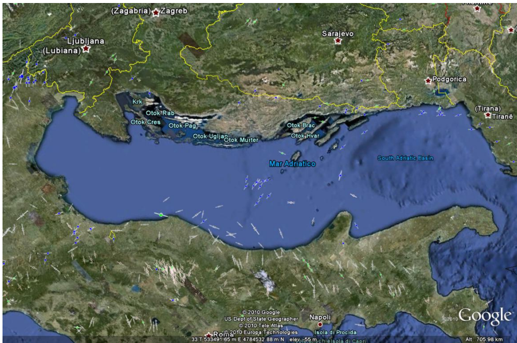
Figura 4.6 – Direzione degli stress basata sulla mappa degli stress globali (fonte: Heidbach et al., 2008)
