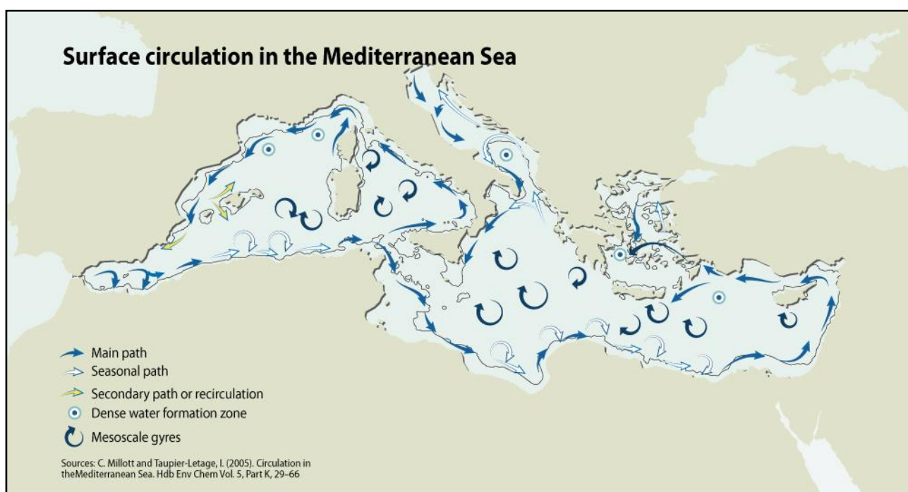
Figura 4.29 – Circolazione superficiale schematica nel Mar Mediterraneo (fonte: State of the Mediterranean marine and coastal environment, 2012 – modificato da Millot e Taupier-Letage, 2005)
