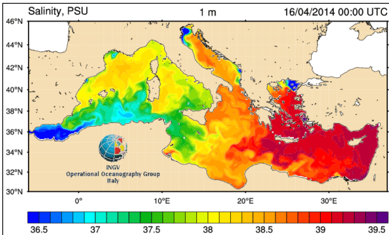
Figura 4.24 - Salinità espressa in psu delle acque superficiali nel Mar Mediterraneo, in data 16/04/2014 (fonte: gnoo.bo.ingv.it/mfs/myocean/bulletin.html?mode=analysis )
