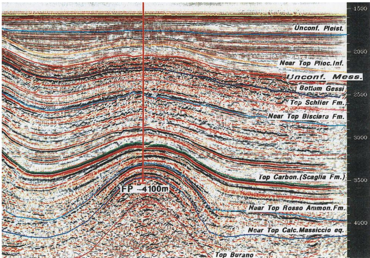
Figura 3.10 – Struttura intercettata dal pozzo Sparviero 1 bis (fonte: unmig.sviluppoeconomico.gov.it/videpi )
