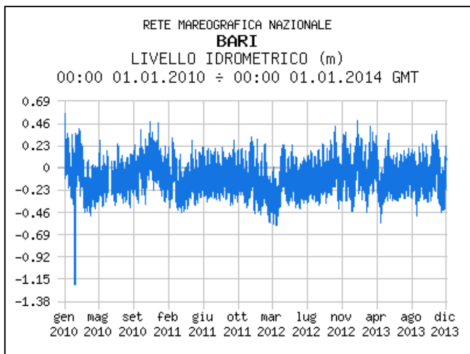
Figura 4.21 - Livello idrometrico nella stazione mareografica di Bari periodo 2010 – 2014 (fonte: www.mareografico.it )
