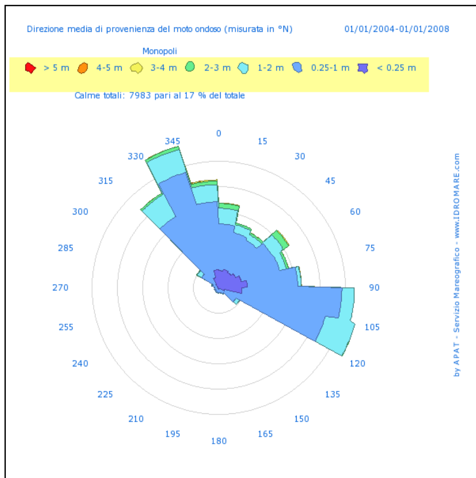
Figura 4.23 - Grafico del moto ondoso nella boa ondometrica di Monopoli (fonte dei dati: www.idromare.it ).
