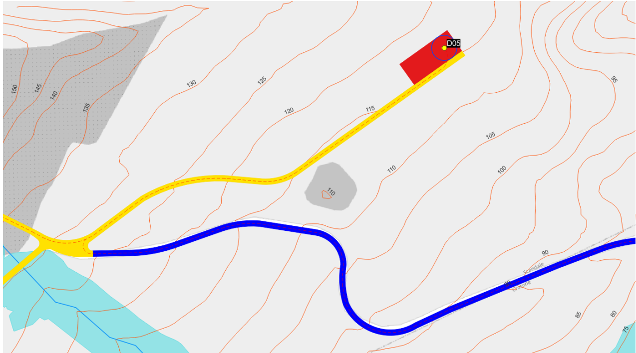
Figura 6-8 – Inquadramento D05 rispetto ai corsi d'acqua e alle aree di attenzione del PGRA con curve di livello.
