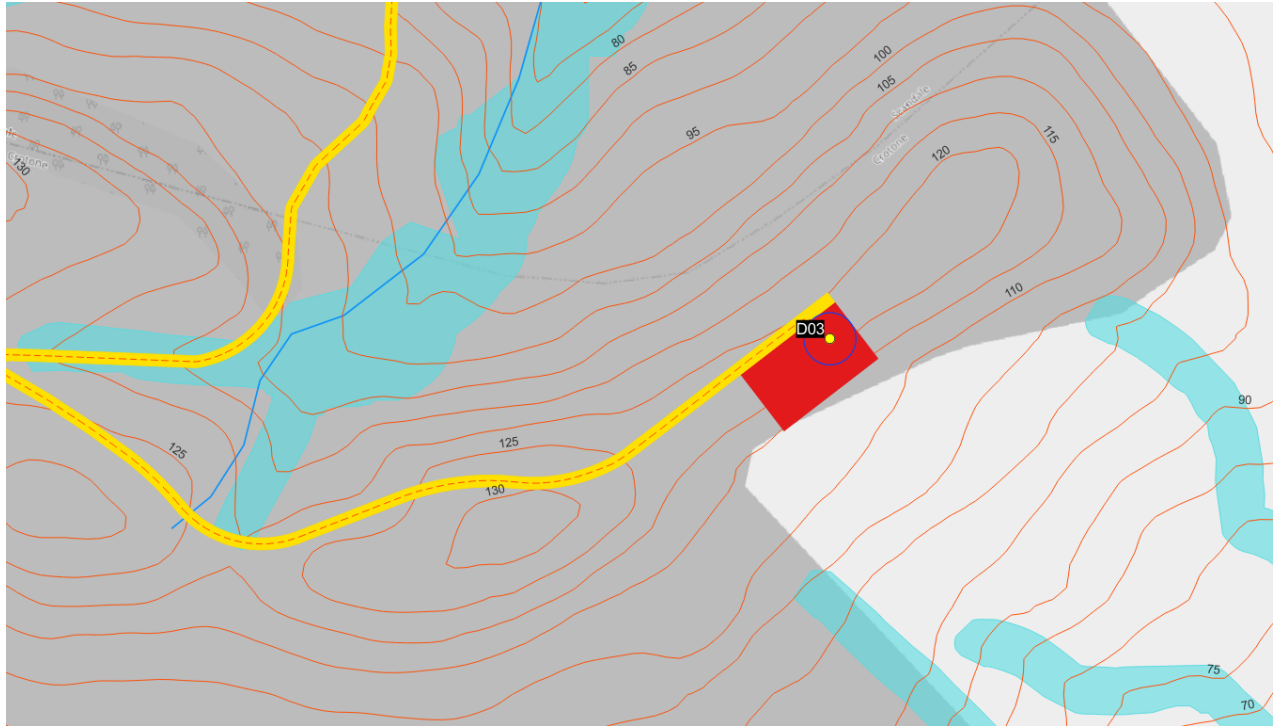
Figura 6-6 – Inquadramento D03 rispetto ai corsi d'acqua e alle aree di attenzione del PGRA con curve di livello.
