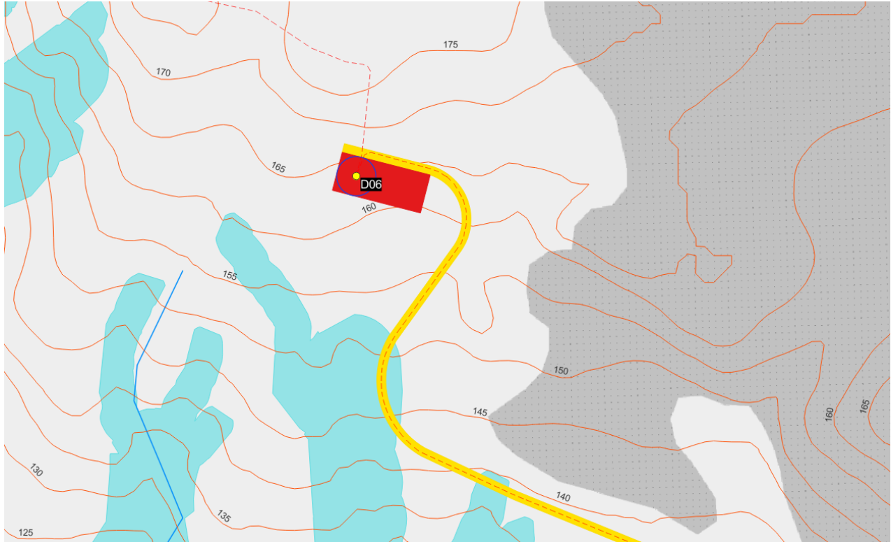
Figura 6-9 – Inquadramento D06 rispetto ai corsi d'acqua e alle aree di attenzione del PGRA con curve di livello.
