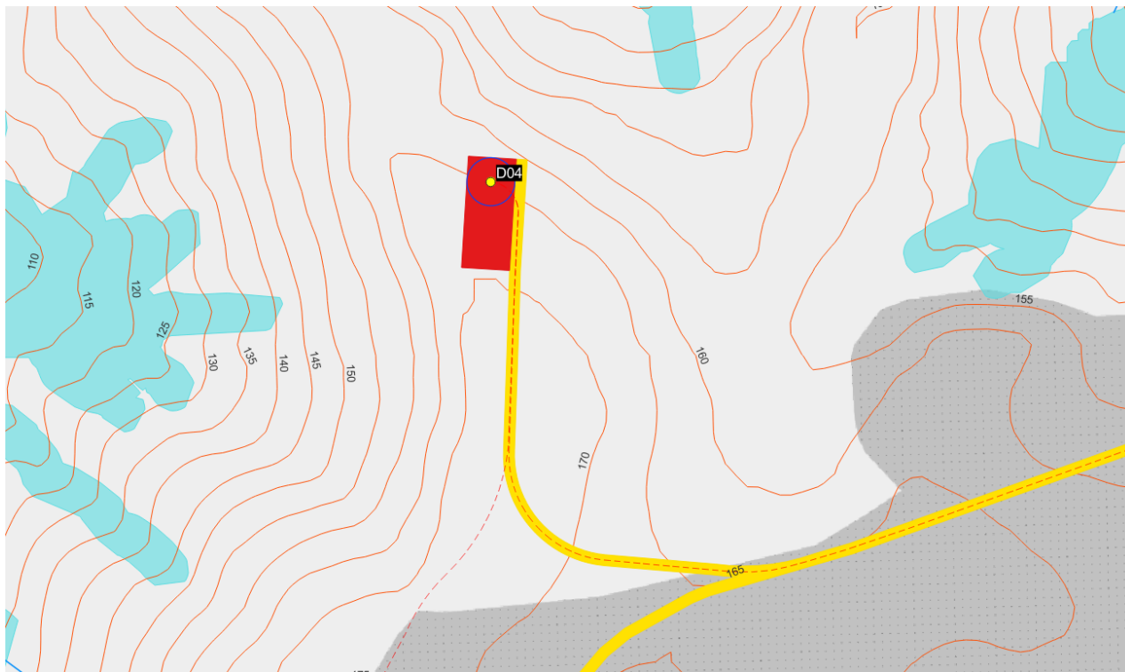
Figura 6-7 – Inquadramento D04 rispetto ai corsi d'acqua e alle aree di attenzione del PGRA con curve di livello.
