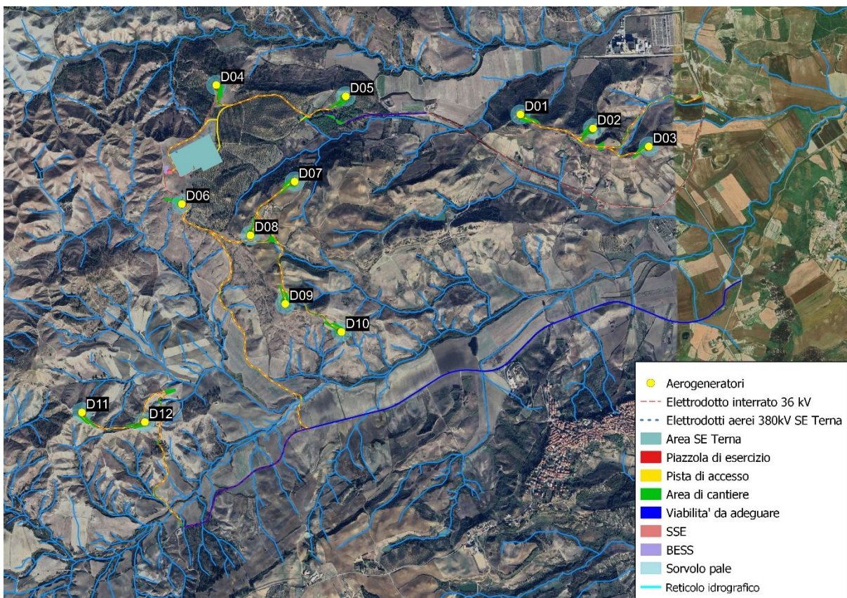
Figura 6-1 – Inquadramento delle opere in progetto rispetto al reticolo idrografico esistente
