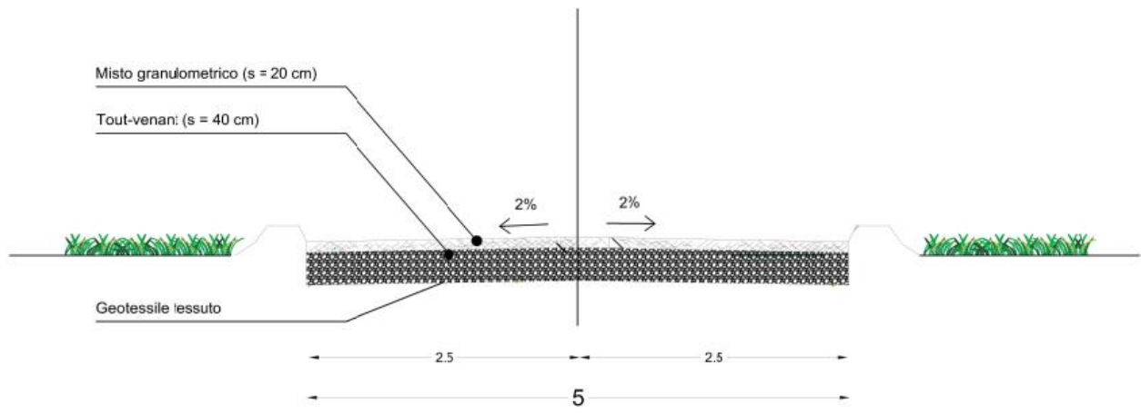
Figura - Sezione stradale tipo
