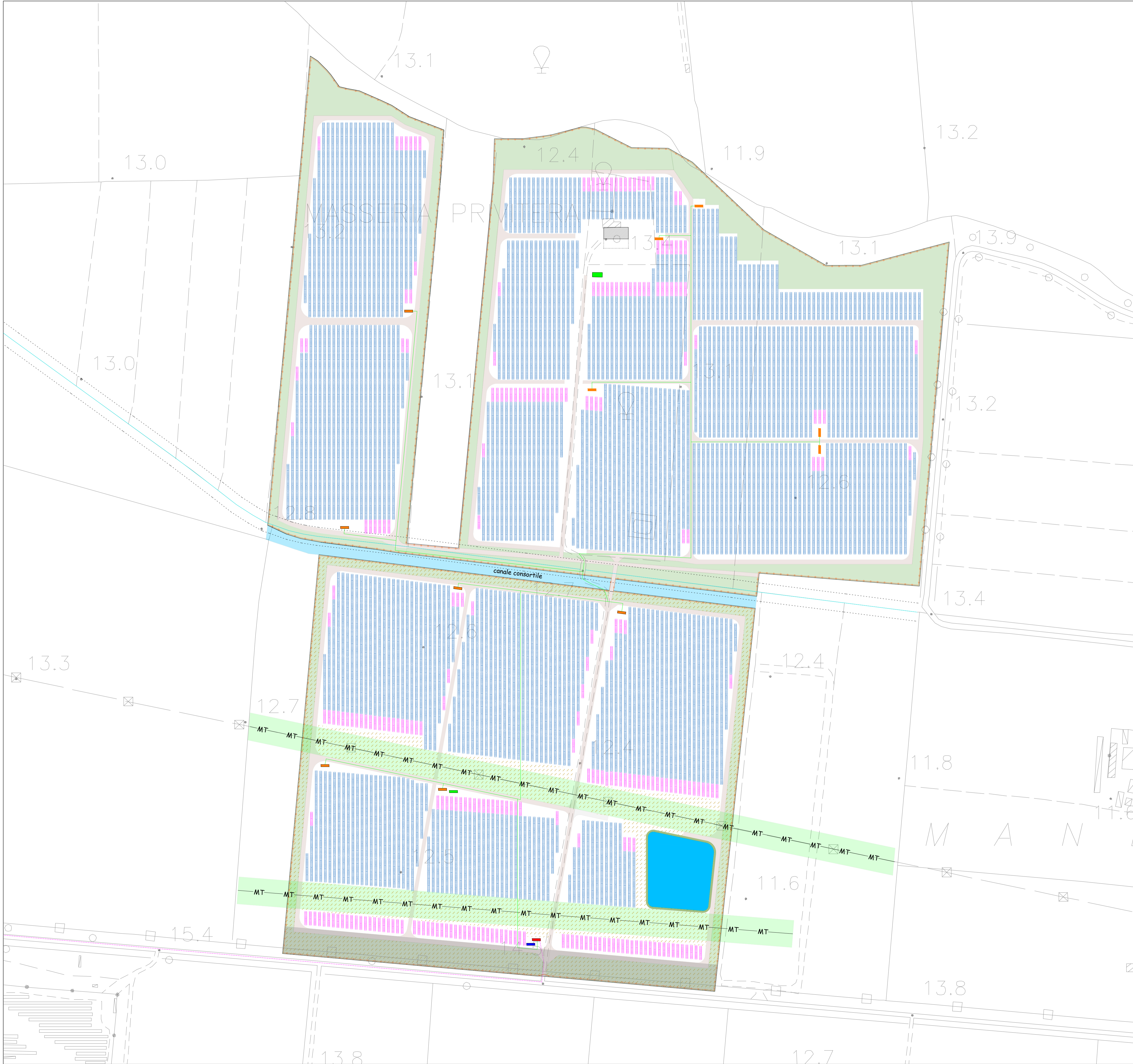
Elaborato : Layout impianto fotovoltaico su CTR (Campo 3)
