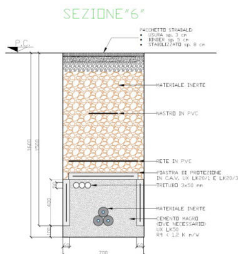
Figura 2.13 – Sezioni tipo posa cavidotti AT
