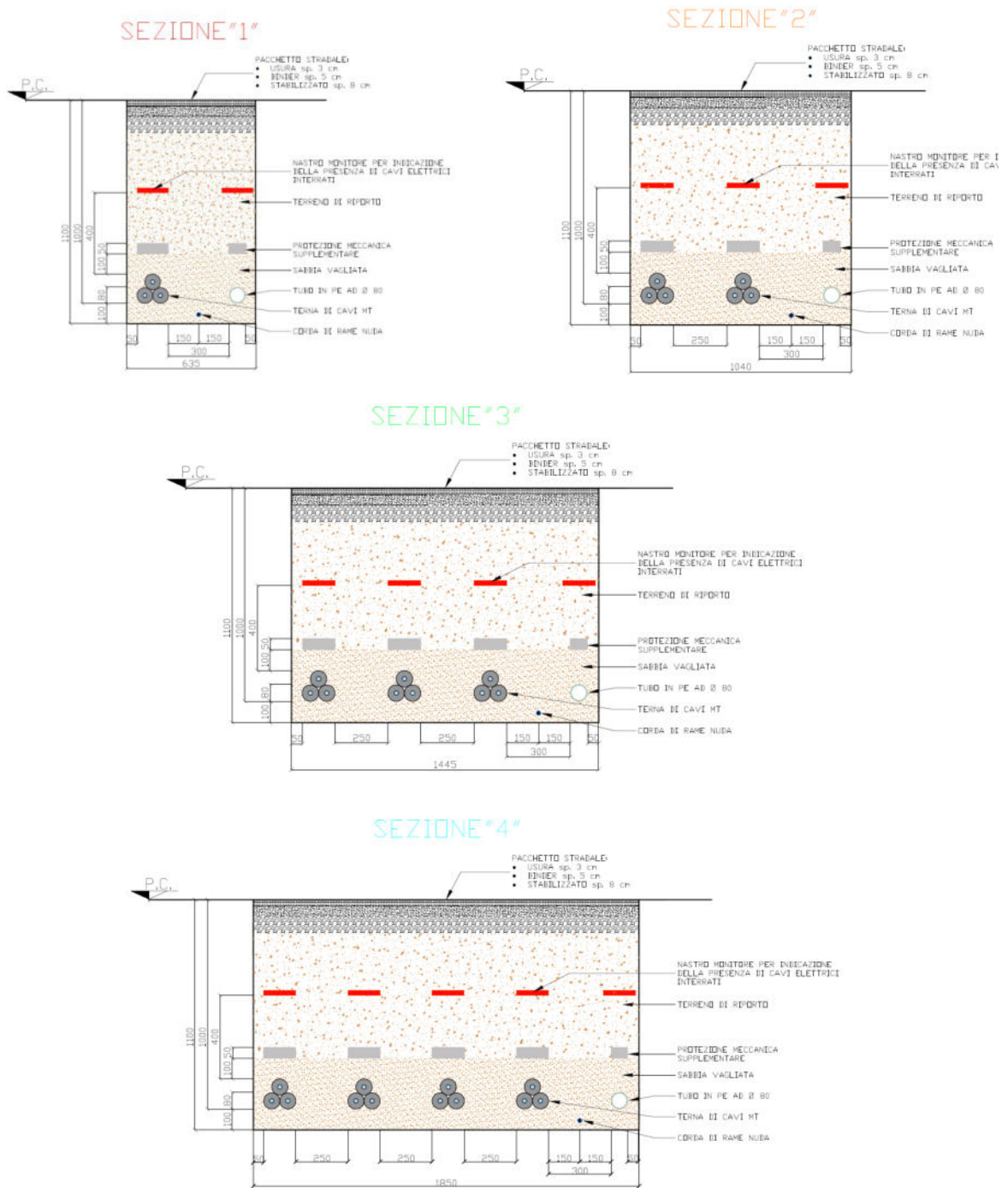
Figura 2.14 – Sezioni tipo posa cavidotti MT
