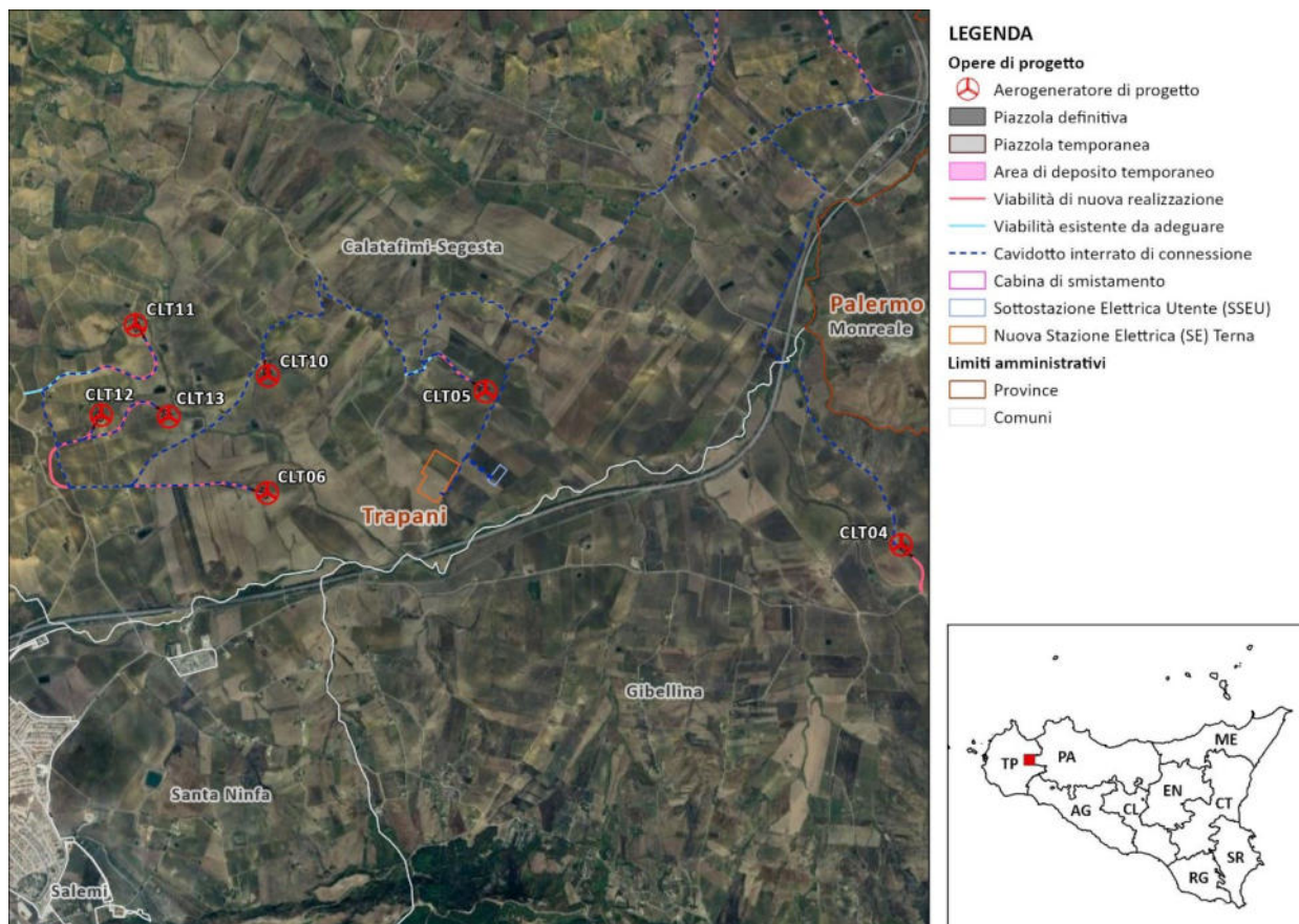
Figura 2.11: Inquadramento della viabilità di progetto nella parte sud del layout
