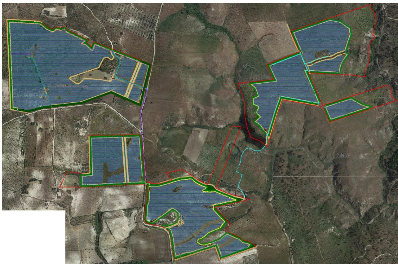
Figura 5 - Layout impianto
