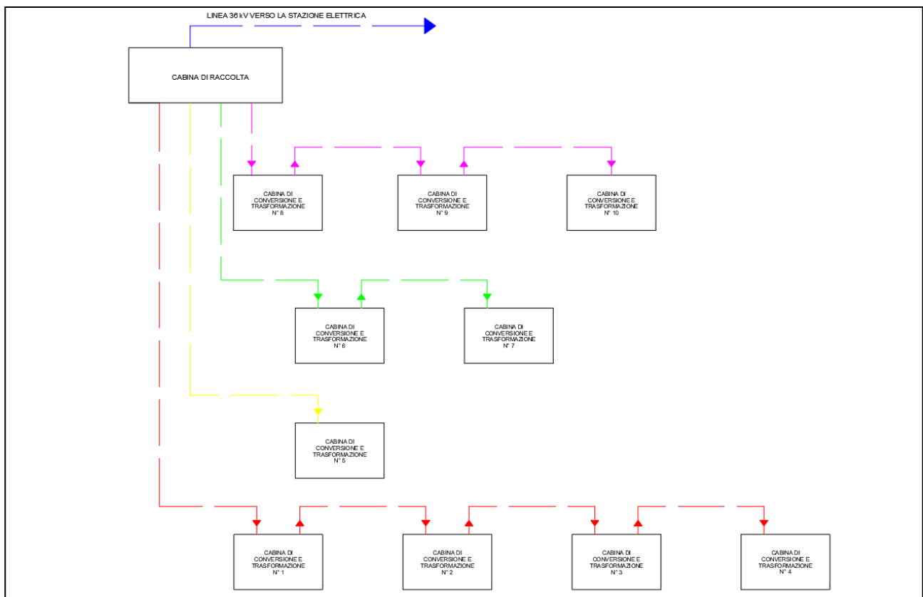
Figura 1- Schema a blocchi rappresentativo dell'impianto
