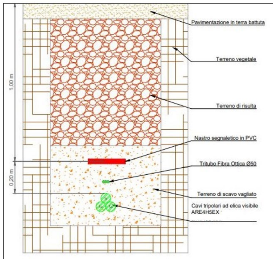
Figura 5 - Particolare di posa comprendente anche il tritubo in fibra ottica
