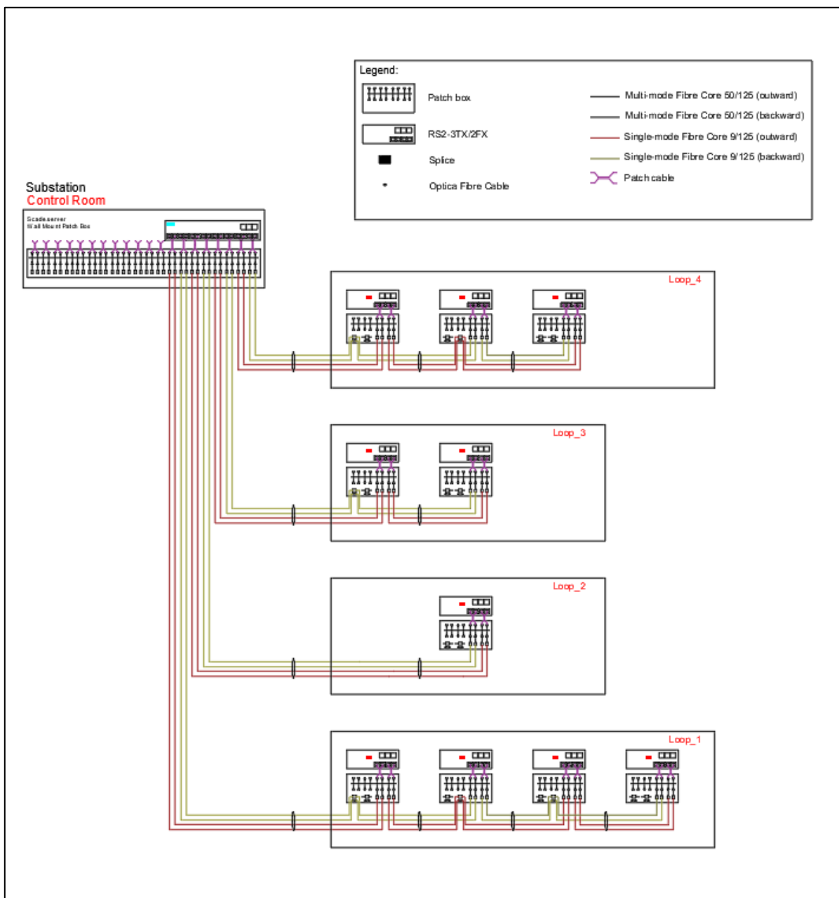
Figura 2 - Schema di impianto con loop di interconnessione
