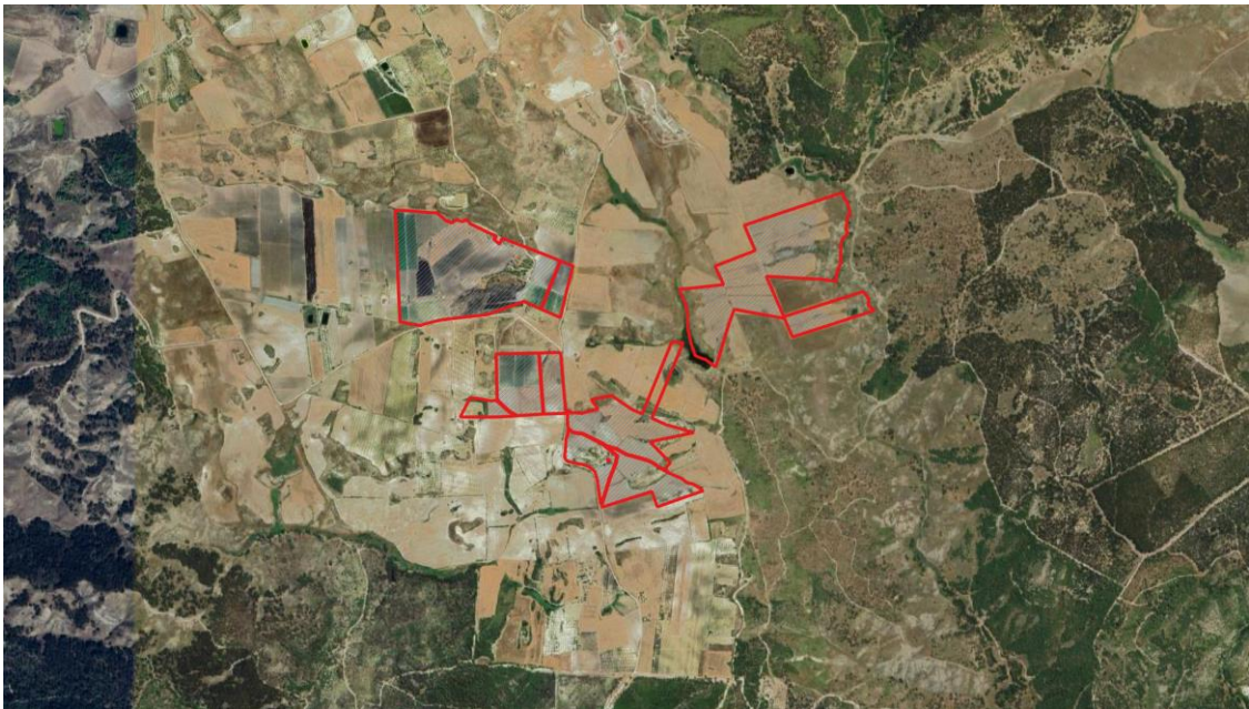
Figura 1 - Layout dell'impianto agrivoltaico su ortofoto.
