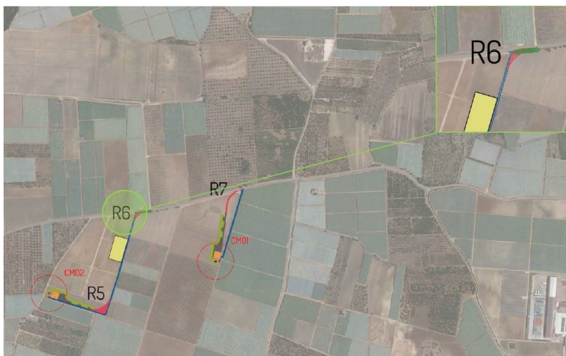
Figura 16: tratto di strada che sarà soggetto ad adeguamento per il passaggio di mezzi speciali
