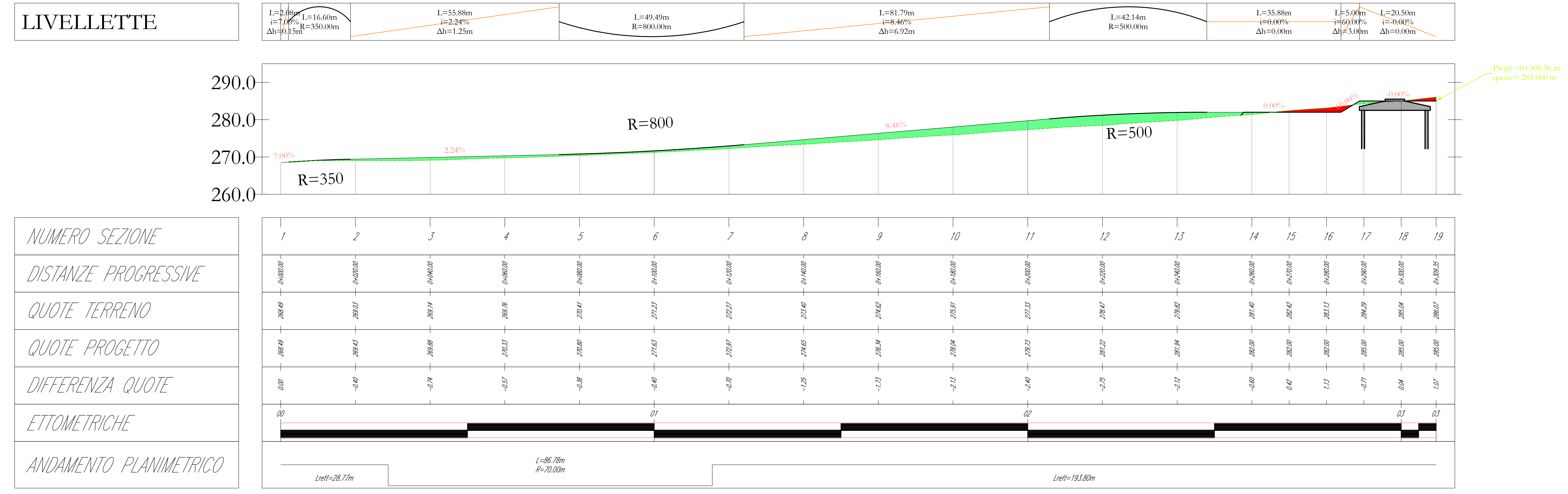
Profilo: Profilo longitudinale CG05 Q.Rif. : 260.00
