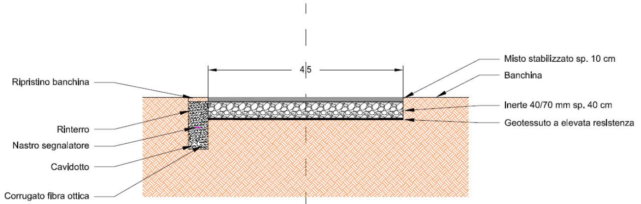
Figura 6 – Sezione tipo strade e piazzole
