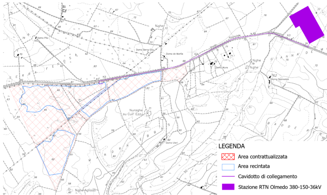
Figura 2 – Inquadramento dell'impianto FV e relative opere di connessione su ortofoto
