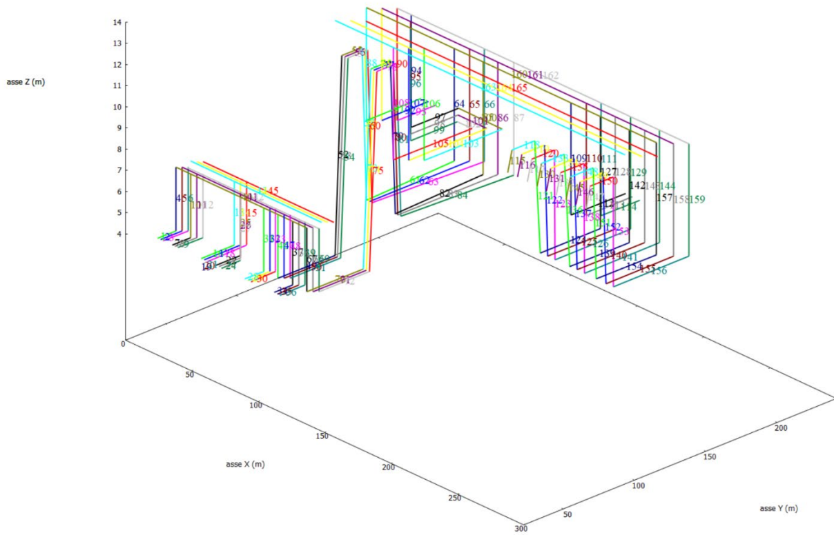
Figura 5 – Schematizzazione degli elementi attivi all'interno del programma di calcolo
