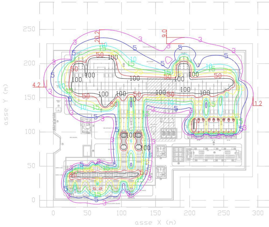
Figura 8 – Livelli di campo magnetico a 10 m dal piano della stazione
