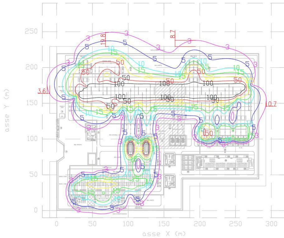
Figura 9 – Livelli di campo magnetico a 15 m dal piano della stazione
