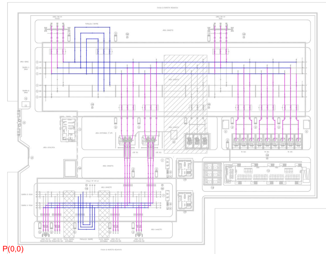
Figura 4 – Schematizzazione degli elementi attivi all'interno della planimetria
