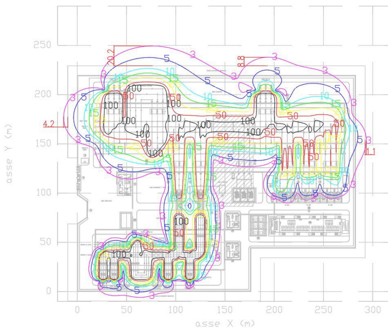
Curve isolivello del campo di Induzione Magnetica B - 5 metri
